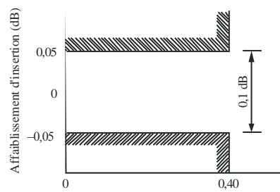
B) Tolérance d'ondulation dans la bande passante
