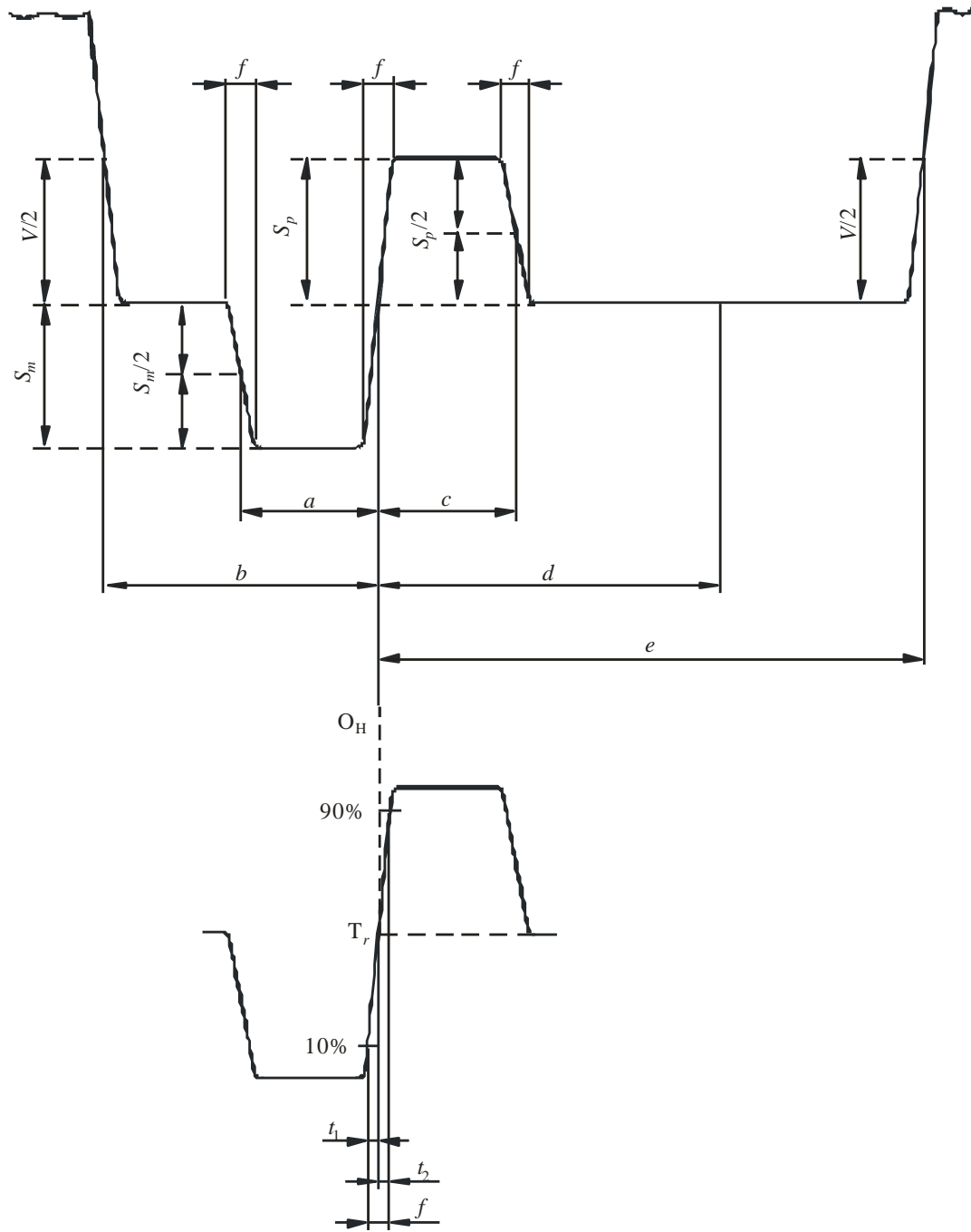
FIGURE 4 Forme d'onde du signal de synchronisation de ligne
