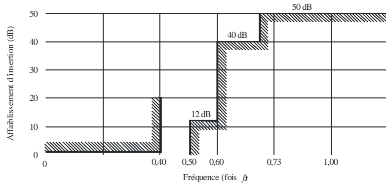
A) Gabarit pour l'affaiblissement d'insertion
