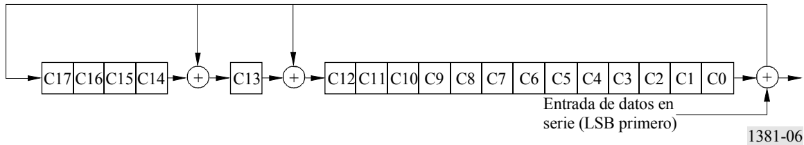
FIGURA 6 Polinomio generador
