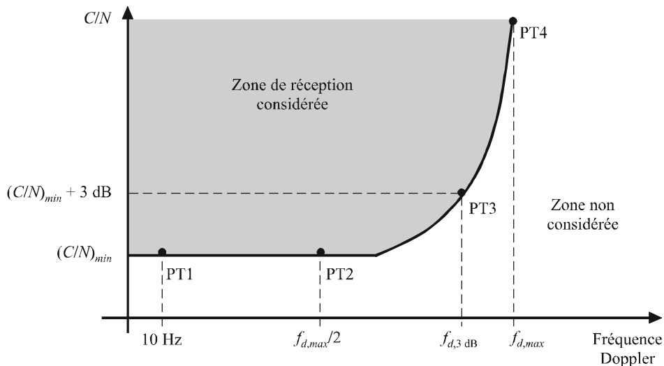
Valeurs du rapport moyen C/N requises dans un canal de propagation utilisé pour la réception mobile
