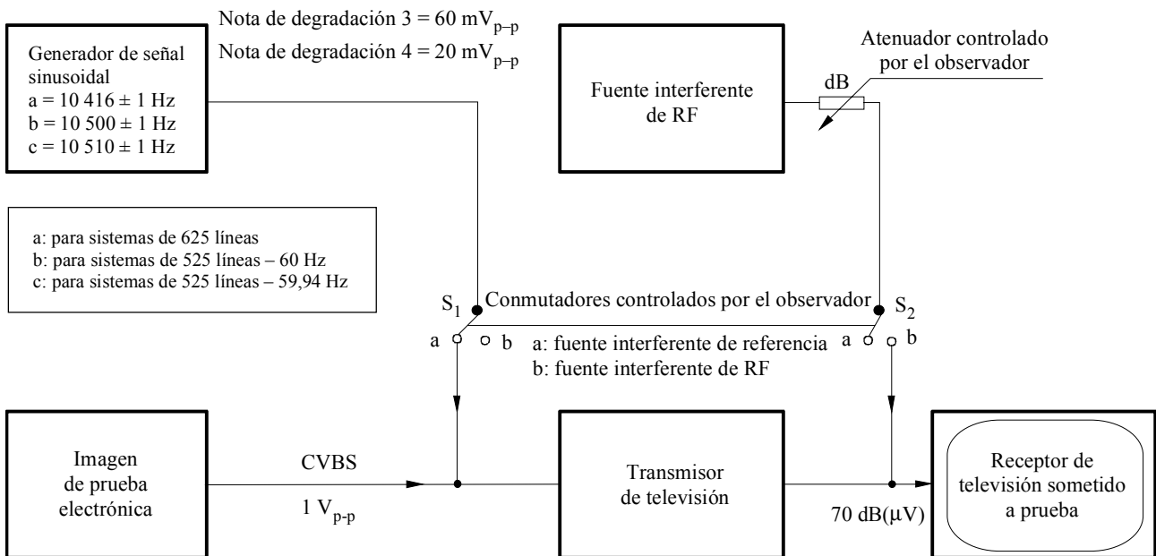
FIGURA 2 Método de comparación subjetiva para la evaluación de las relaciones de protección
