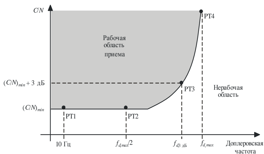
РИСУНОК 3 Необходимое среднее значение C/N в канале распространения подвижной связи
