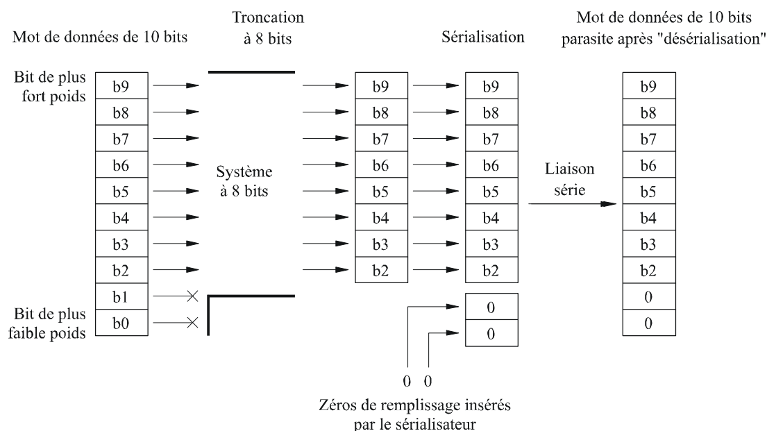
FIGURE 2 Altération d'un mot de données
