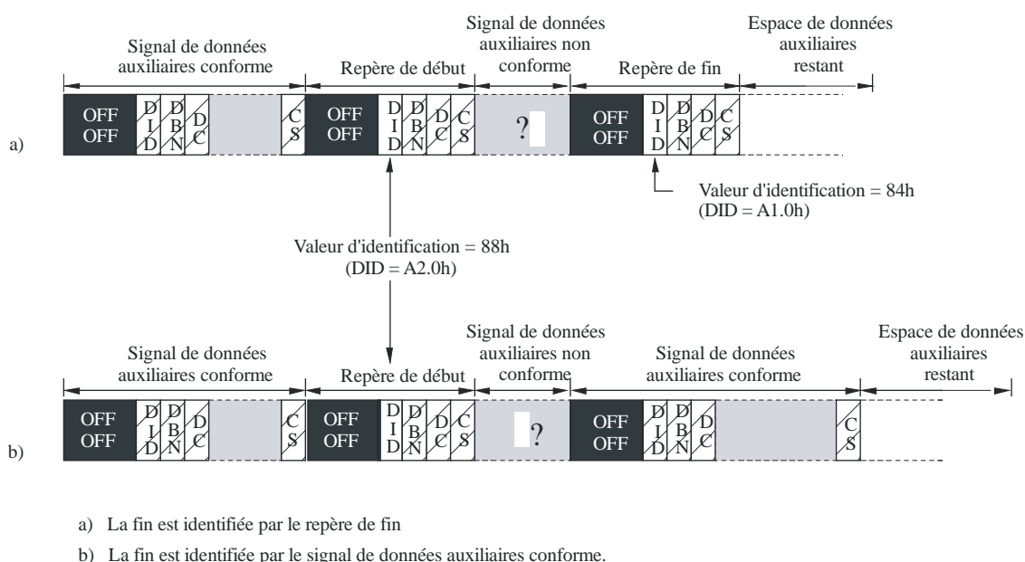
FIGURE 4 Insertion de paquets de données auxiliaires non conformes
