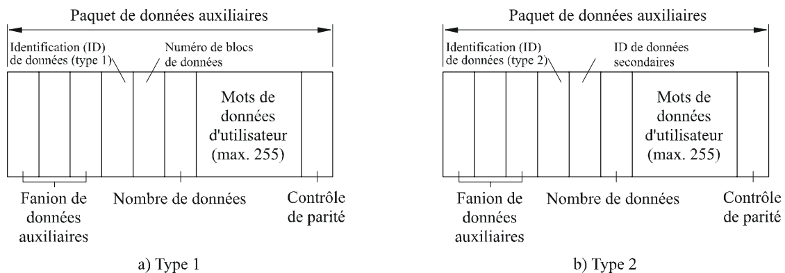
FIGURE 1 Types de paquets de données auxiliaires
