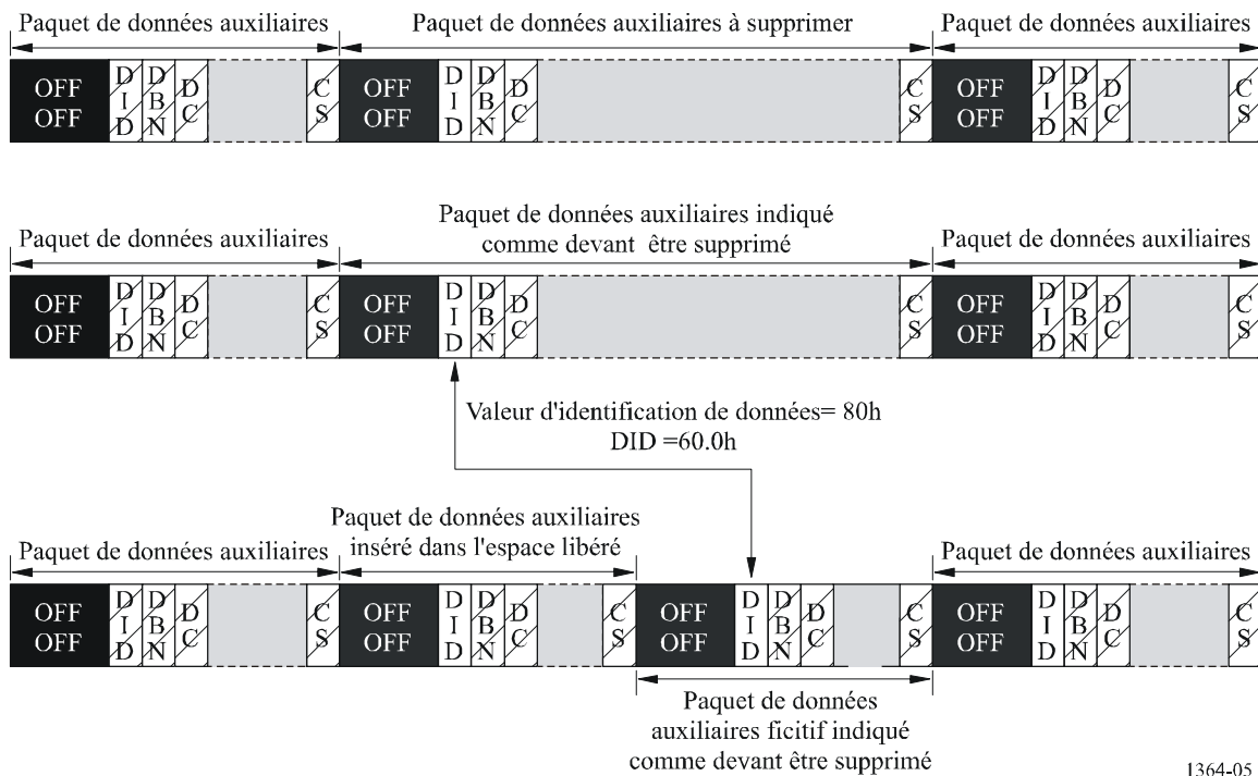
FIGURE 5 Suppression d'un paquet de données auxiliaires et réutilisation de l'espace de données auxiliaires
