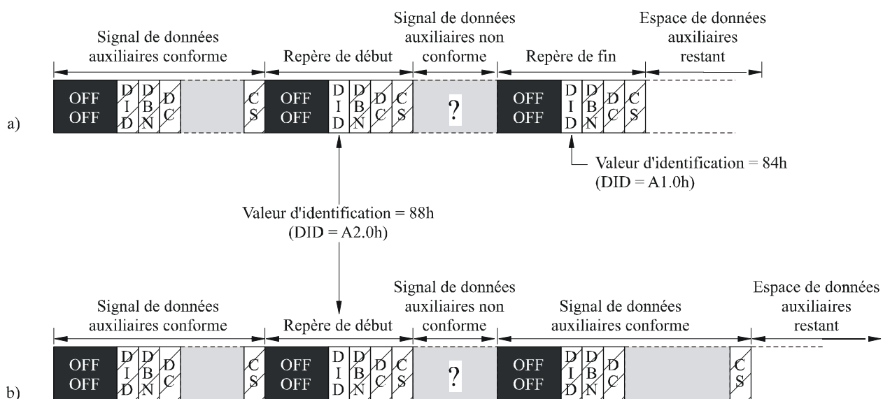
FIGURE 4 Insertion de paquets de données auxiliaires non conformes
