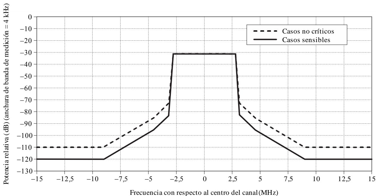
Plantillas de los límites del espectro específicas para el sistema D de canalización de 6 MHz (DTMB)
