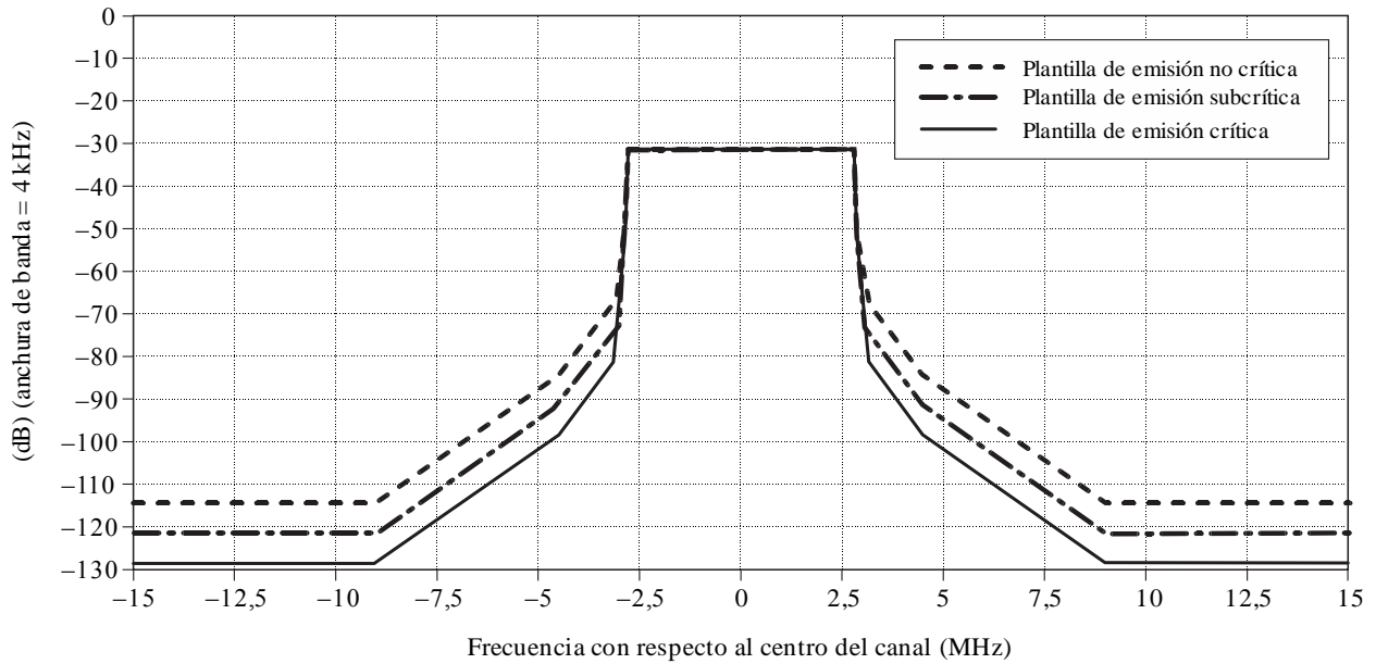
Plantillas de límite del espectro para el sistema C de canalización de 6 MHz (ISDB-T)
