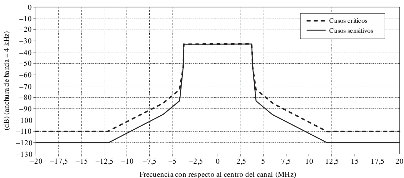
Plantillas de límite del espectro para el sistema C de canalización de 8 MHz (ISDB-T)
