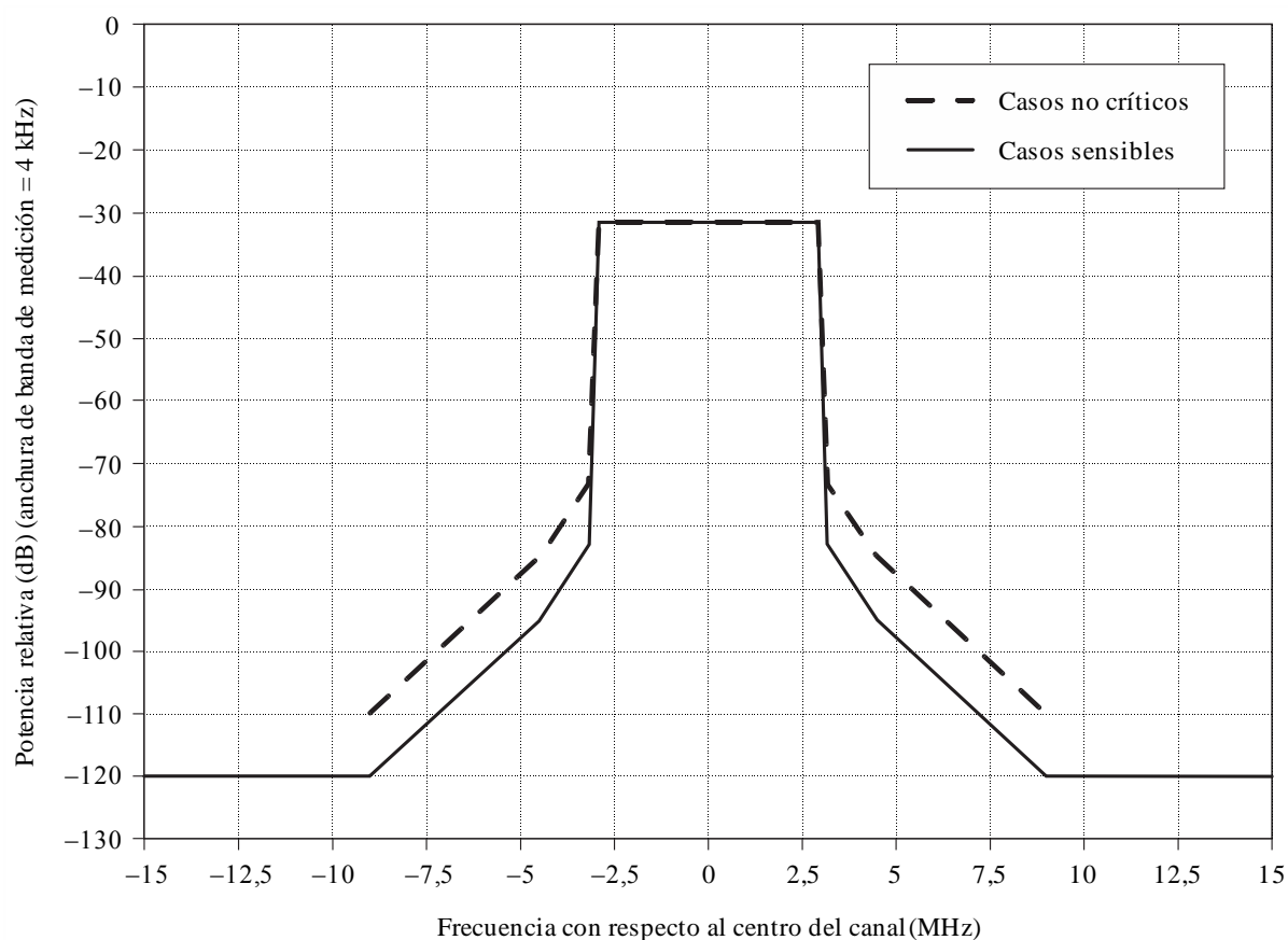
Plantillas de límite del espectro para el sistema B de canalización de 6 MHz (DVB-T)
