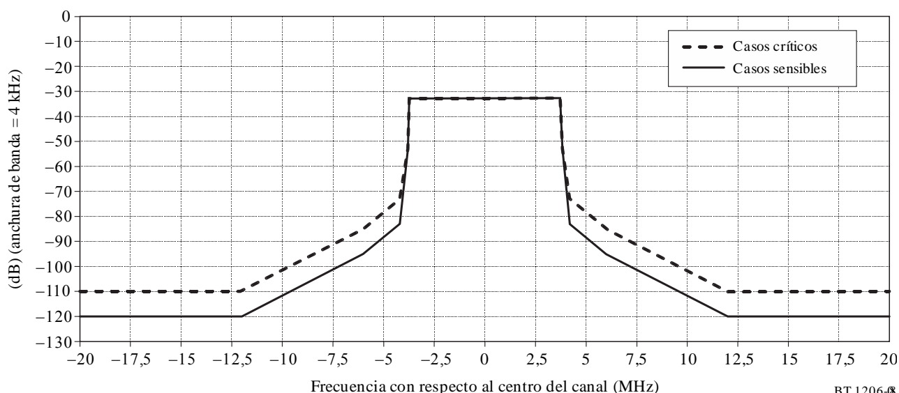
Plantillas de límite del espectro para el sistema C de canalización de 7 MHz (ISDB-T)
