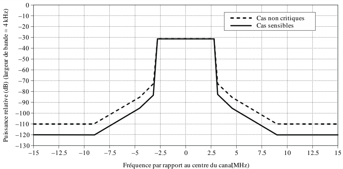
Gabarits de limite spectrale propres au système D (DTMB) utilisant un découpage en canaux de 6 MHz
