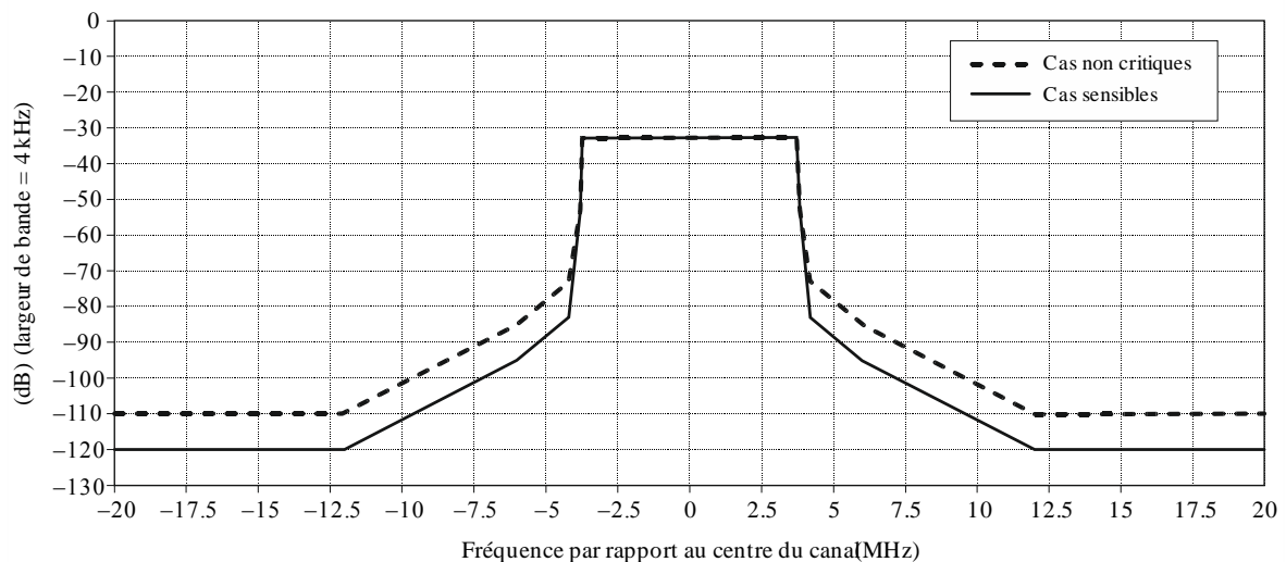
Gabarits de limite spectrale propres au système C (ISDB-T) utilisant un découpage en canaux de 7 MHz
