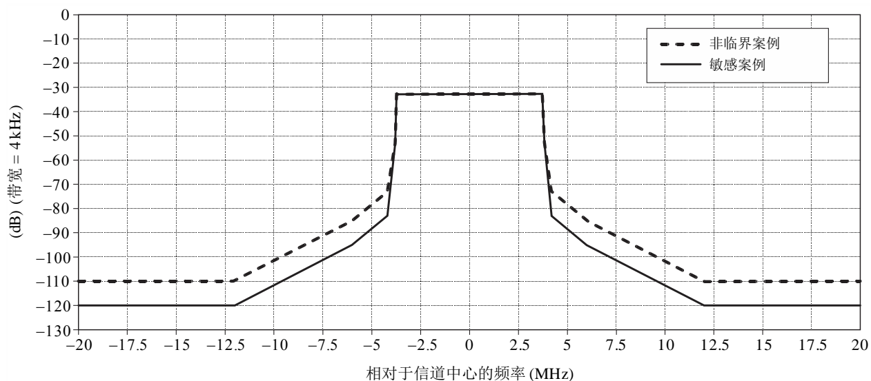
用于8 MHz信道配置系统C (ISDB-T) 的频谱限制掩模
