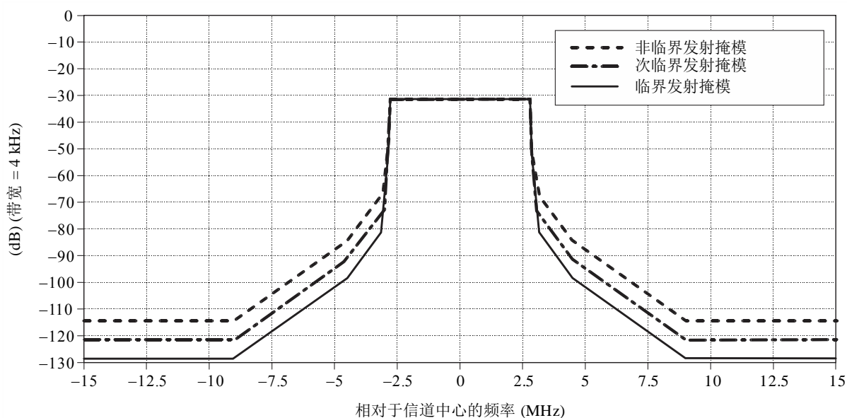
用于6 MHz信道配置系统C (ISDB-T) 的频谱限制掩模
