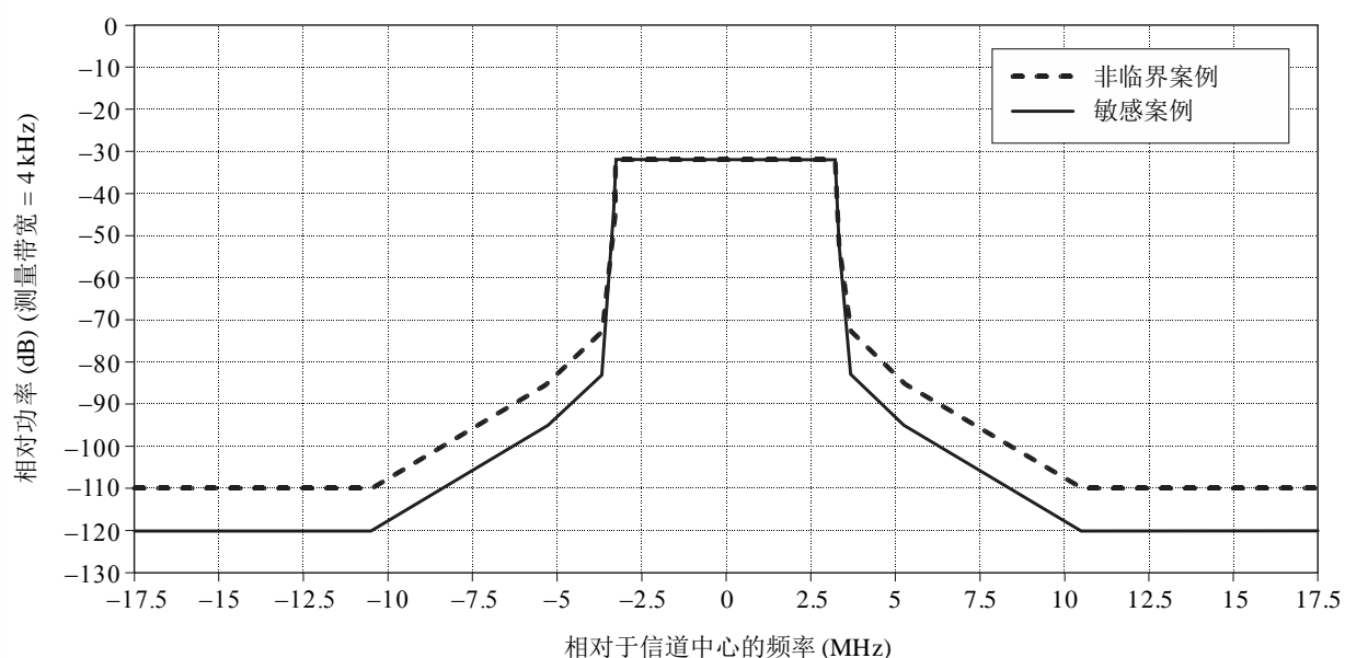
用于7 MHz信道配置系统D (DTMB) 的频谱限制掩模
