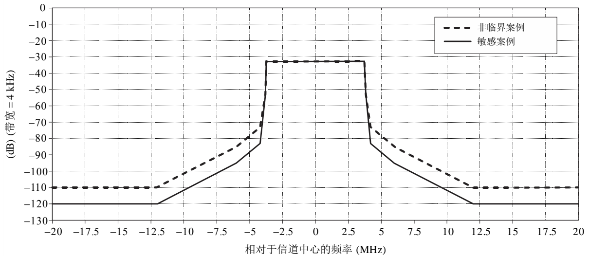
用于7 MHz信道配置系统C (ISDB-T) 的频谱限制掩模
