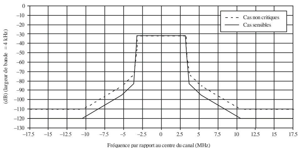
Gabarits de limite spectrale propres au système C (ISDB-T) utilisant un découpage en canaux de 7 MHz
