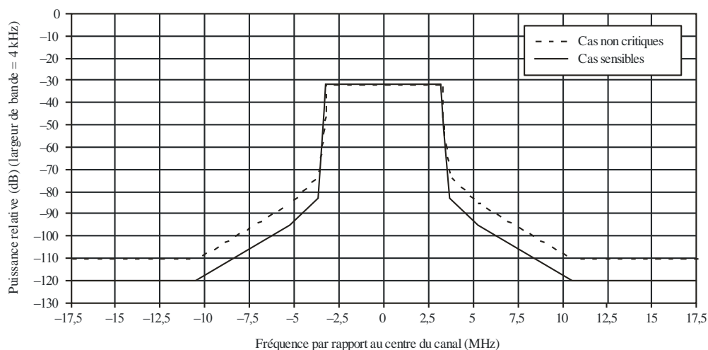
Gabarits de limite spectrale propres au système D (DTMB) utilisant un découpage en canaux de 7 MHz
