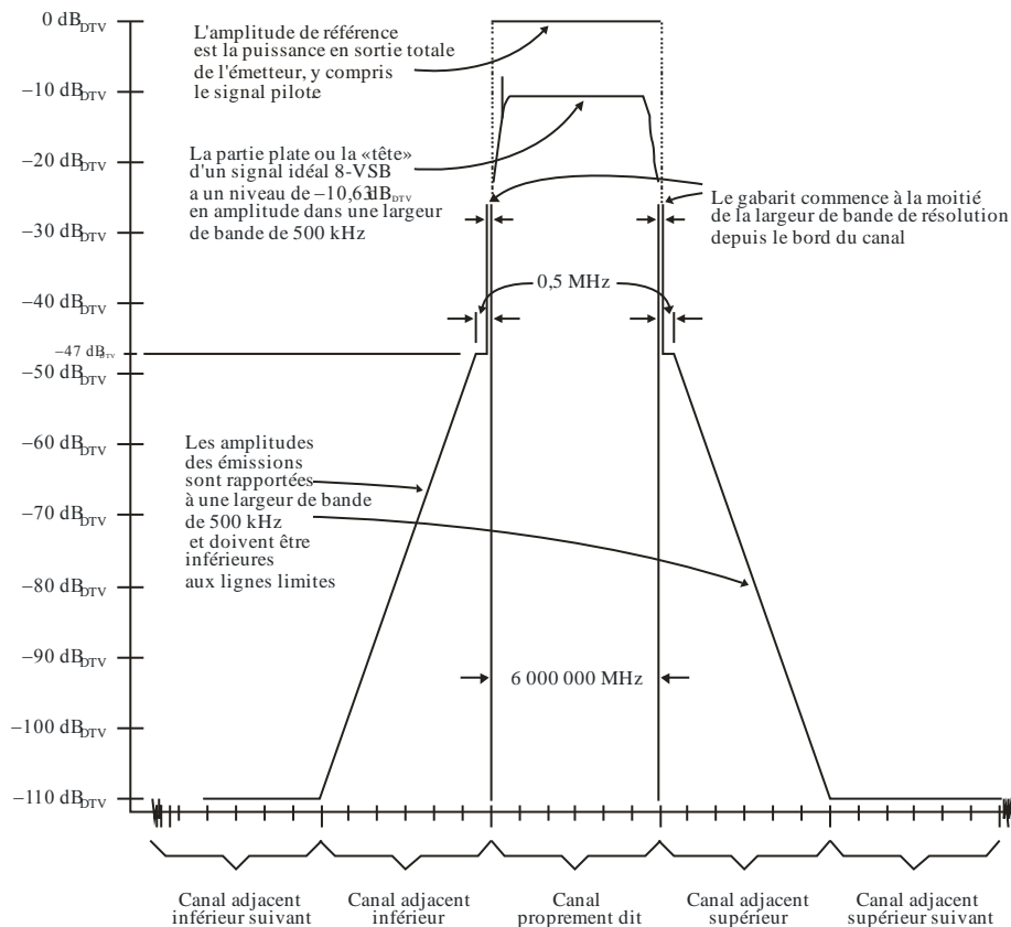
FIGURE 1 Gabarit de limite spectrale pour des systèmes de télévision numérique de Terre utilisant des canaux de 6 MHz et une modulation 8-VSB
