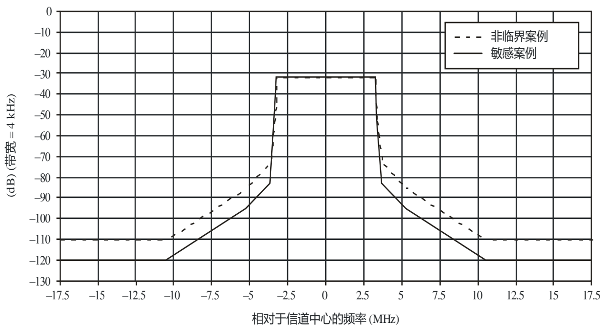
用于7 MHz信道配置系统C (ISDB-T) 的频谱限制掩模
