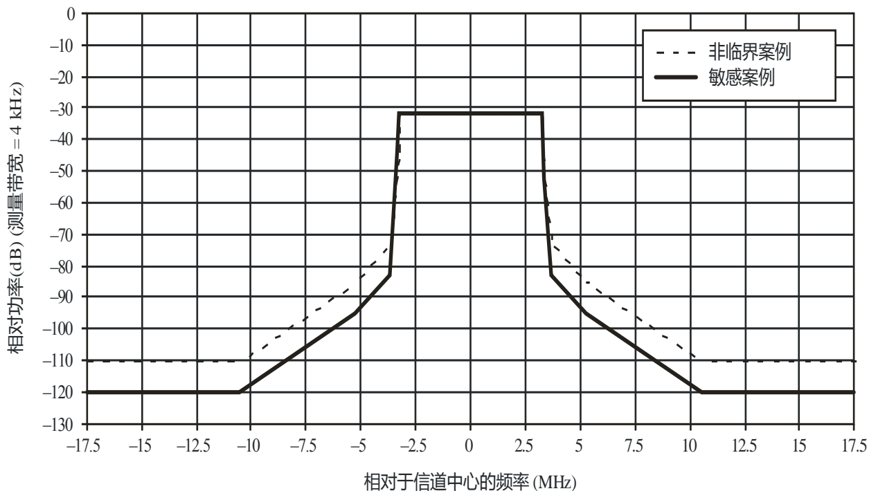
用于7 MHz信道配置系统D (DTMB) 的频谱限制掩模
