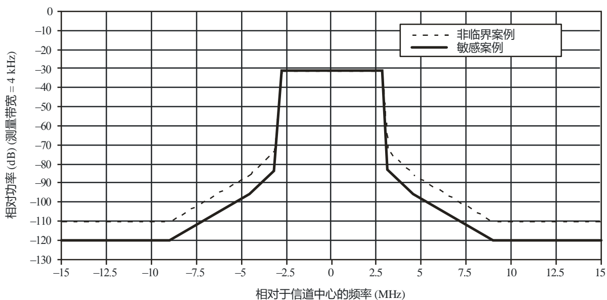
用于6 MHz信道配置系统D (DTMB) 的频谱限制掩模
