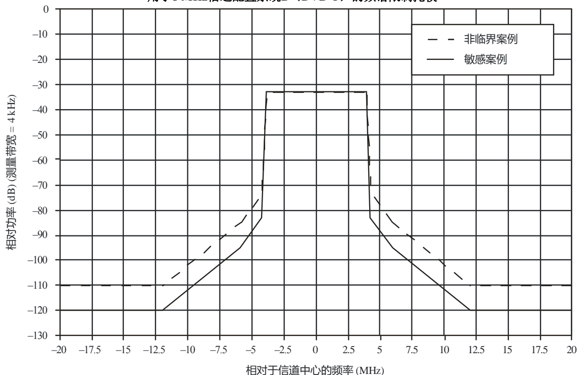
用于8 MHz信道配置系统B (DVB-T) 的频谱限制掩模
