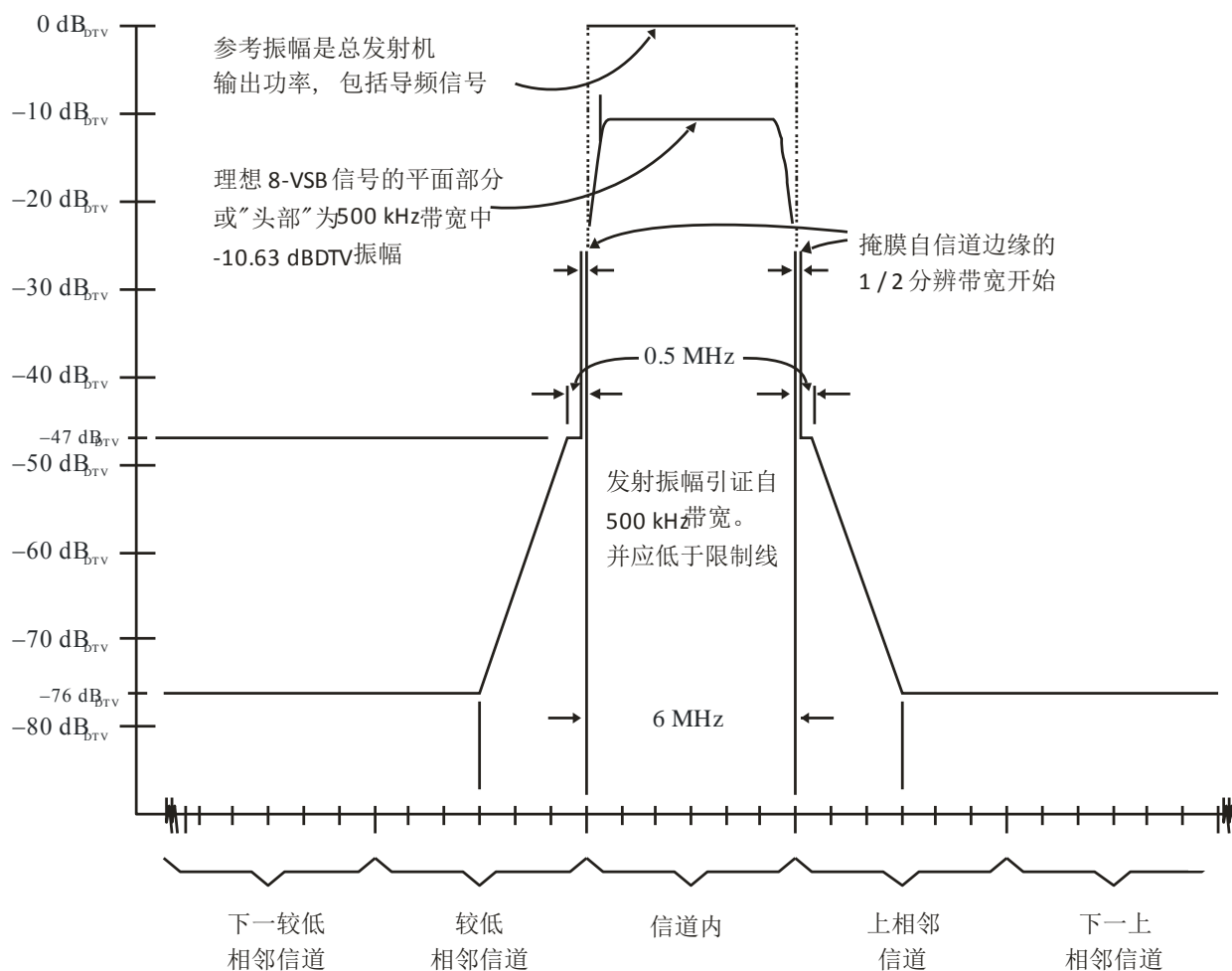
6 MHz高功率8-VSB LPTV发射机和转换器
