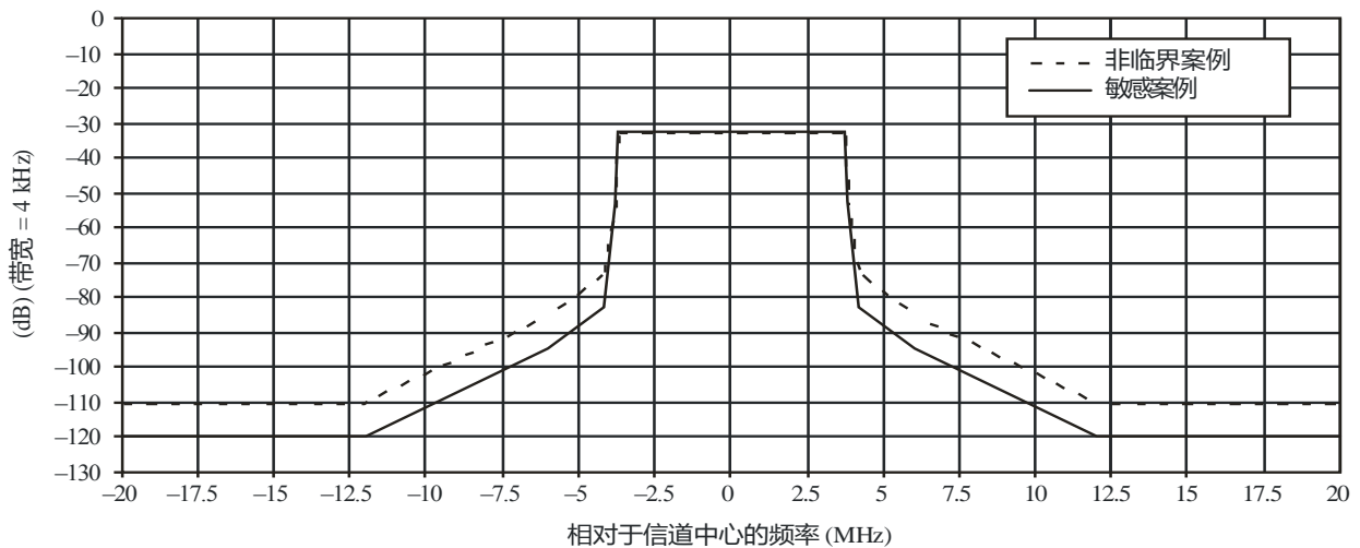
用于8 MHz信道配置系统C (ISDB-T) 的频谱限制掩模
