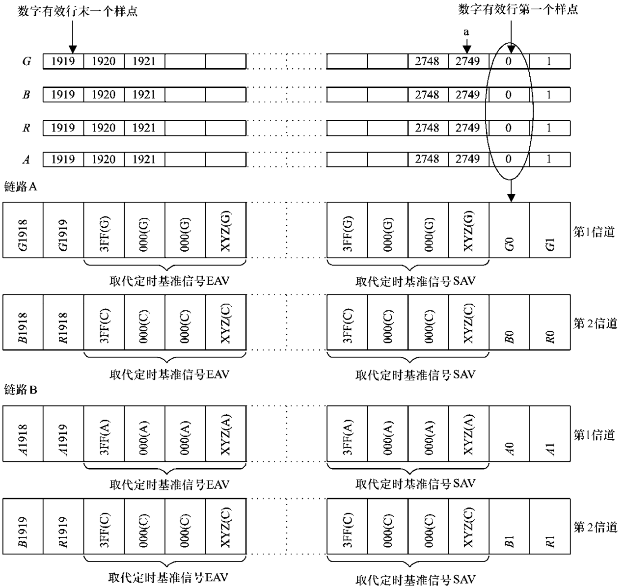
4:4:4 (R'G'B') 和4:4:4 (R'G'B'+A) 10比特信号的复用结构
