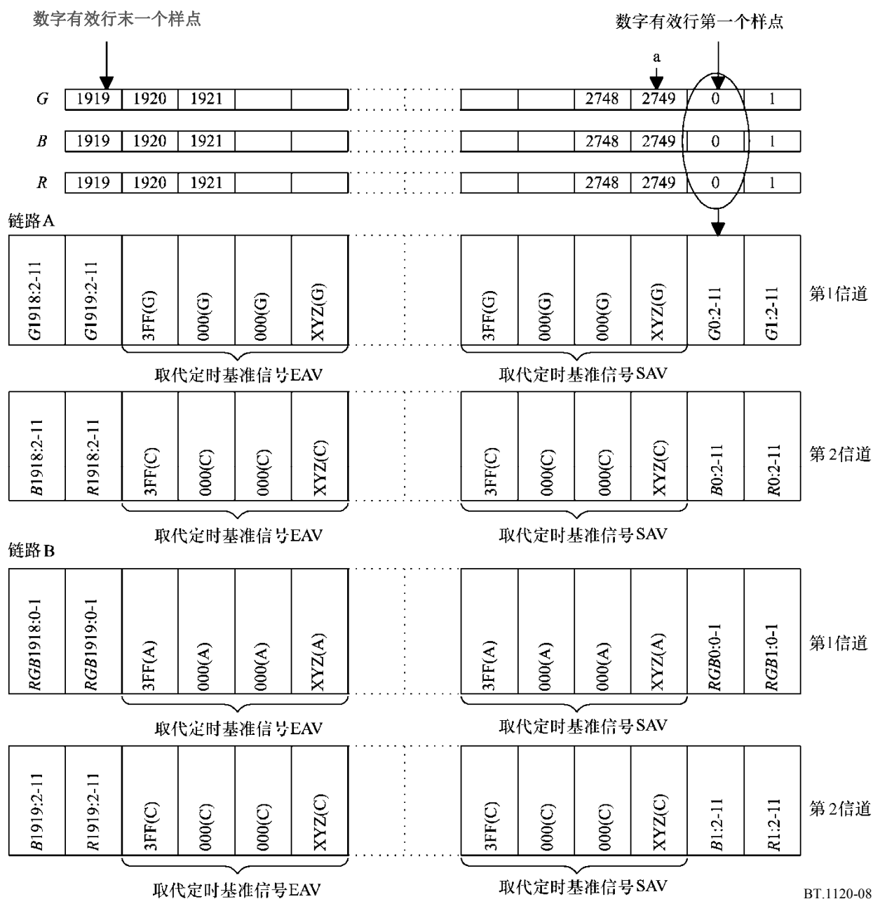
4:4:4 (R'G'B) 12比特信号的复用结构
