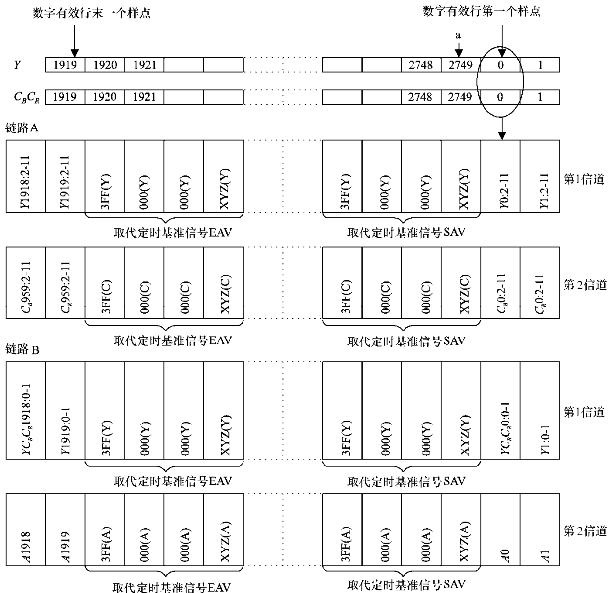
图10 4:2:2 (YCbBR) 12比特信号的复用结构
