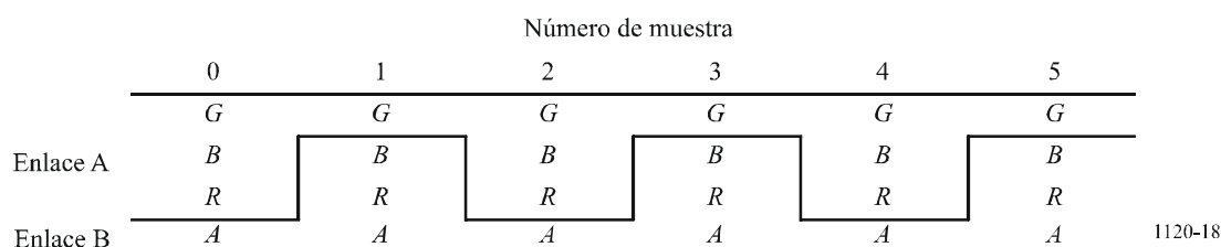
FIGURA 18 Contenido del enlace para señales 4:4:4 (RGB) y 4:4:4 (RGB + A) de 10 bits
