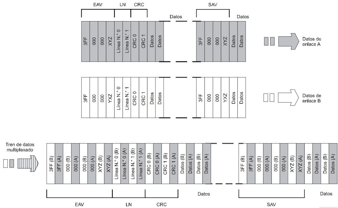
FIGURA 27 Multiplexación de enlace doble enlace único
