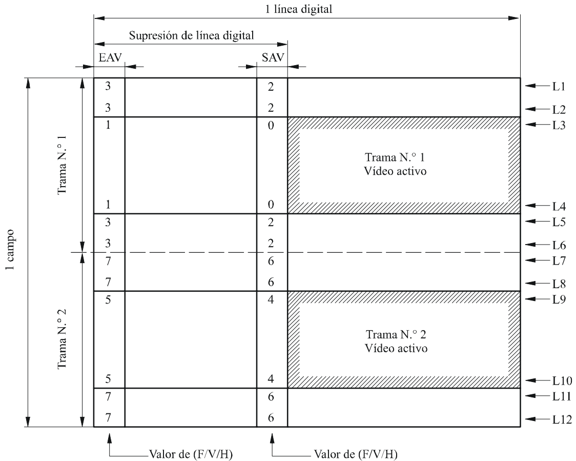
FIGURA 1 Relaciones de la temporización de trama
