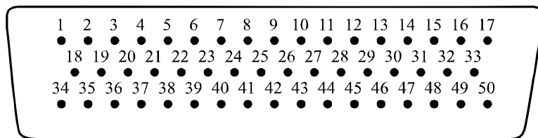
Cara de conexión para el receptáculo conector que contiene las patillas (conector macho) en el sistema 1250/50/2:1
