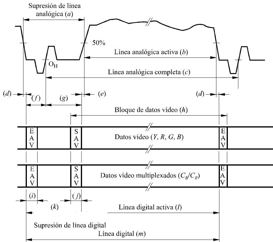
FIGURA 6 Formato de datos y relaciones de temporización con la onda analógica
