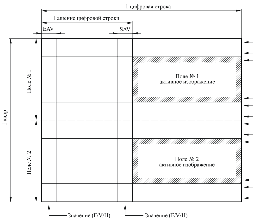
РИСУНОК 1 Соотношения параметров синхронизации поля
