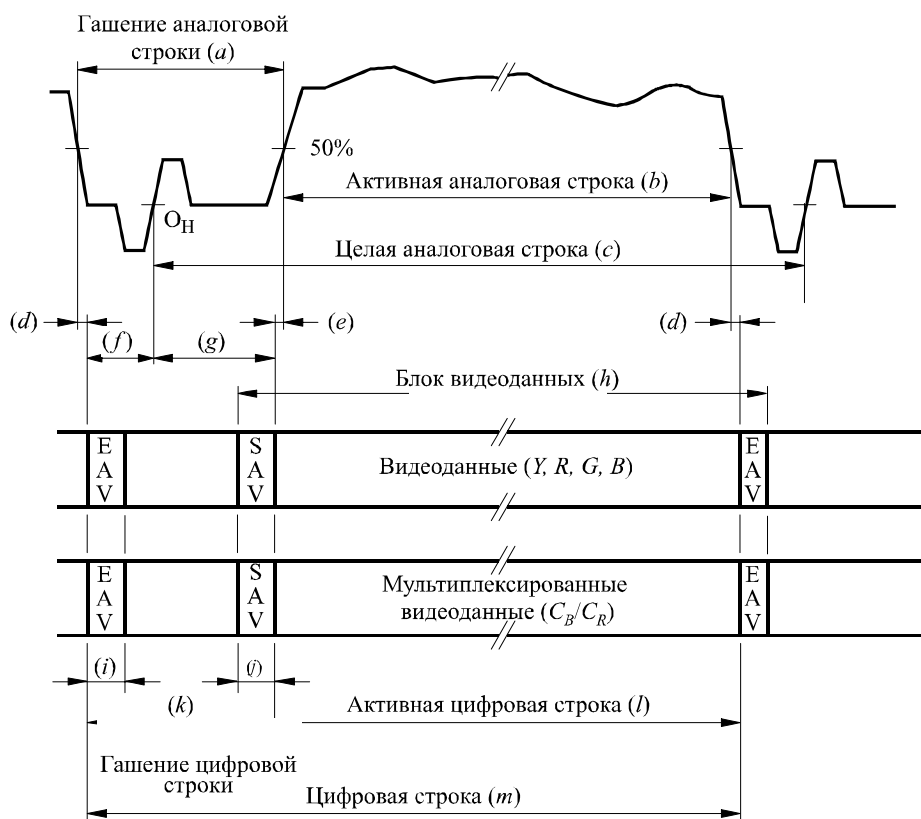
Формат данных и соответствие синхронизации видеосигнала аналоговому сигналу
