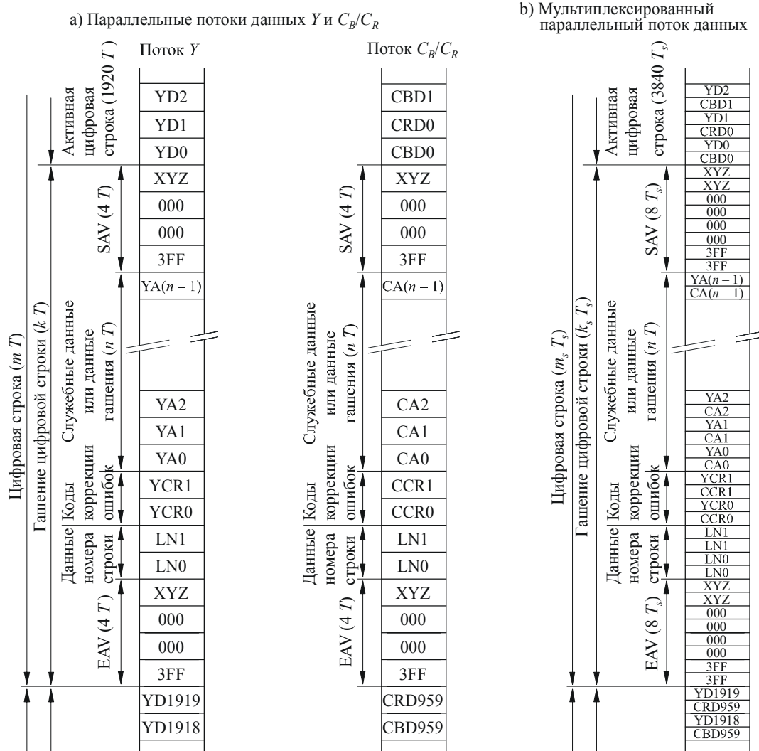
РИСУНОК 14 Поток данных
