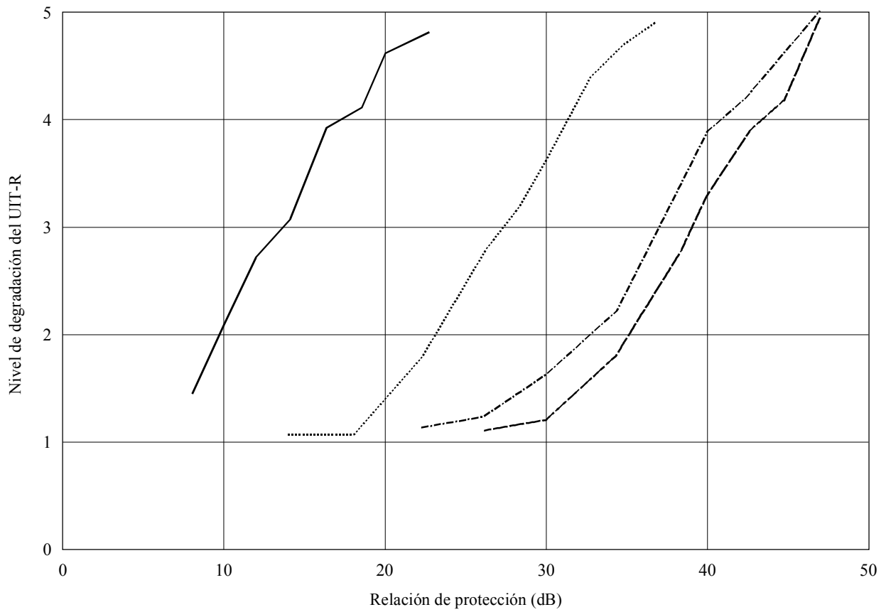
FIGURA 9 Relación de protección para estereofonía en isofrecuencia e isomodulación Modulación: Piano estereofónico
