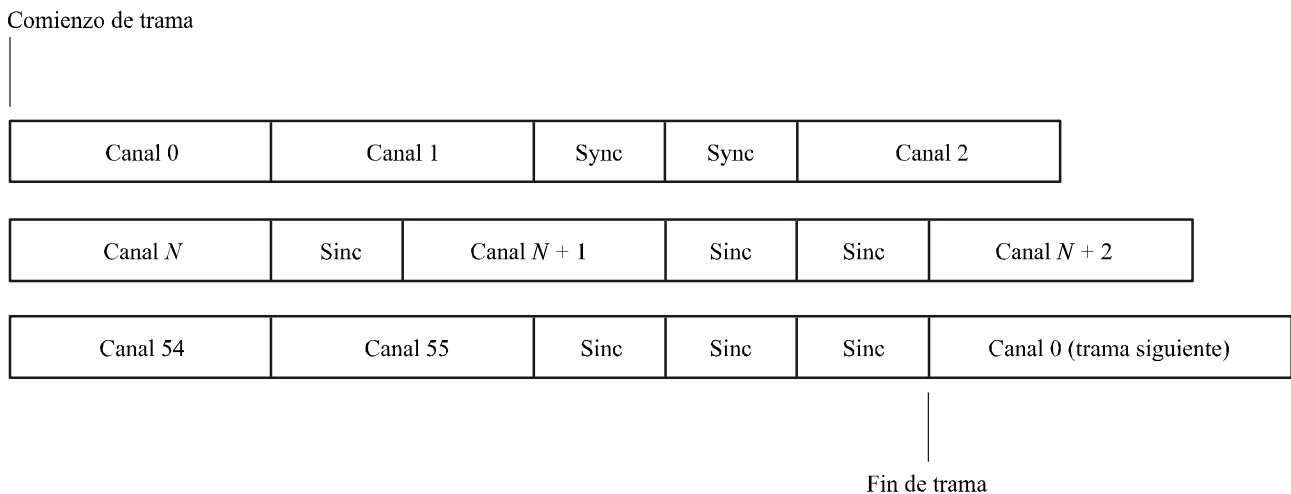
FIGURA 4 Posiciones permitidas de los símbolos de sincronización 4B5B
