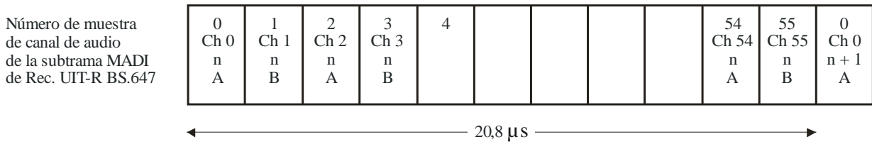
FIGURA 2 48 kHz con 56 canales activos
