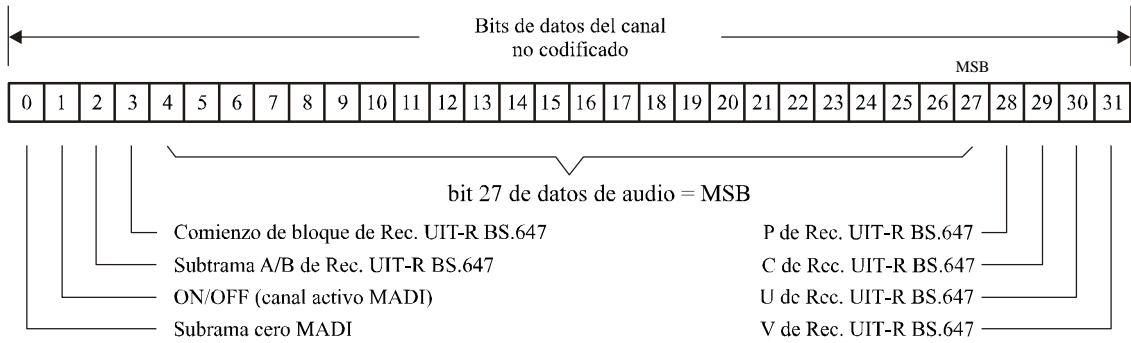
FIGURA 3 Formato de los datos de un canal
