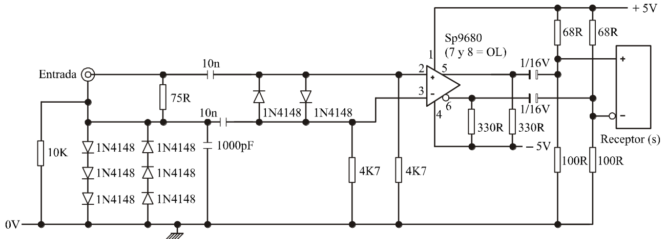
FIGURE 8 Circuito tampón de la MADI (informativo)
