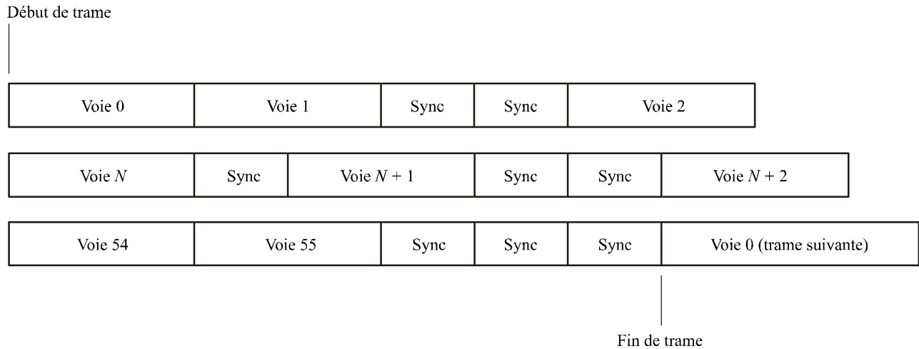
FIGURE 4 Quelques positions admissibles du symbole de synchronisation 4B5B
