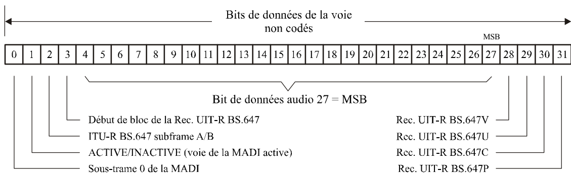
FIGURE 3 Structure des données de la voie
