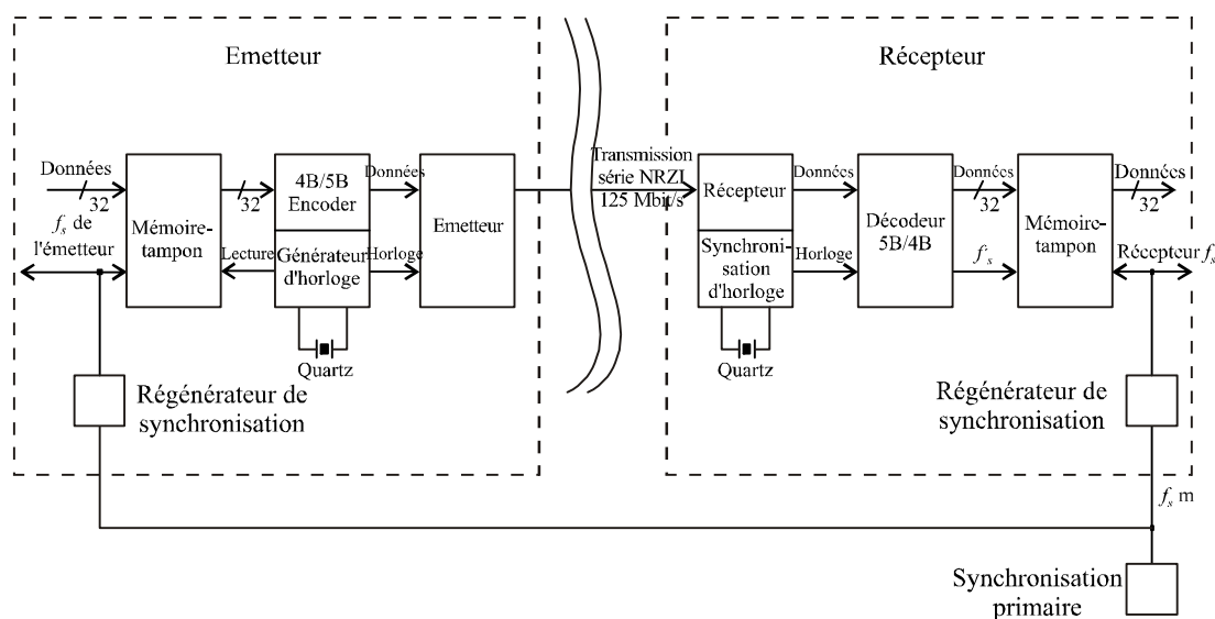
FIGURE 1 Diagramme de la MADI
