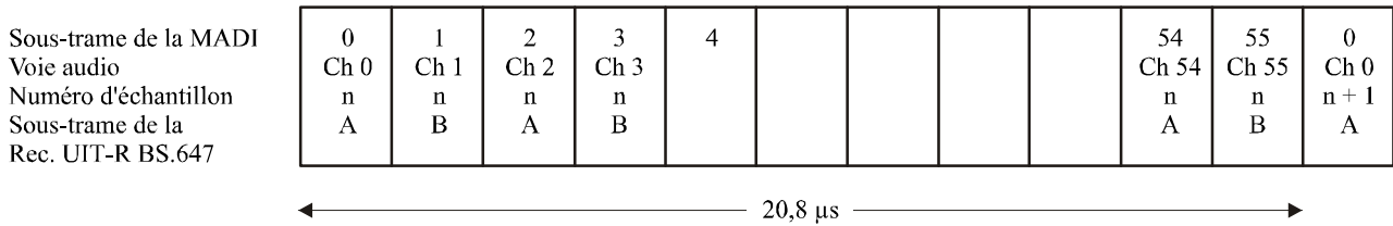
FIGURE 2 48 kHz avec 56 voies en service
