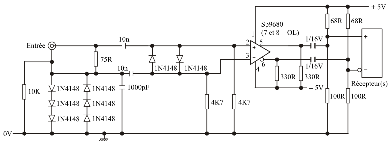
FIGURE 8 Circuits de la mémoire-tampon de la MADI
