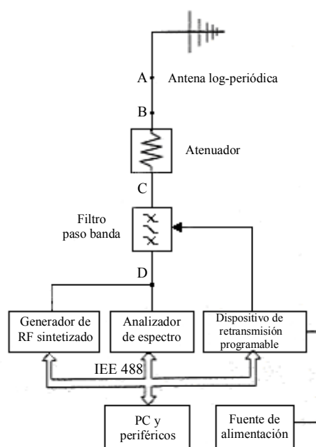
Diagrama de bloques de un dispositivo de medición
