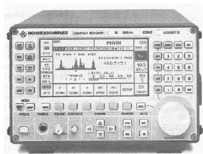
Receptor selectivo con analizador de espectro
