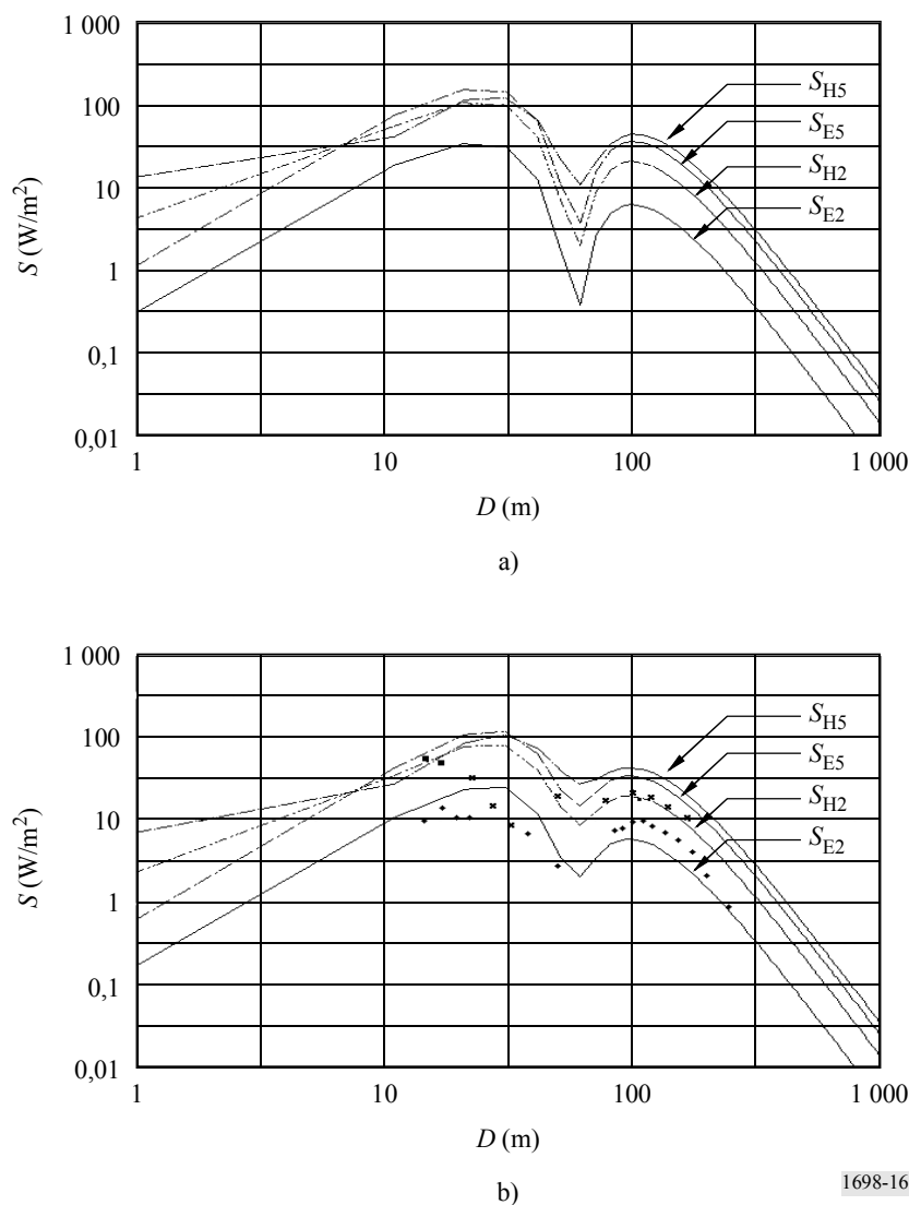
FIGURA 16 Vector de Poynting «equivalente» de la antena HRS 4/4/1, evaluado por el programa AWAS cuando los dipolos están alimentados por a) corrientes idénticas y b) tensiones idénticas, junto con los datos experimentales (curva de puntos)
