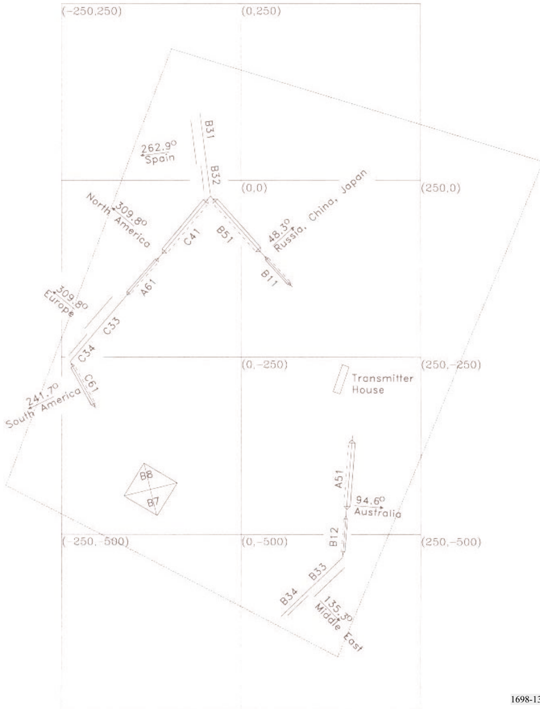
Esquema del campo de antenas del centro de ondas decamétricas de Radio Yugoslavia
