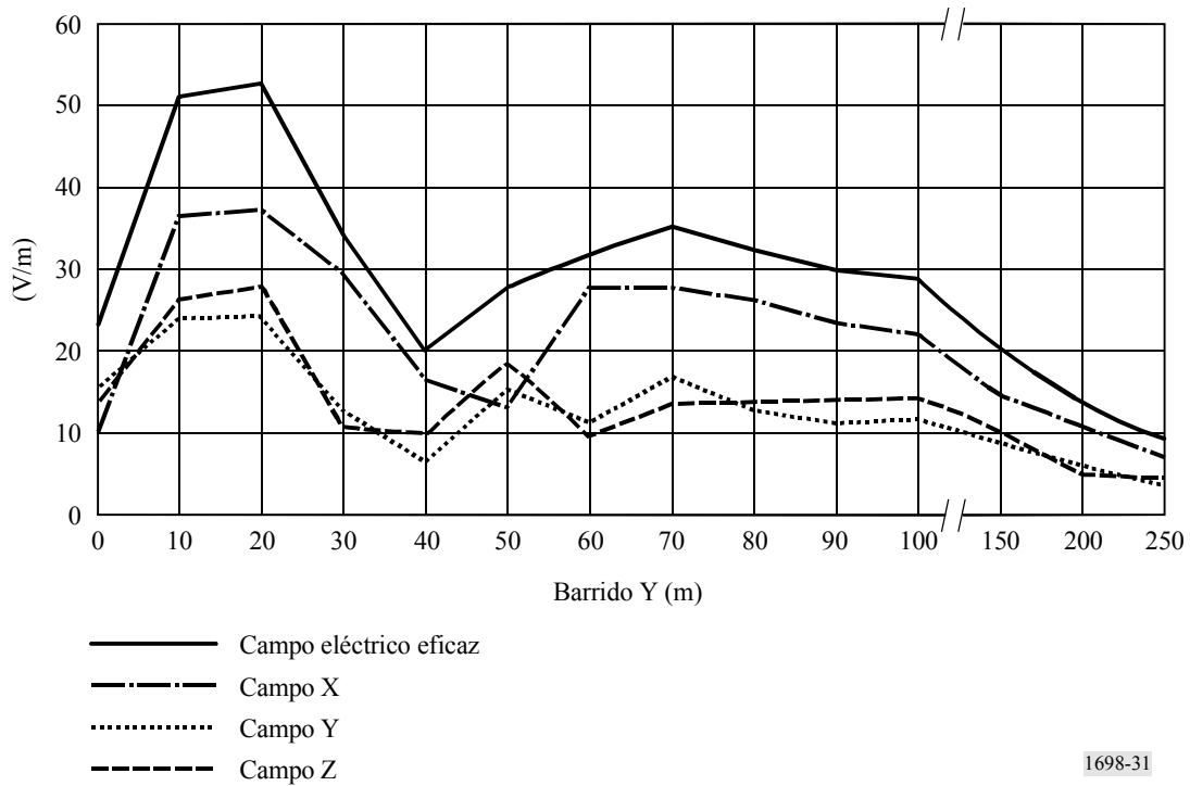
FIGURA 31 Campo E medido
