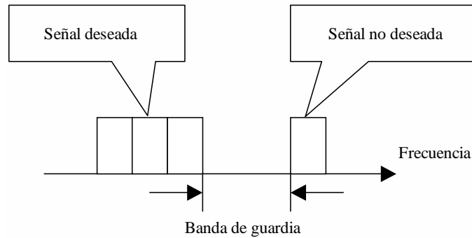
FIGURA 5 Banda de guarda y disposición de las señales
