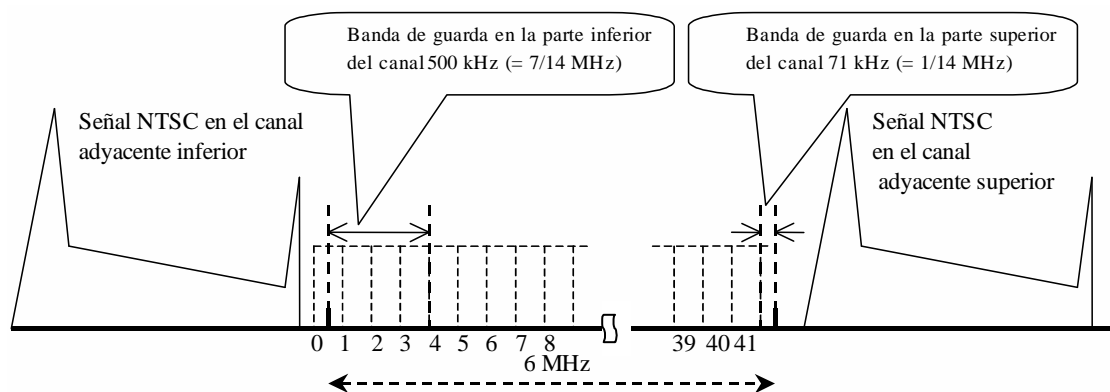
FIGURA 4 Bandas de guarda que coexisten con una señal de televisión analógica adyacente
