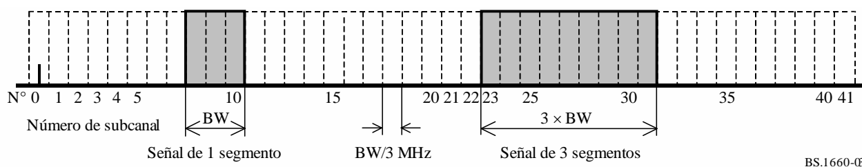
FIGURA 3 Definición de subcanal
