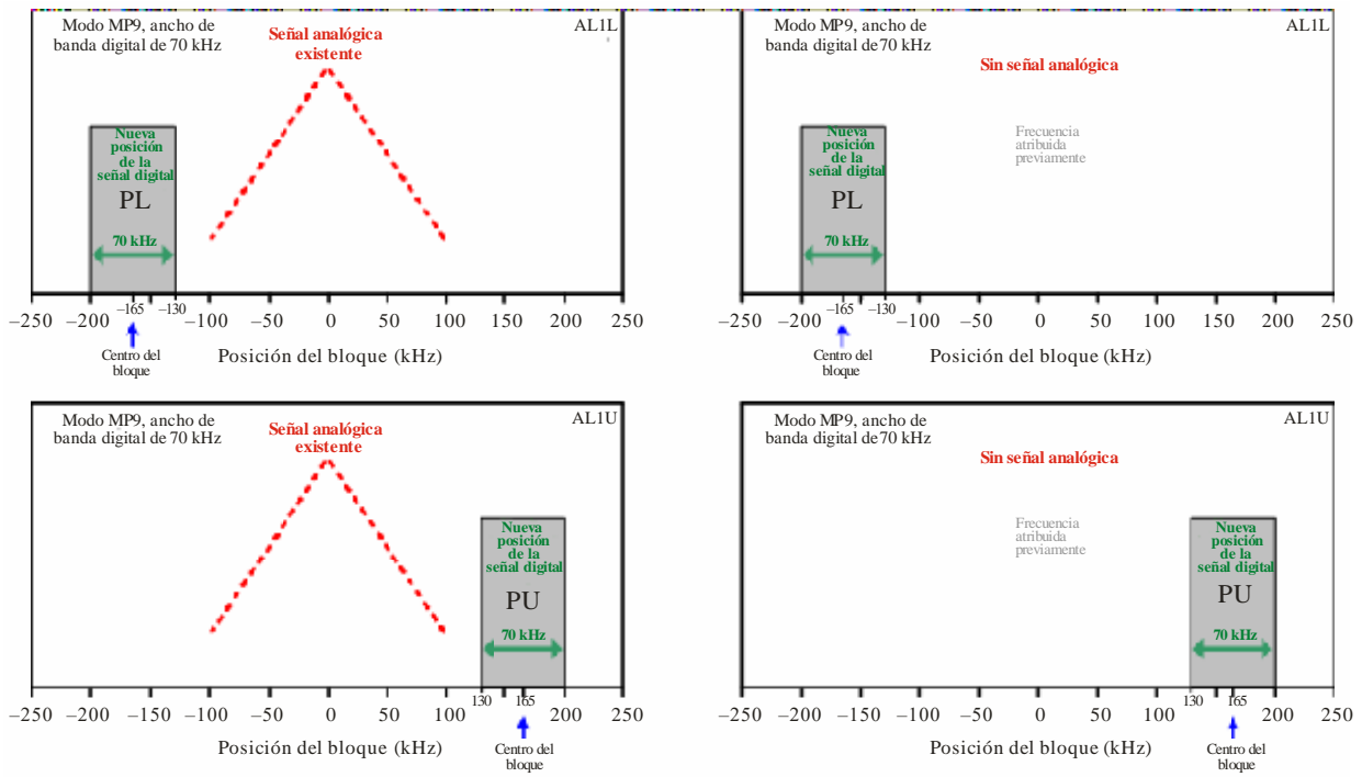
FIGURA 8 Ejemplos de posición de bloques digitales de 70 kHz en el sistema HD Radio
