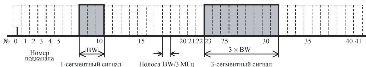
РИСУНОК 8 Определение подканала
