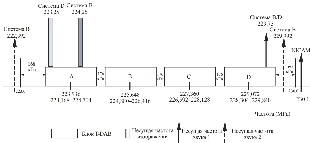
РИСУНОК 2 Позиция блоков T-DAB в канале 12
