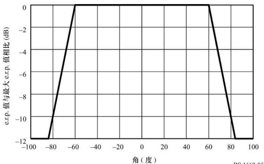
周缘发射机的辐射图
