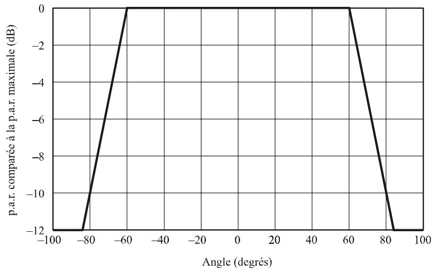
Diagramme de rayonnement des émetteurs périphériques
