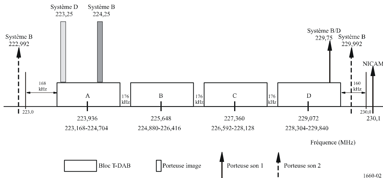
FIGURE 2 Position des blocs T-DAB dans le canal 12
