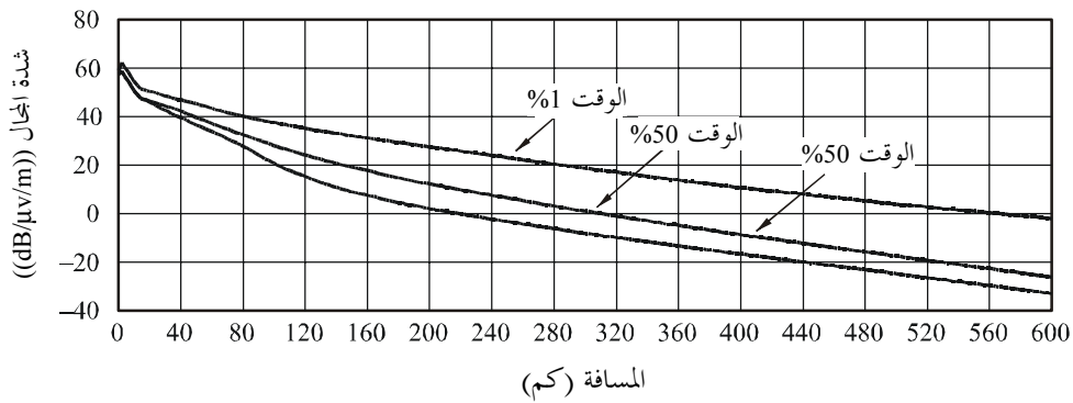
ب) تغير شدة المجال تبعاً للمسافة : على مسار بحري بارد
