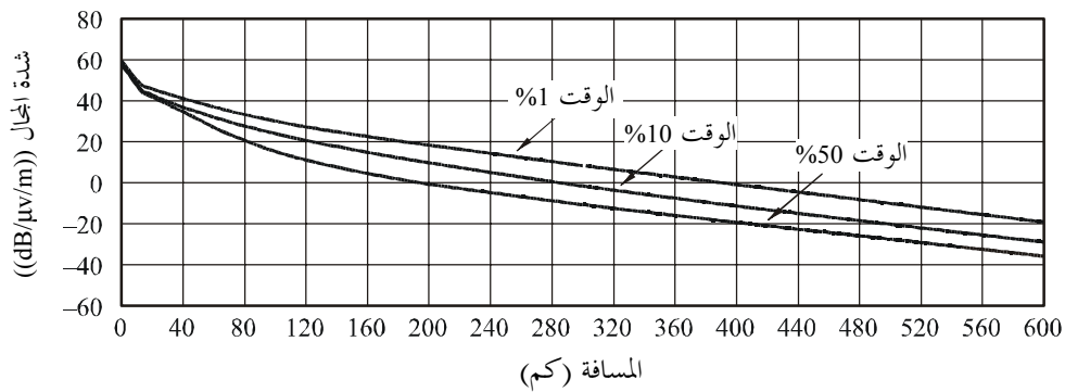
أ) تغير شدة المجال تبعاً للمسافة : على مسار بري
