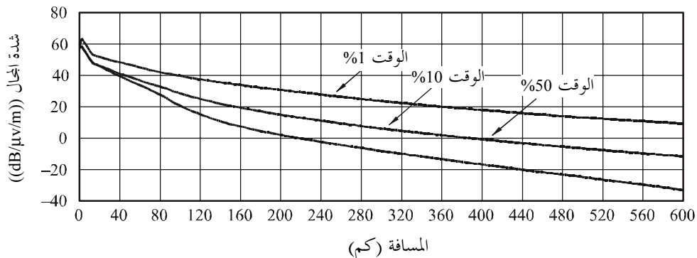
ب) تغير شدة المجال تبعاً للمسافة : على مسار بحري دافئ
