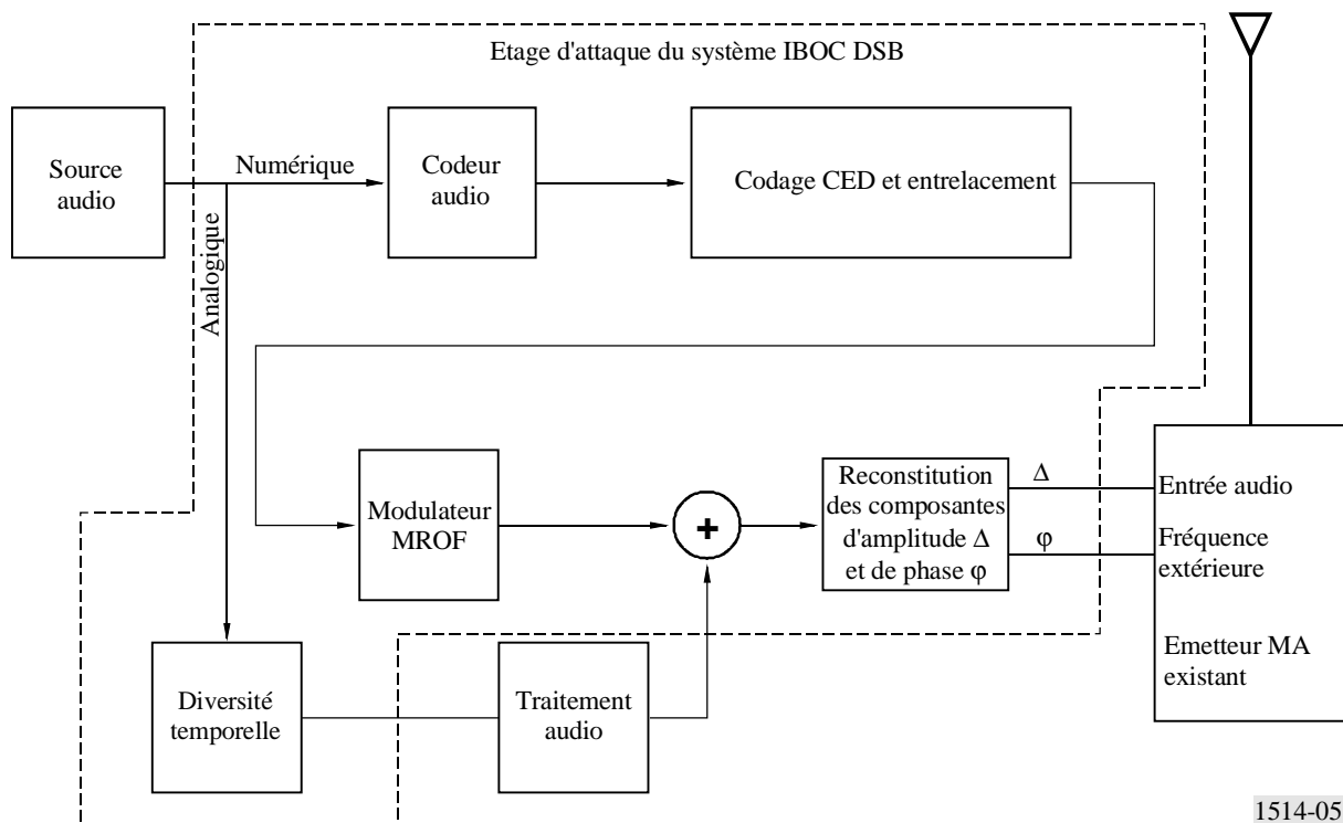
FIGURE 5 Schéma fonctionnel de l'émetteur du système IBOC DSB en ondes hectométriques, mode hybride
