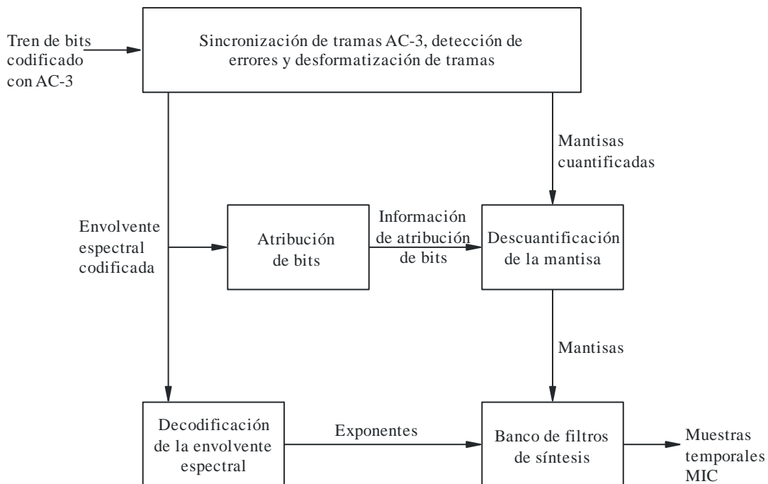
FIGURA 8 Decodificador AC-3
