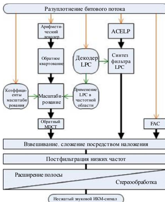
РИСУНОК 13 Блок-схема декодера USAC MPEG-D
