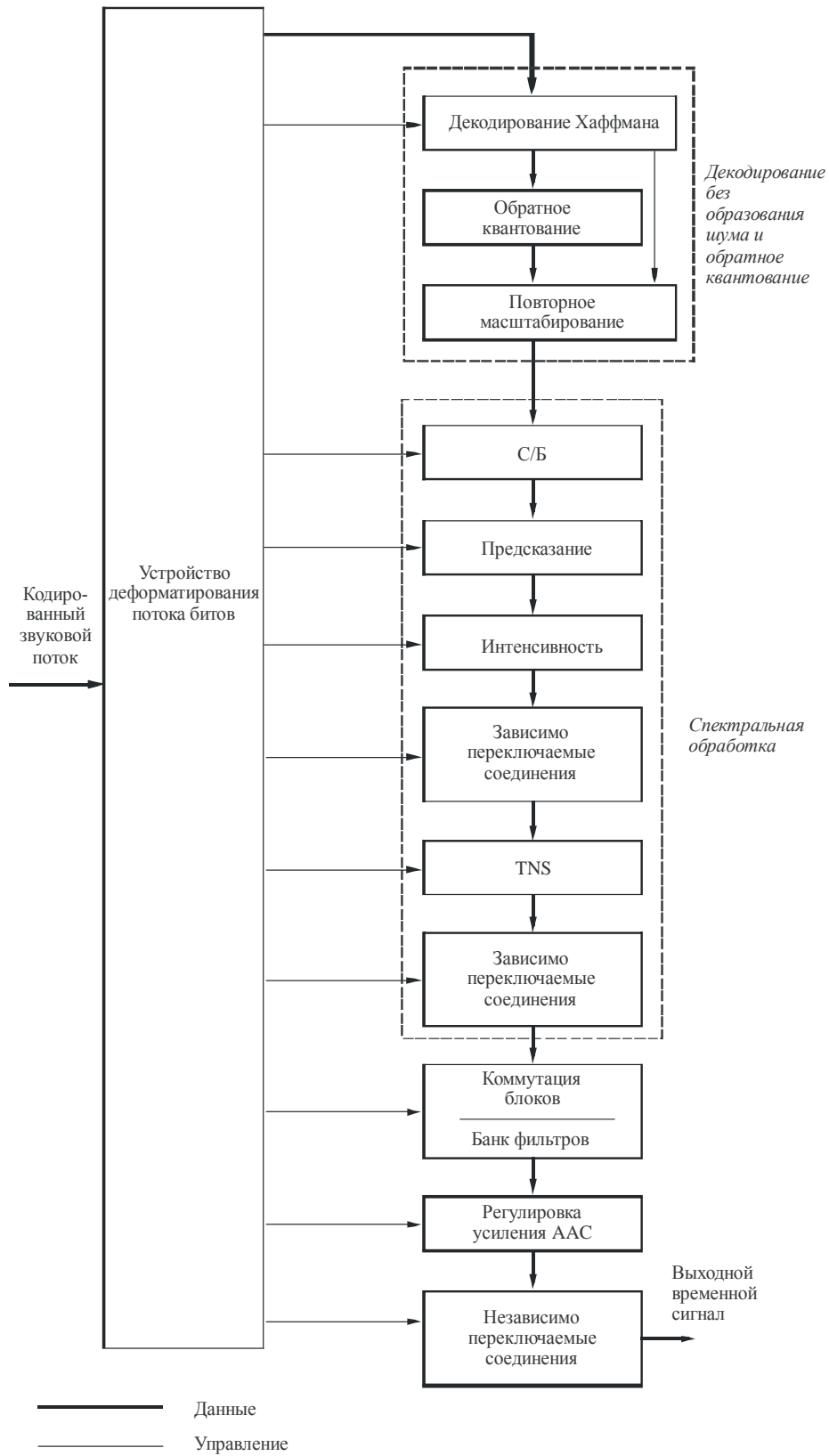
РИСУНОК 6 Функциональная схема декодера AAC MPEG-2
