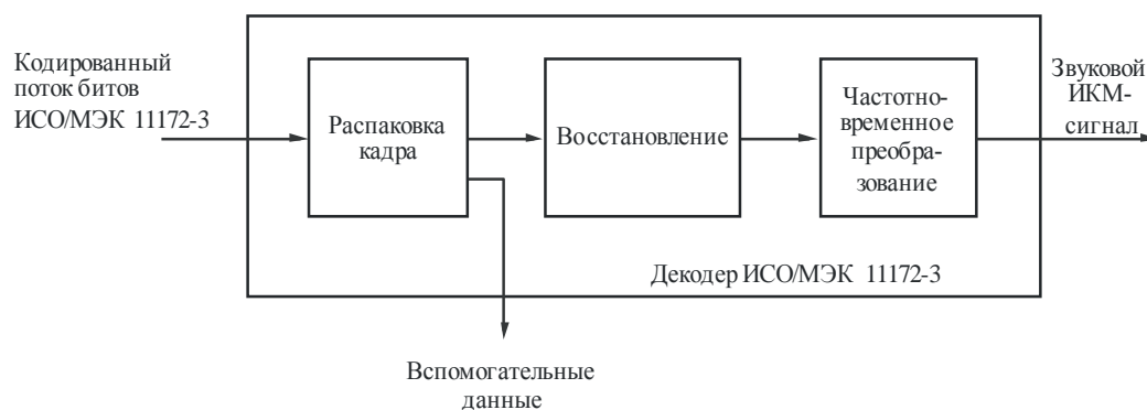
Блок-схема декодера
