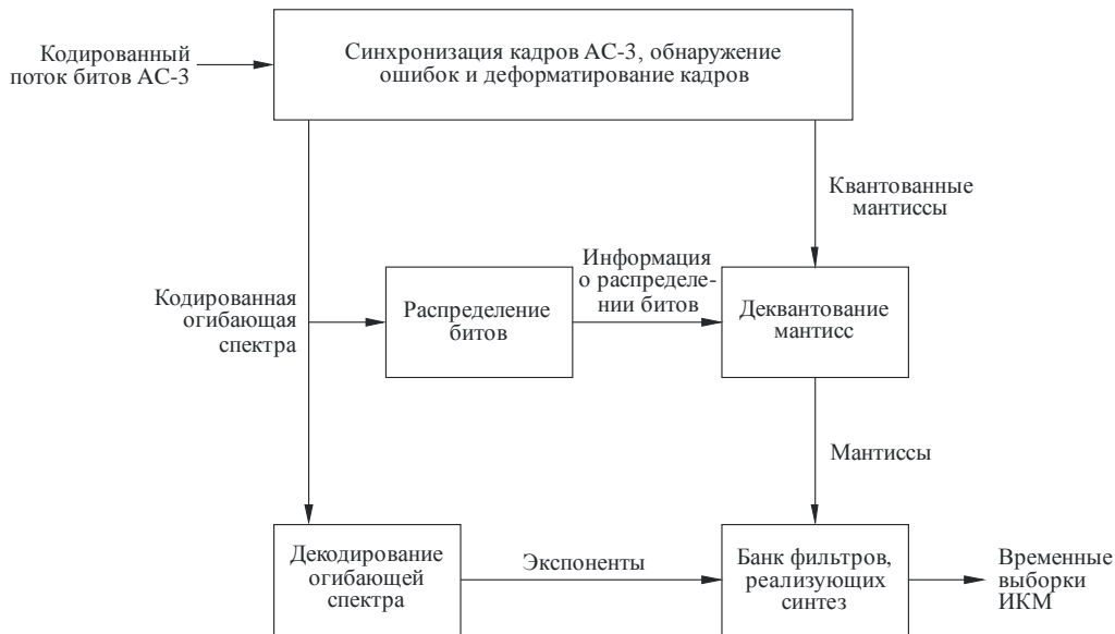
РИСУНОК 8 Декодер АС-3
