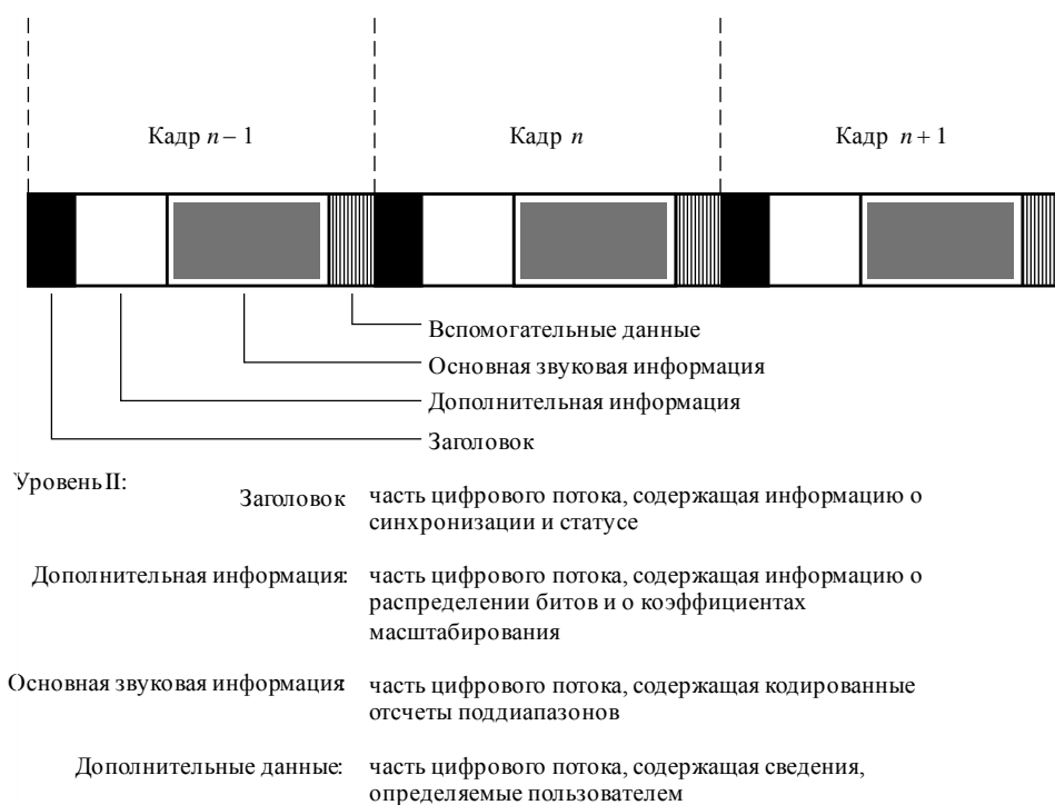
Формат цифрового потока уровня II ИСО/МЭК 11172-3
