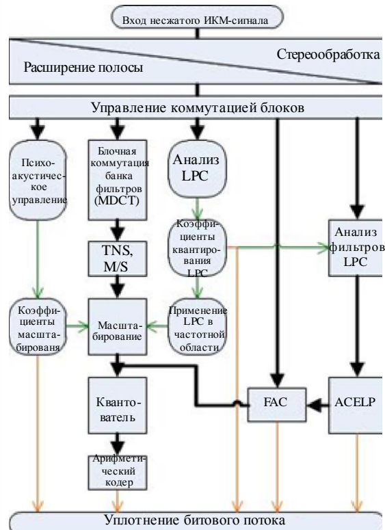
РИСУНОК 12 Блок-схема кодера USAC MPEG-D
