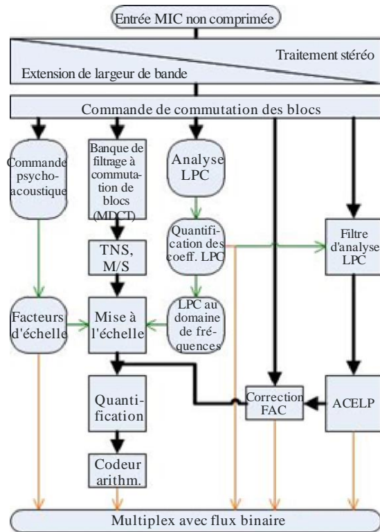
FIGURE 12 Schéma fonctionnel d'un codeur MPEG-D USAC
