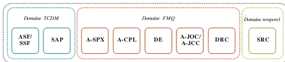
FIGURE 16 Outils de décodage Décodeur AC-4
