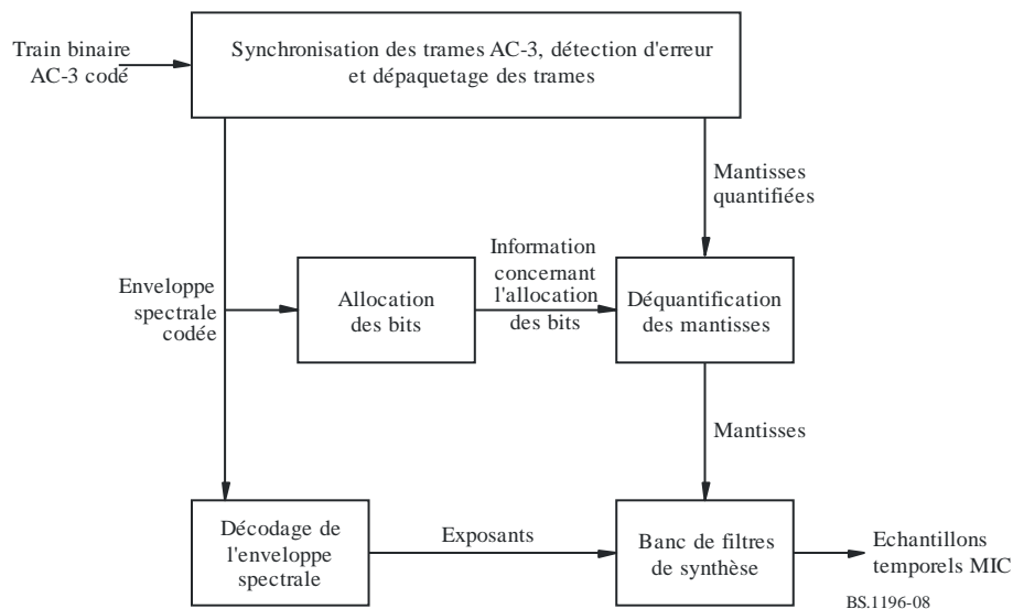
FIGURE 8 Décodeur AC-3
