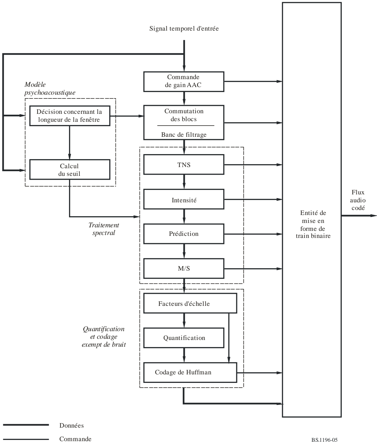
FIGURE 5 Schéma fonctionnel d'un codeur MPEG-2 AAC
