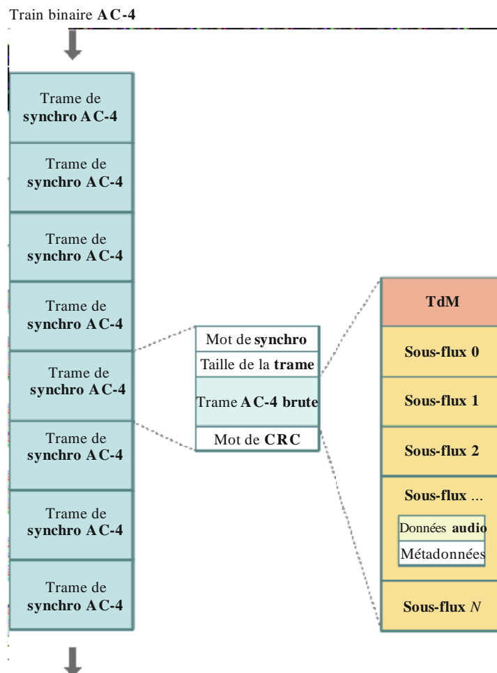
FIGURE 14 Syntaxe du train binaire de haut niveau
