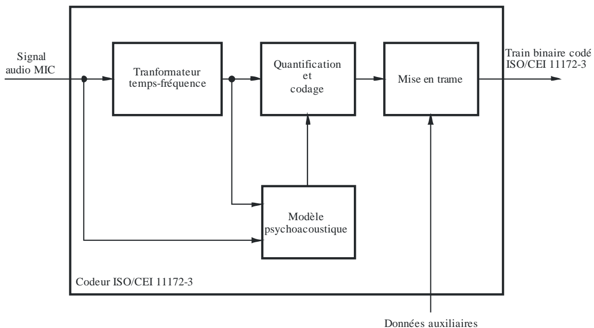
Schéma fonctionnel d'un codeur type
