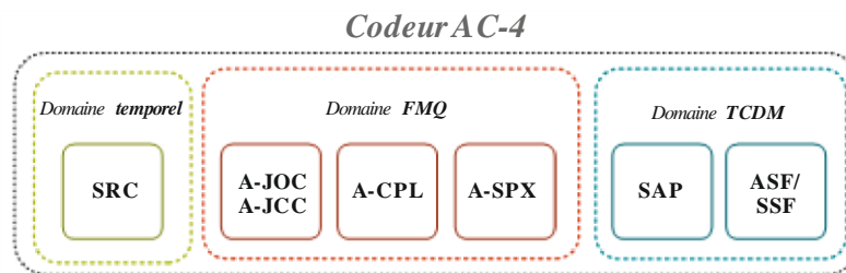
FIGURE 15 Outils de codage disponibles dans le système AC-4
