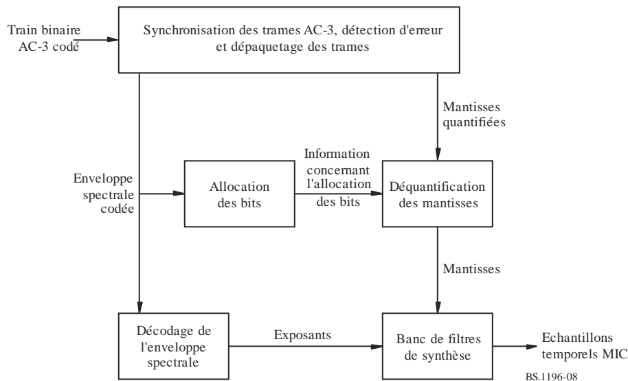
FIGURE 8 Décodeur AC-3
