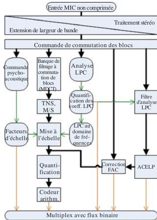
Schéma fonctionnel d'un codeur MPEG-D USAC
