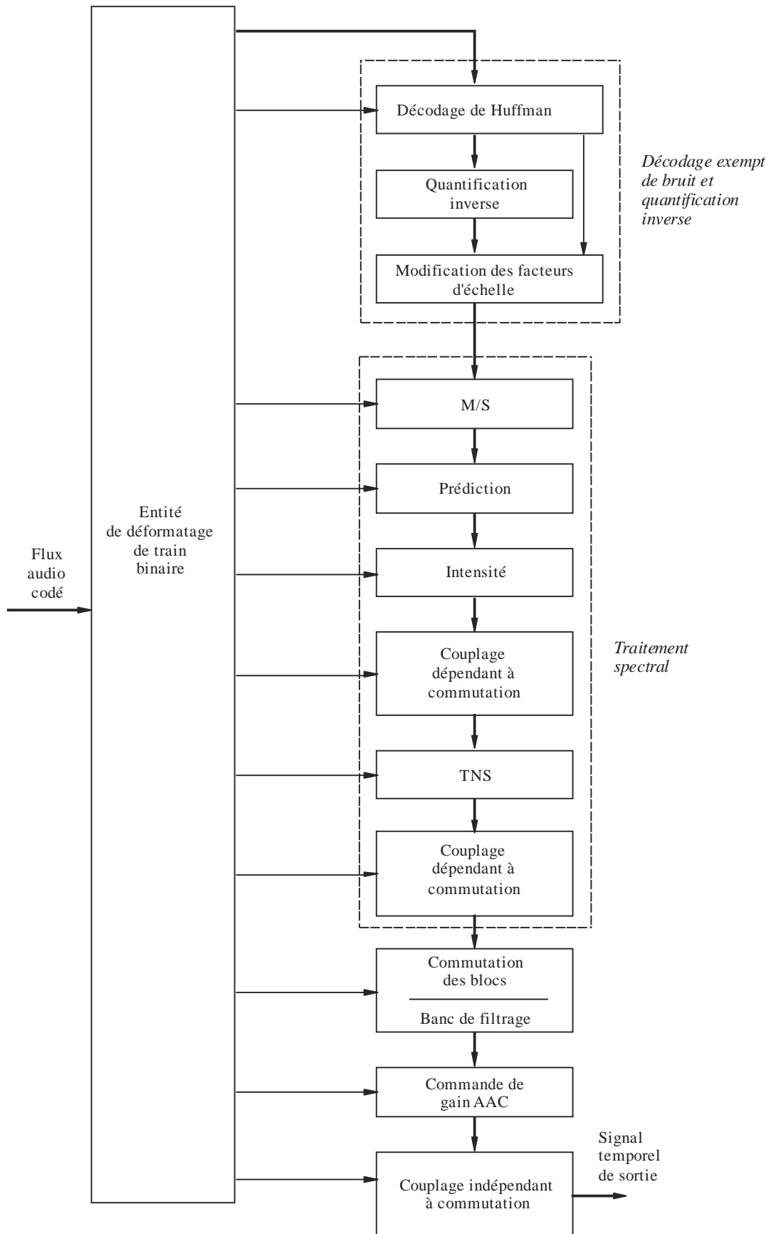
Schéma fonctionnel d'un décodeur MPEG-2 AAC
