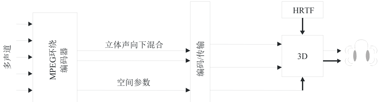
MPEG环绕的虚拟环绕解码过程
