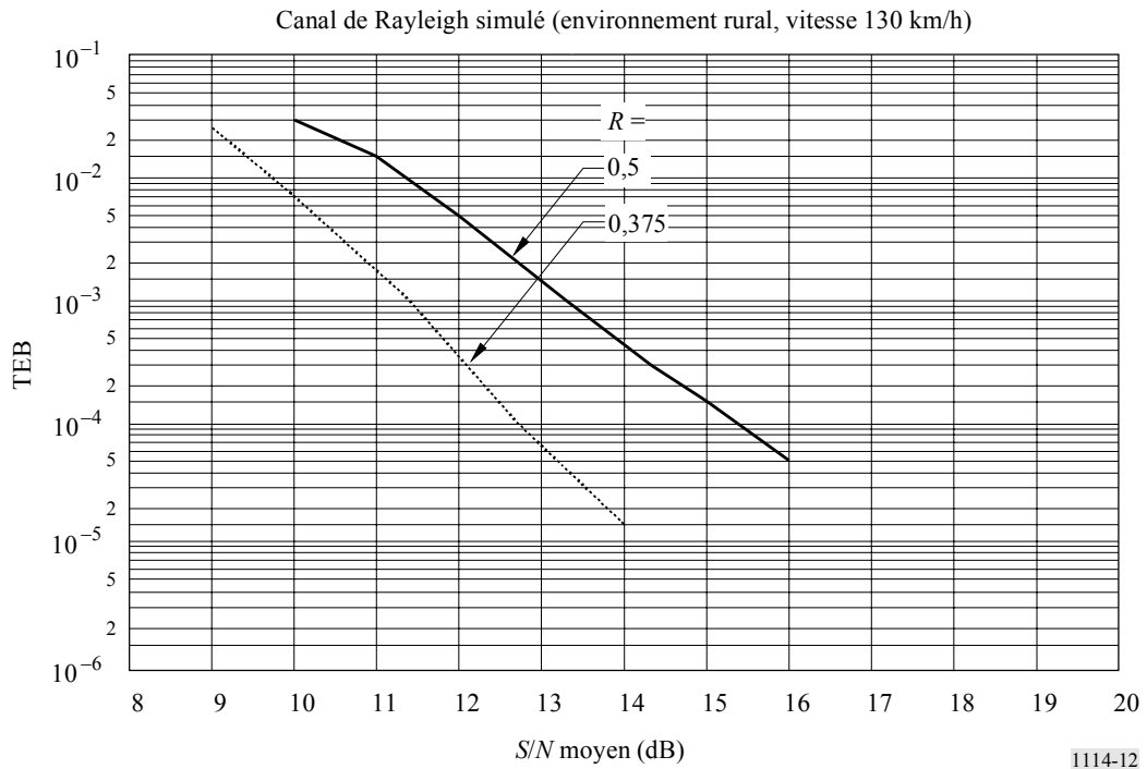
FIGURE 12 TEB en fonction du rapport S/N pour le Système A (Mode de transmission I, 226 MHz)
