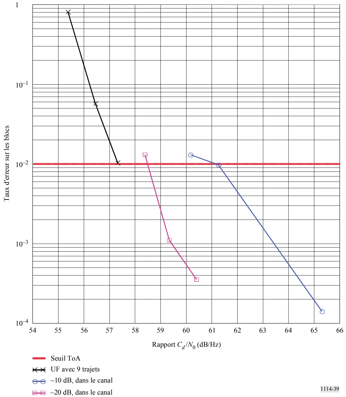
FIGURE 39 Taux d'erreur sur les blocs du système hybride avec un brouilleur à 10 canaux à évanouissement individuel
