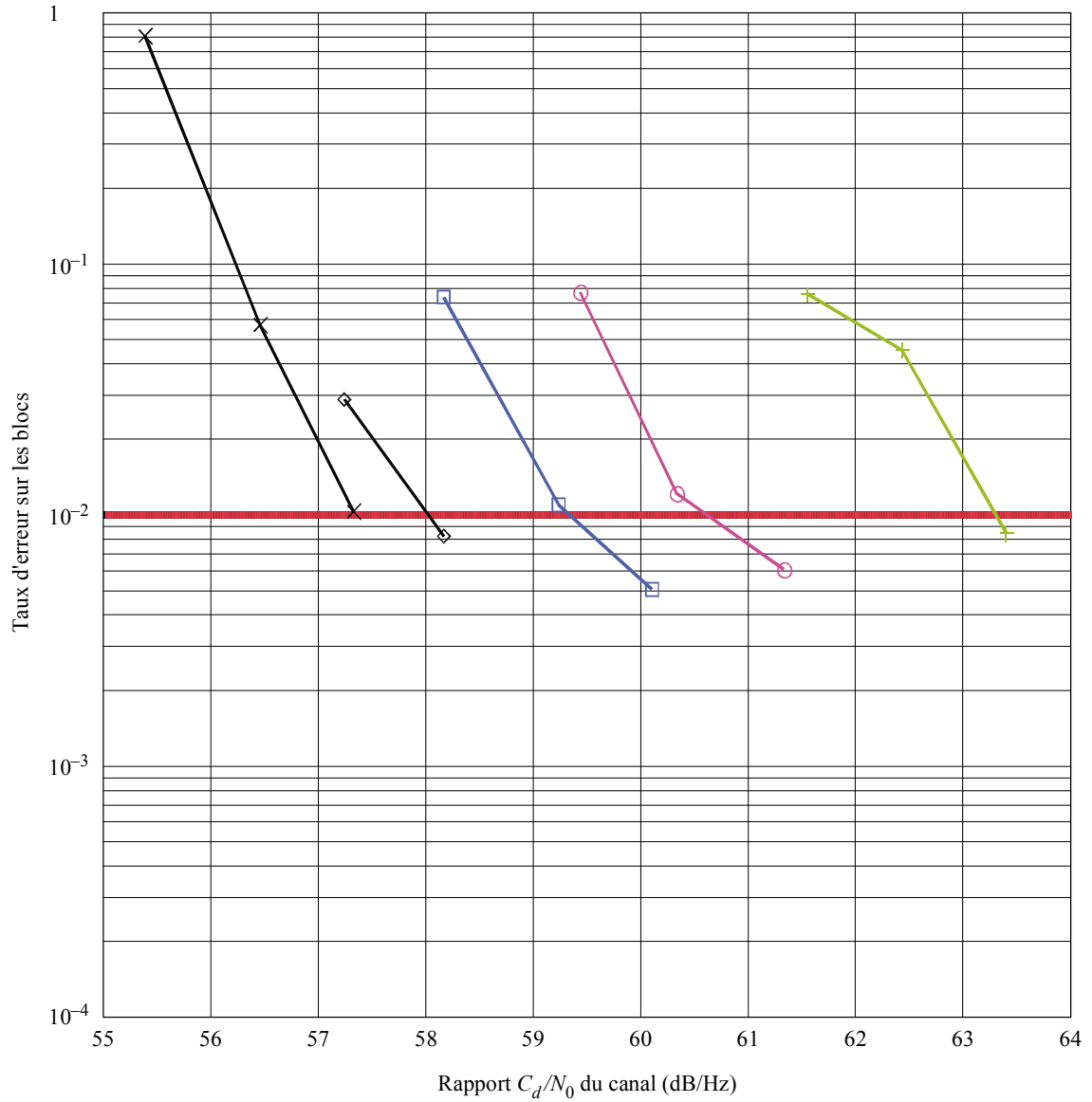
FIGURE 38 Taux d'erreur sur les blocs d'un système hybride dans un environnement urbain à 9 trajets à évanouissement rapide avec un brouilleur du premier canal adjacent à évanouissement individuel
