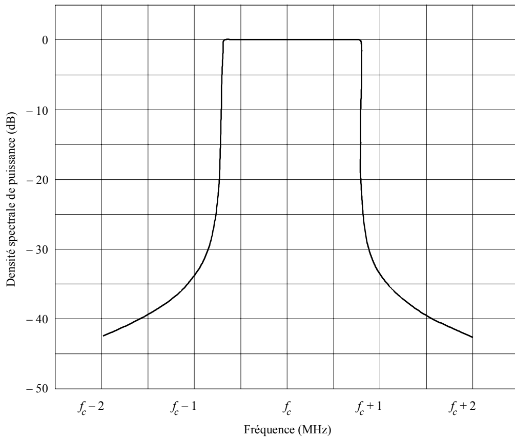
FIGURE 6 Spectre d'émission théorique du Système A (Mode de transmission II)
