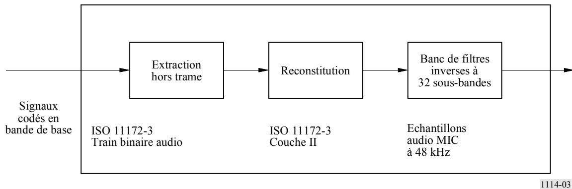
Diagramme fonctionnel du système décodeur audio de base
