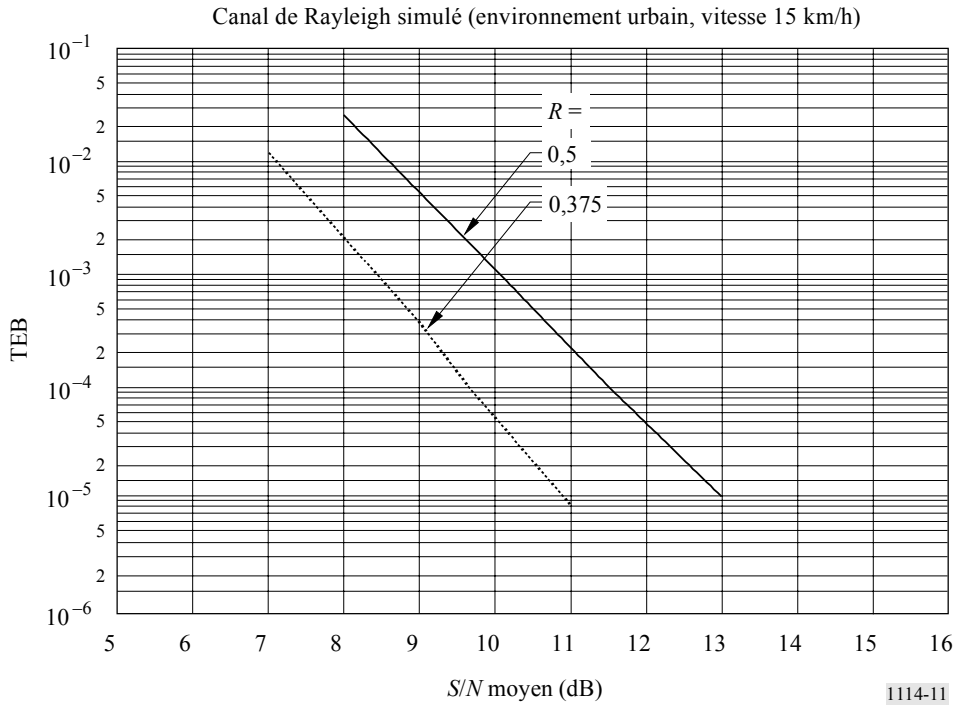
FIGURE 11 TEB en fonction du rapport S/N pour le Système A (Mode de transmission II, 1 480 MHz)
