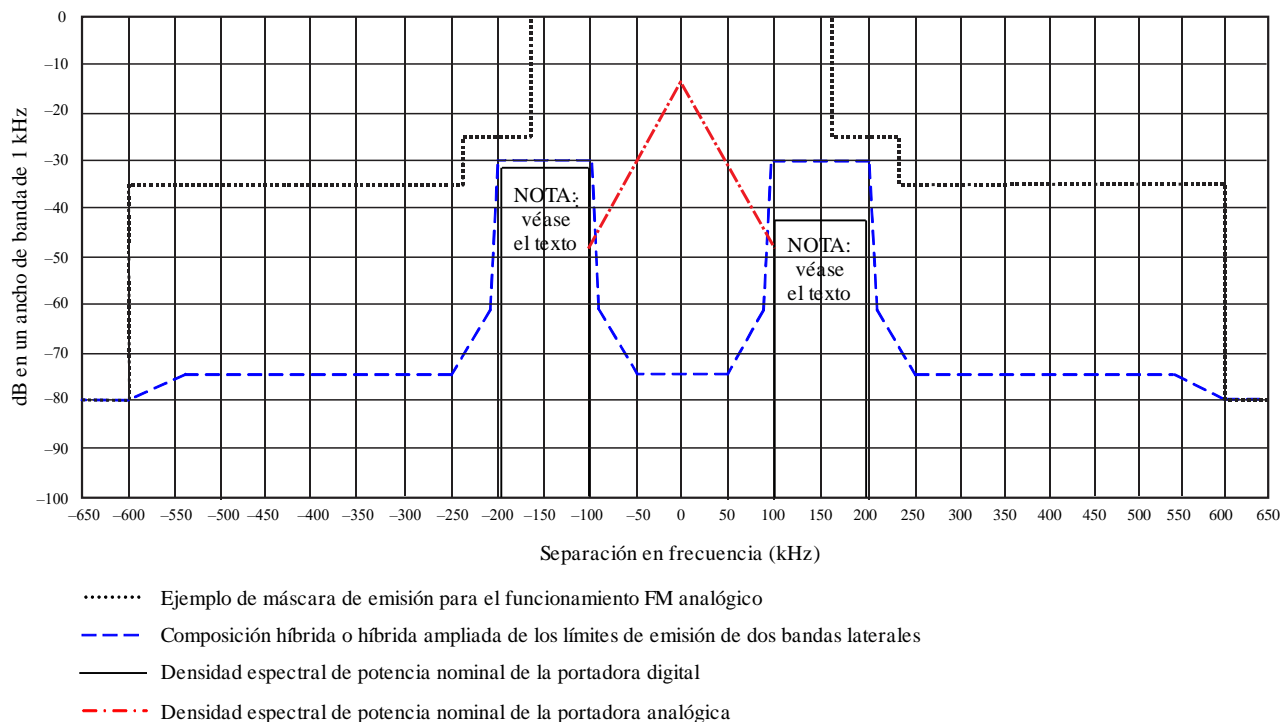
FIGURA 31 Límites de la emisión en modo híbrido IBOC*
