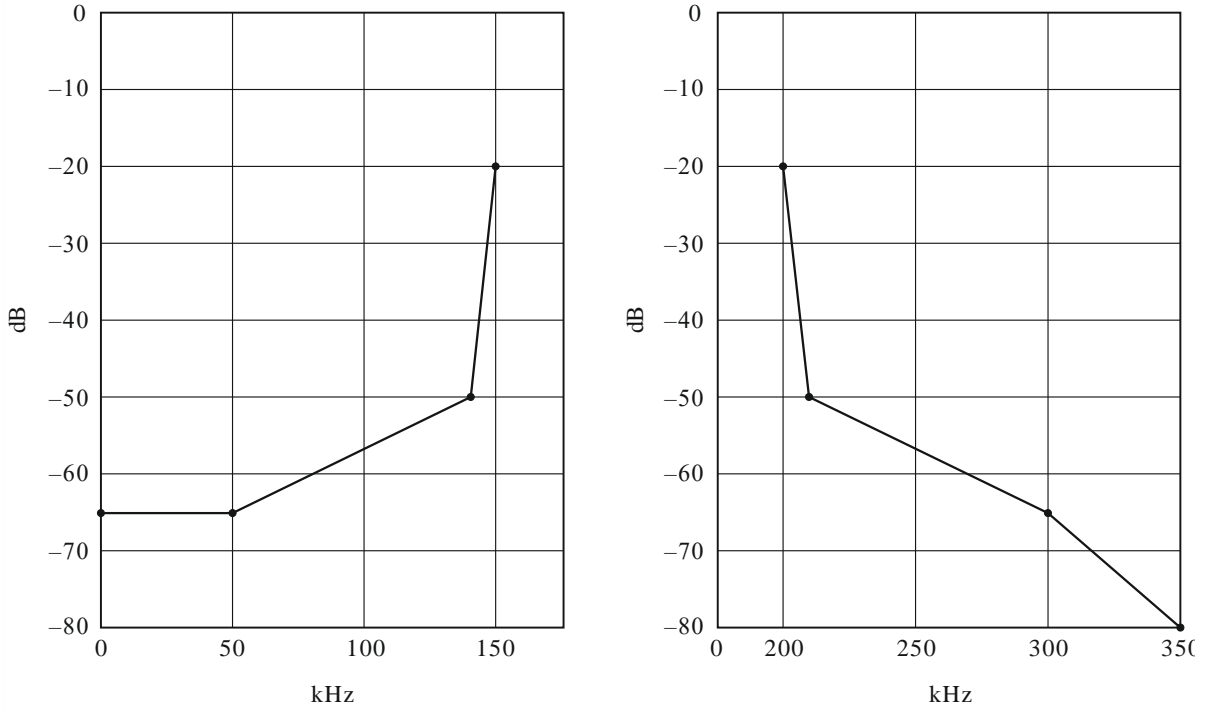
FIGURA 49 Curva espectral para el modo espectral C
