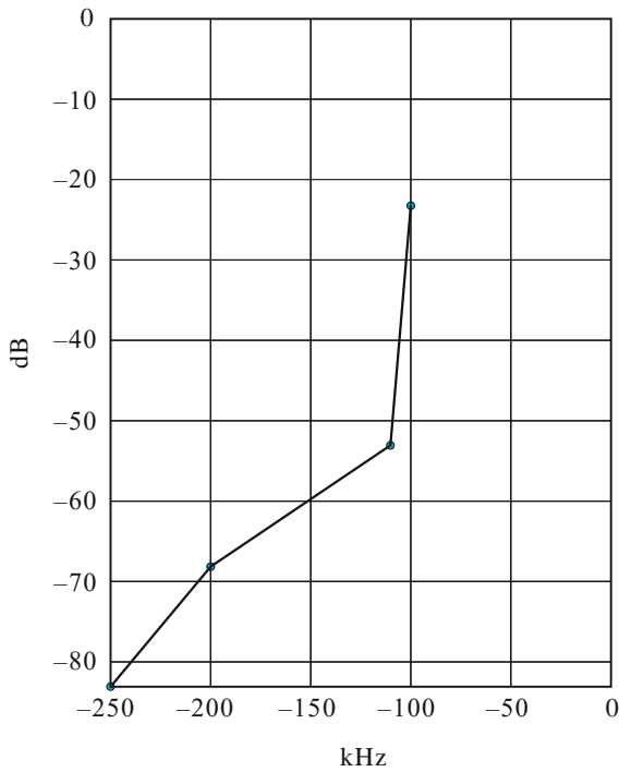
Curva espectral para el modo espectral B
