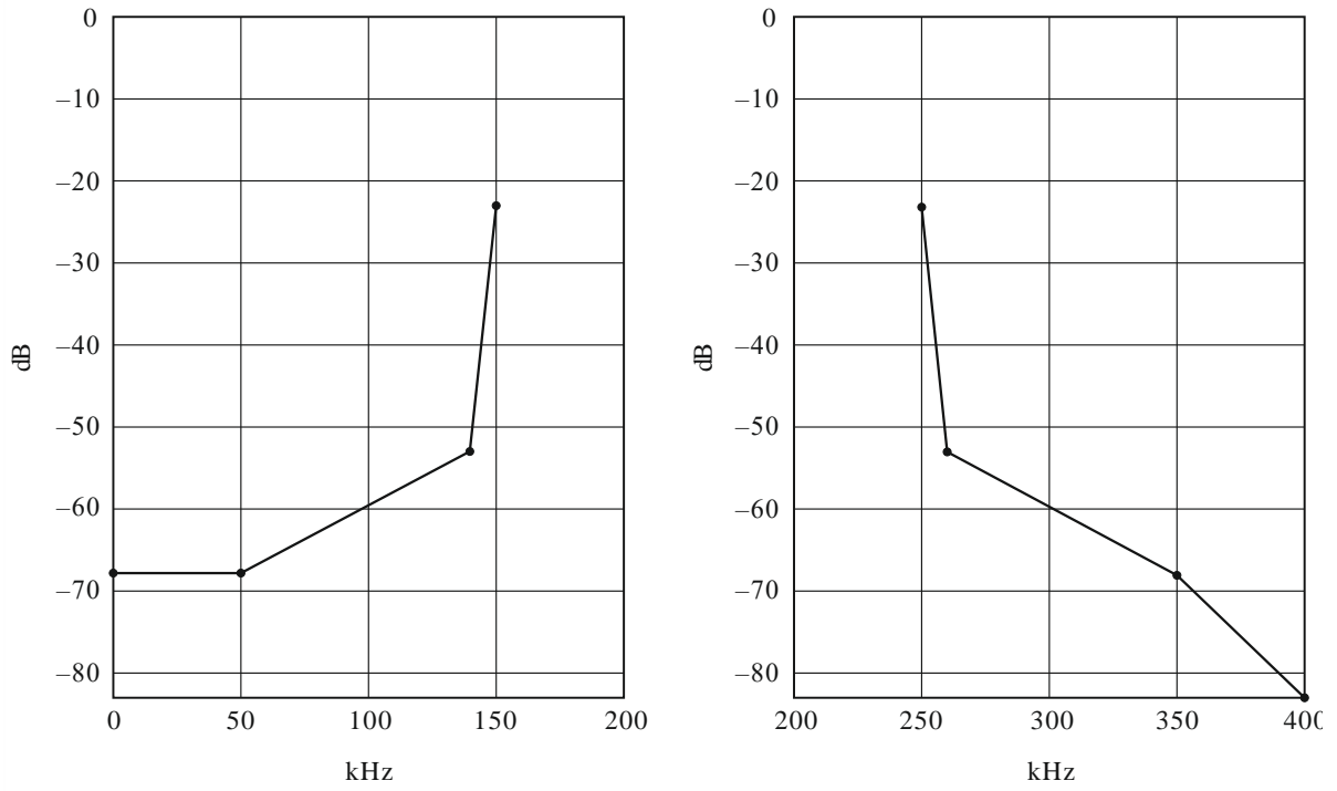
FIGURA 50 Curva espectral para el modo espectral D
