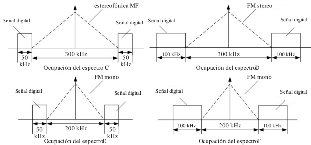
Diagrama del espectro de difusión simultánea
