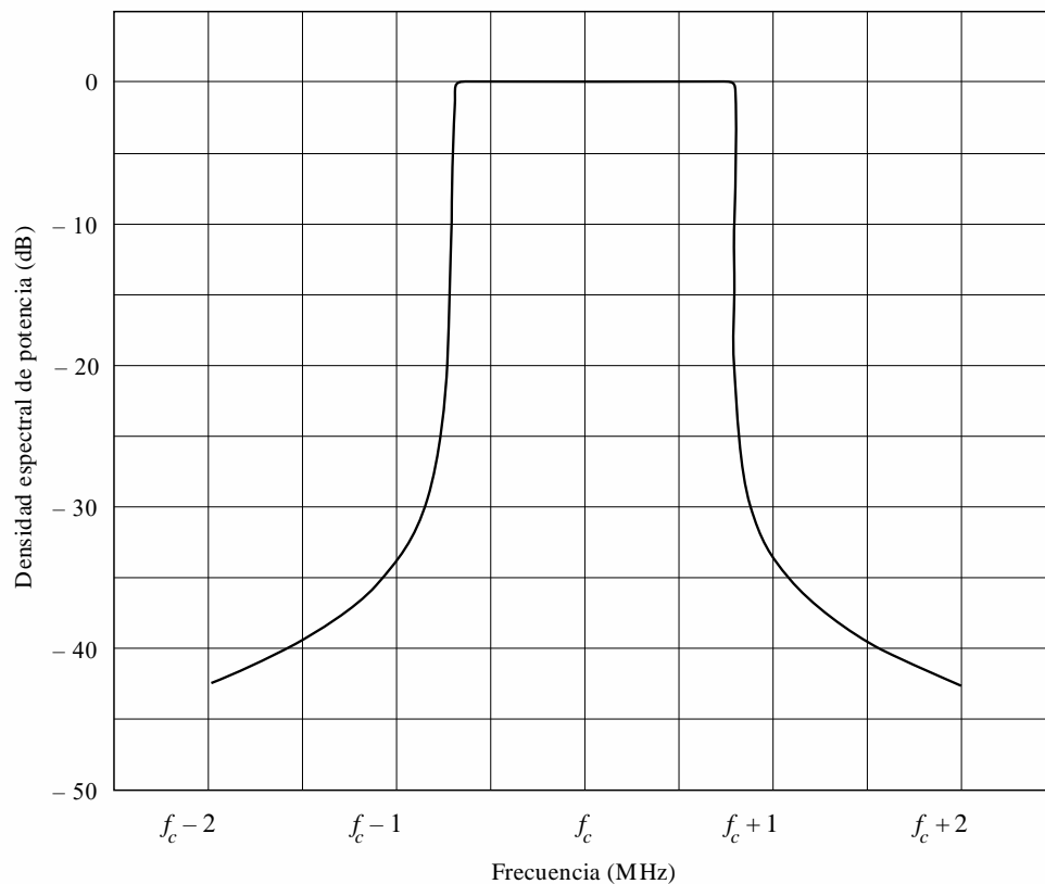
FIGURA 3 Espectro teórico de la señal de transmisión del Sistema A en Modo II
