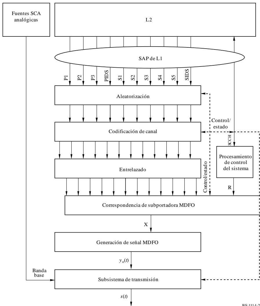
FIGURA 25 Diagrama de bloques funcional de L1 de la interfaz aérea de MF
