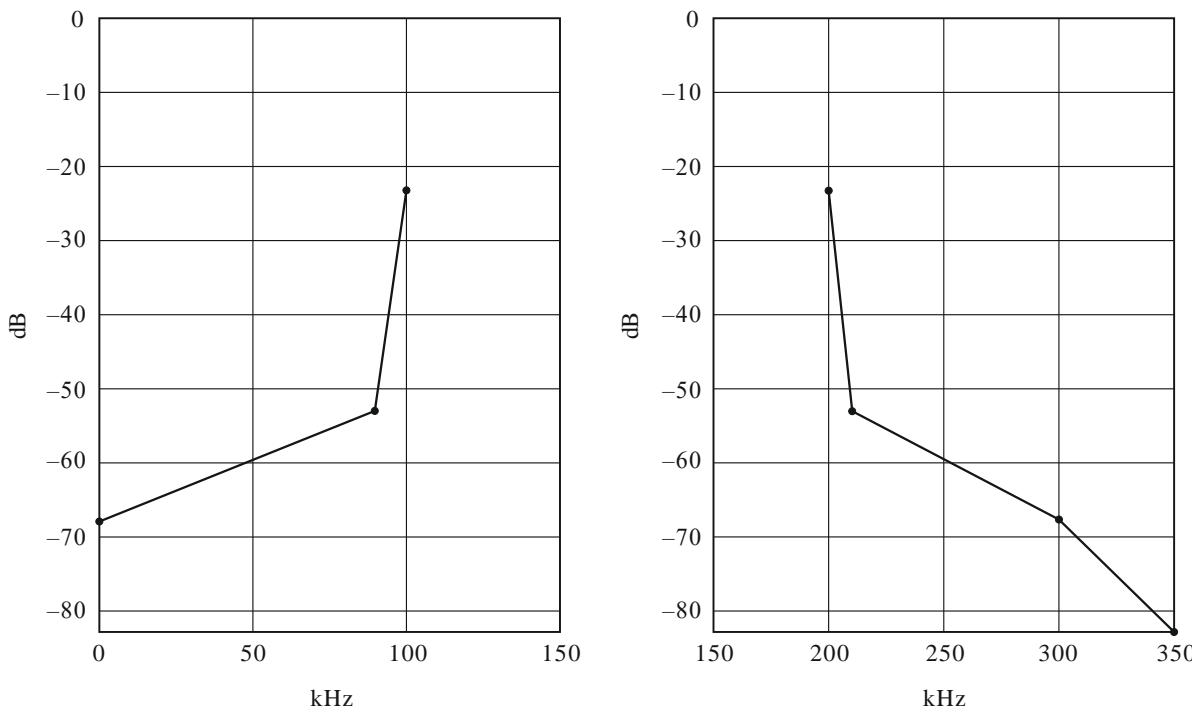
FIGURA 52 Curva espectral para el modo espectral F
