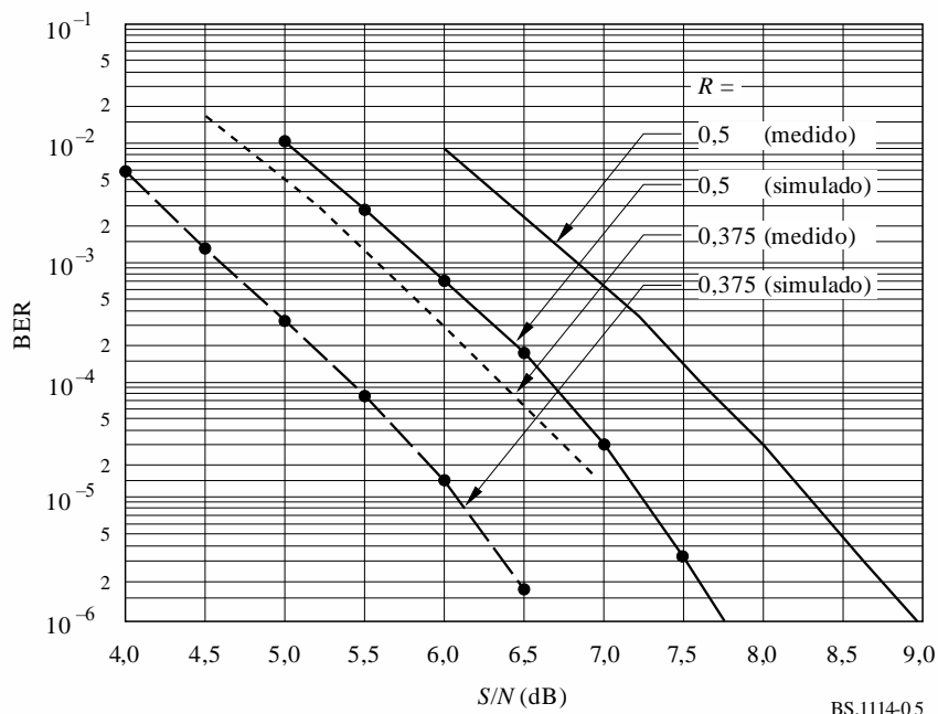
FIGURA 5 BER en función de la relación S/N para el Sistema A Canal gaussiano
