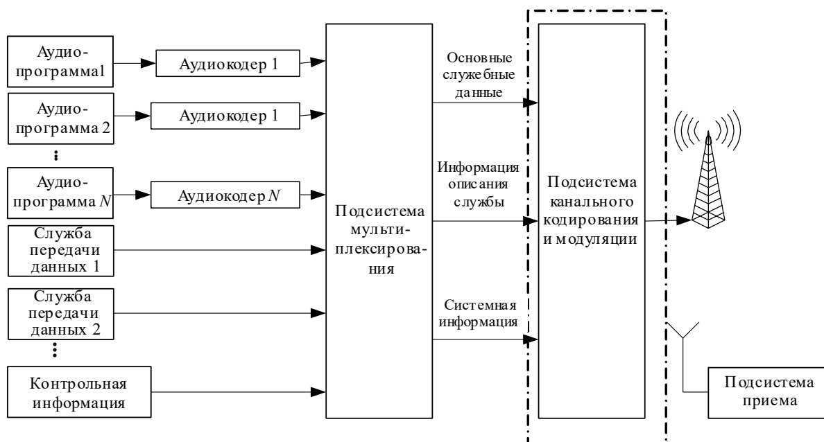
РИСУНОК 42 Обзор системы
