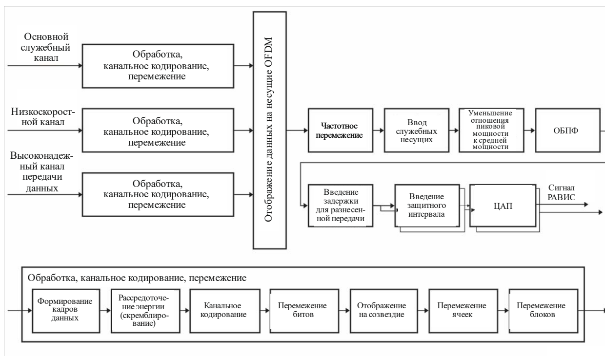
Функциональная блок-схема передатчика РАВИС
