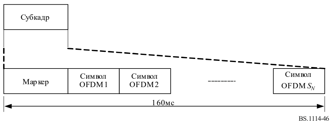
РИСУНОК 46 Структура субкадра
