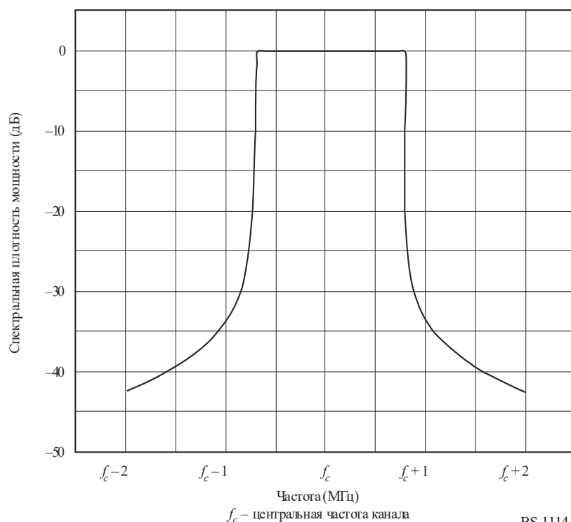
Расчетный спектр сигнала передачи в системе А при передаче в режиме II
