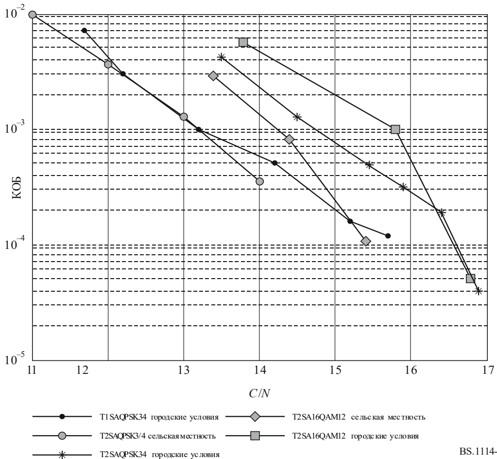
КОБ в зависимости от отношения C/N в многолучевом канале
