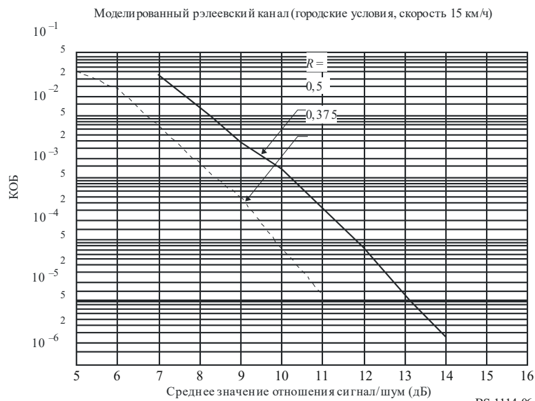
РИСУНОК 6 Зависимость КОБ от отношения сигнал/шум для системы А (передача в режиме I, 226 МГц)
