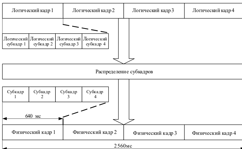
РИСУНОК 44 Логический кадр и распределение субкадров
