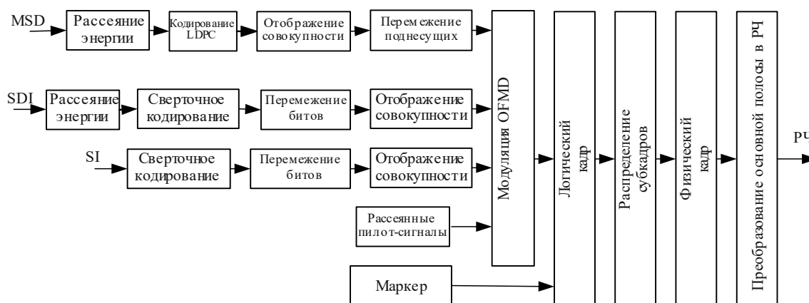
РИСУНОК 45 Блок-схема кодирования каналов и модуляции
