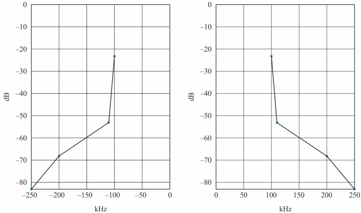
Gabarit spectral du mode d'occupation spectrale B
