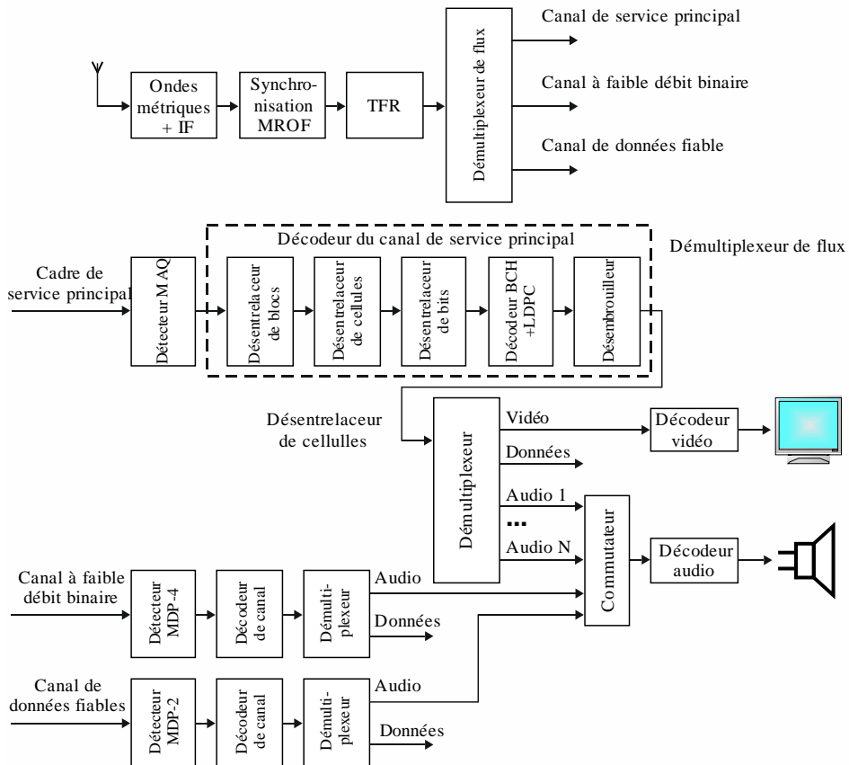
Schéma fonctionnel d'un récepteur du système RAVIS
