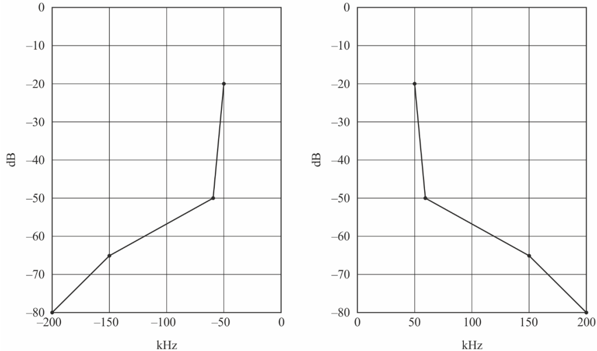
Gabarit spectral du mode d'occupation spectrale A
