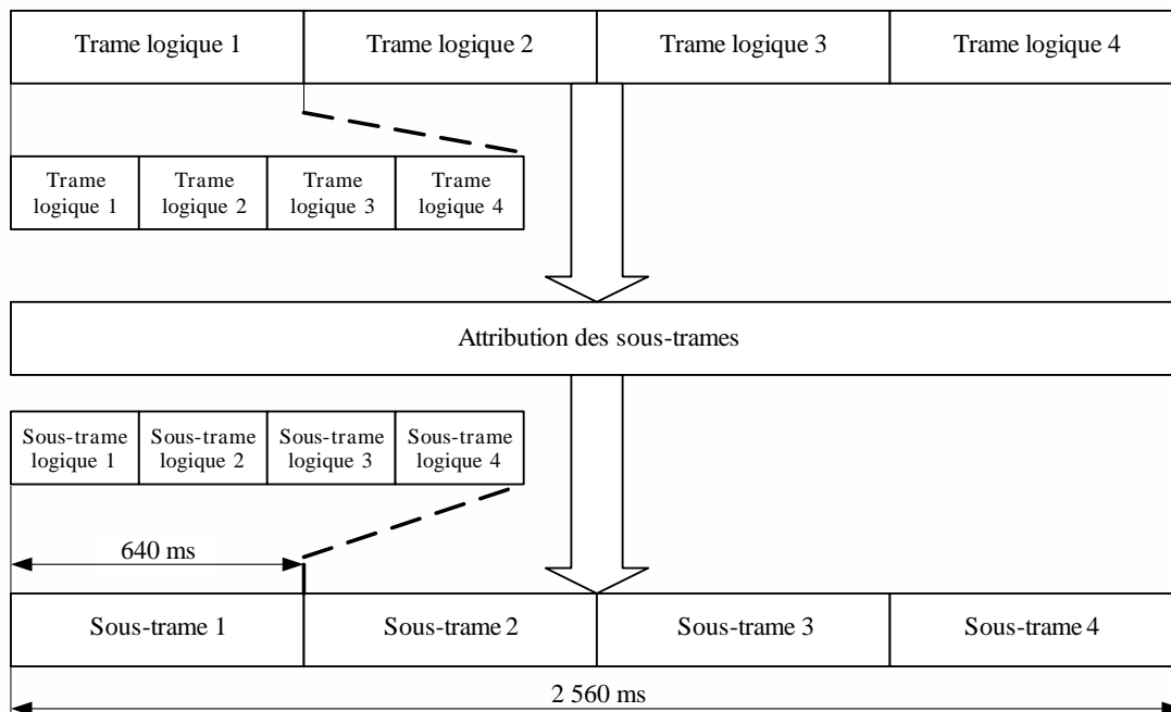
FIGURE 44 Trame logique et attribution des sous trames
