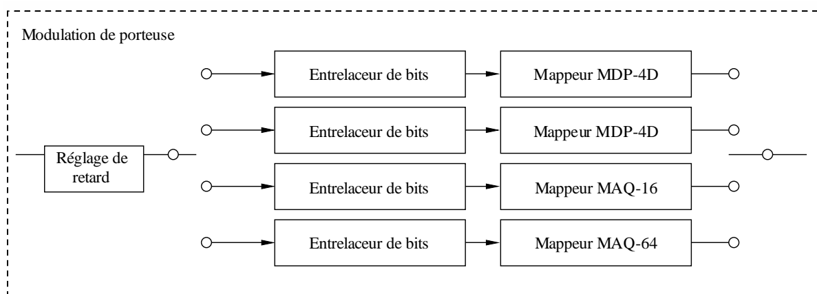
Configuration du bloc de modulation de porteuse
