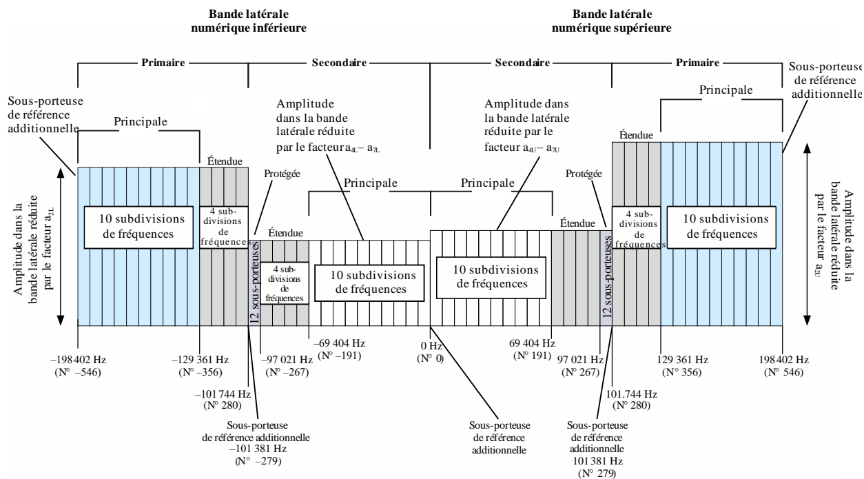
Spectre pour la forme d'onde tout numérique – Modes de service MP5, MP6 et MP12, MS1 à MS4
