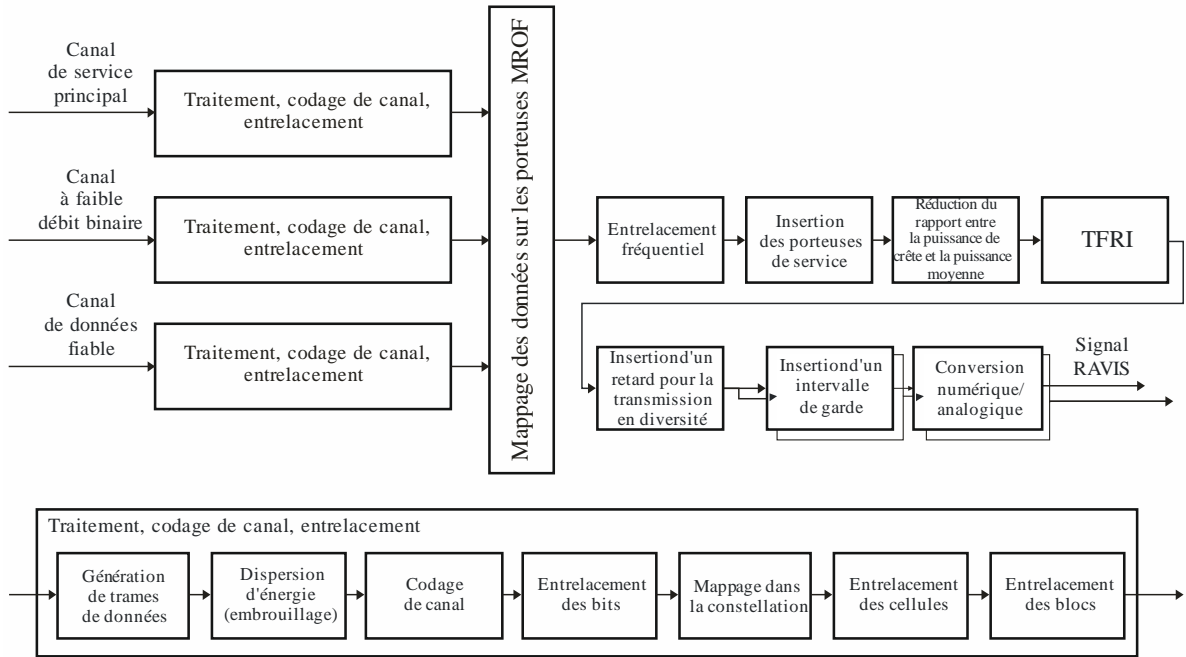
Schéma fonctionnel d'un émetteur du système RAVIS
