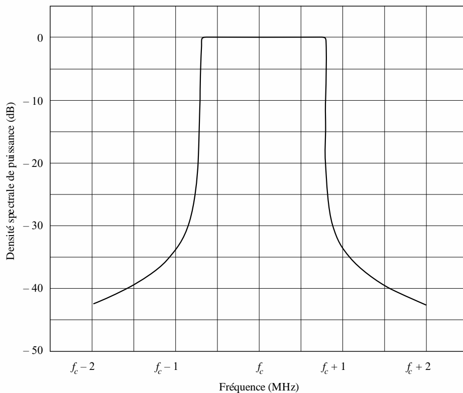
FIGURE 3 Spectre d'émission théorique du Système A (Mode de transmission II)
