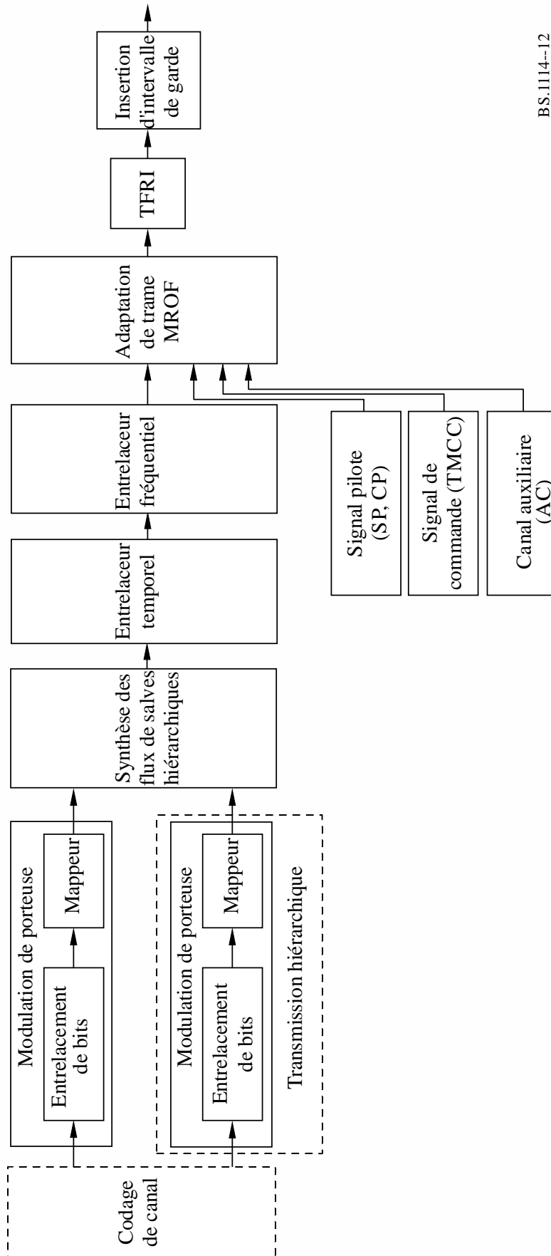
Diagramme de bloc de modulation
