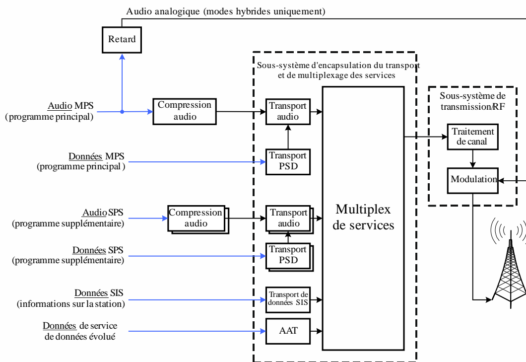
FIGURE 21 Aperçu du système de radiodiffusion IBOC
