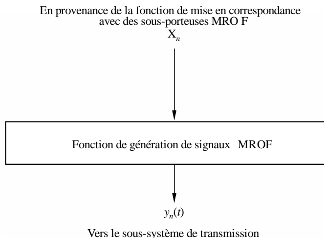
FIGURE 26 Schéma conceptuel de la fonction de génération de signaux MROF
