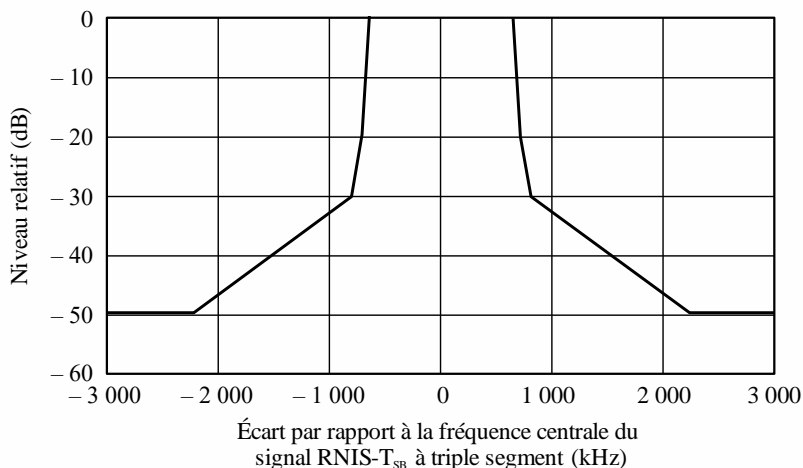
Masque spectral pour signal RNIS-T à triple segment (largeur de bande du segment = 6/14 MHz)
