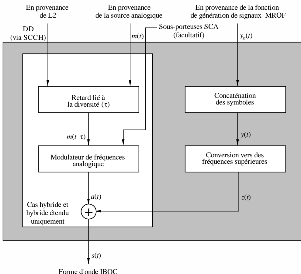
Schéma fonctionnel du sous-système de transmission dans le cas hybride ou hybride étendu
