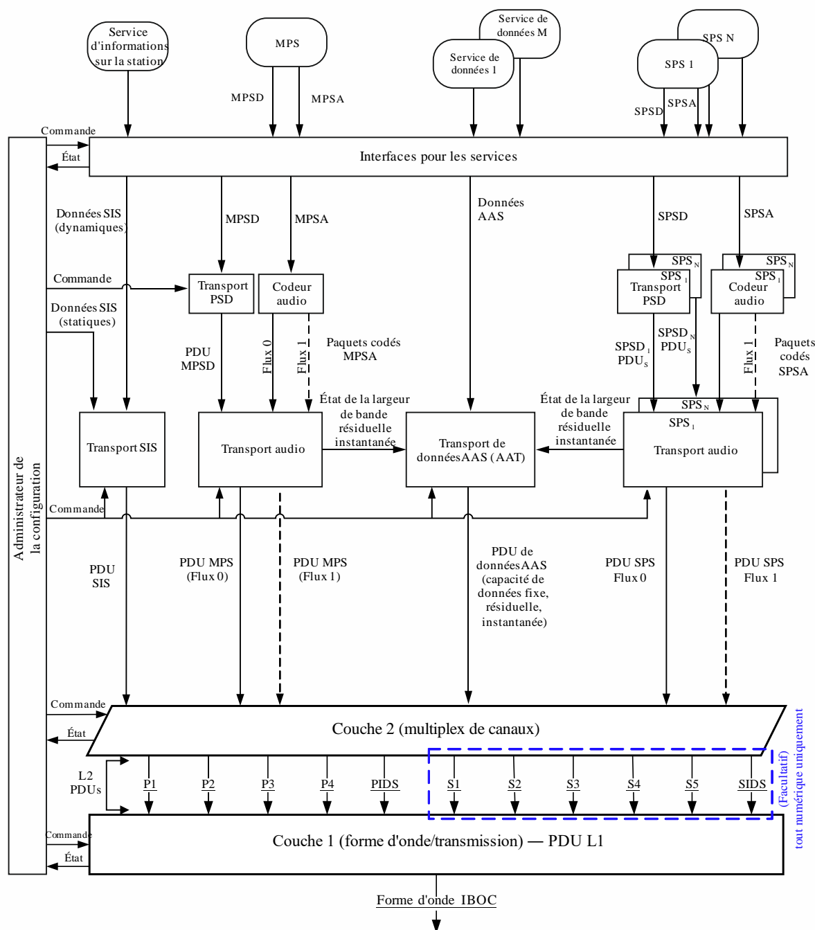
FIGURE 22 Schéma de la pile de protocoles du système MF IBOC
