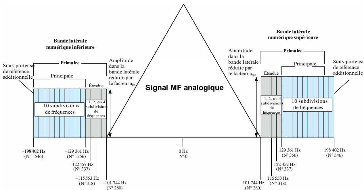
Spectre pour la forme d'onde hybride étendue – Modes de service MP2, MP3, MP11, MP12, MP5 et MP6
