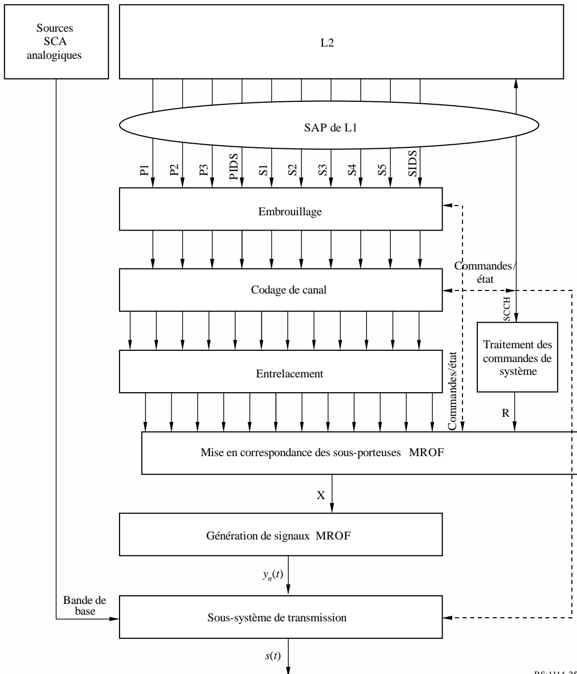
FIGURE 25 Schéma fonctionnel de L1 à l'interface radioélectrique MF
