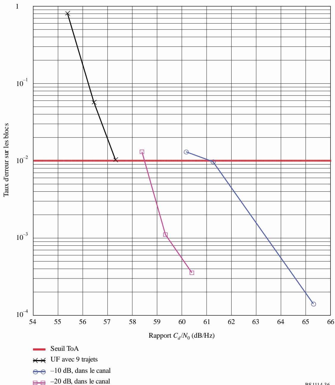
FIGURE 36 Taux d'erreur sur les blocs du système hybride avec un brouilleur à 10 canaux à évanouissement individuel
