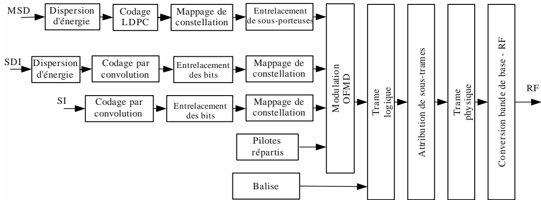
Schéma fonctionnel de codage de canal et de modulation
