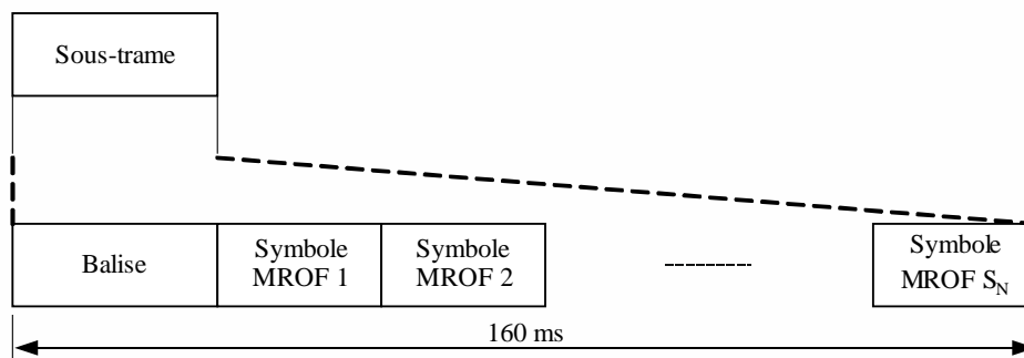
FIGURE 46 Structure d'une sous-trame
