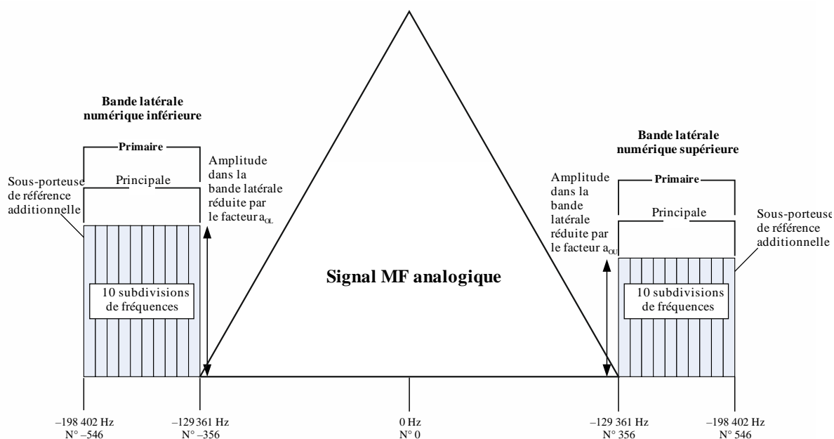
FIGURE 28 Spectre pour la forme d'onde hybride – Mode de service MP1
