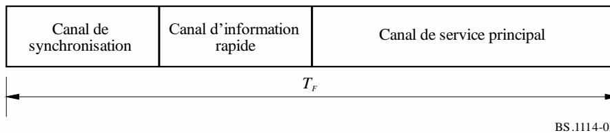
FIGURE 1 Structure de la trame du multiplex
