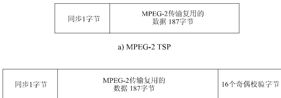
b) RS-TSP (传输TSP)，RS (204, 188) 差错防护TSP
