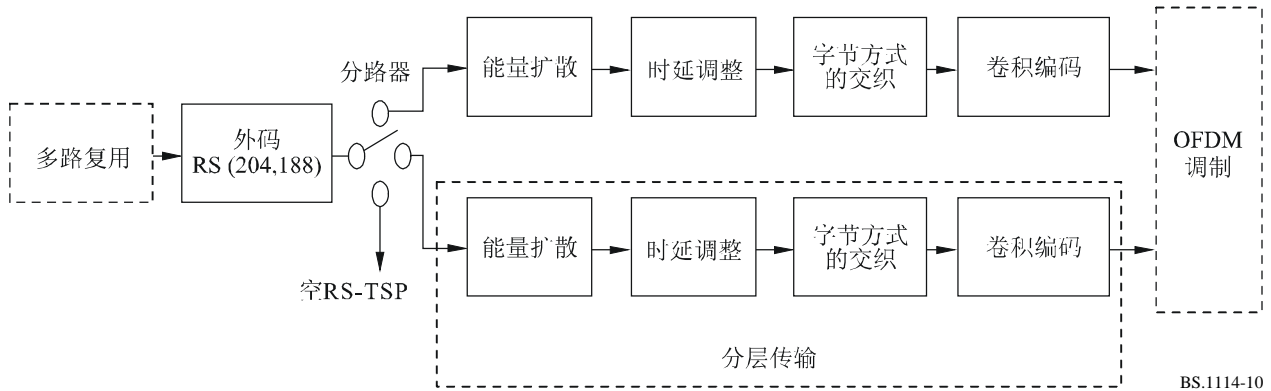
图10 信道编码图
