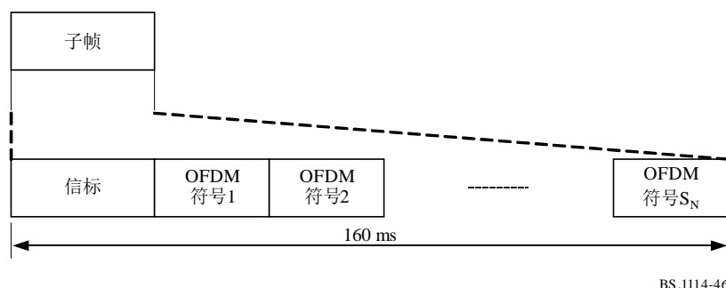
图46 子帧结构
