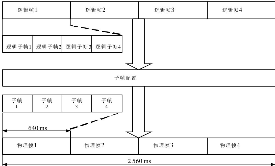
图44 逻辑帧和子帧配置
