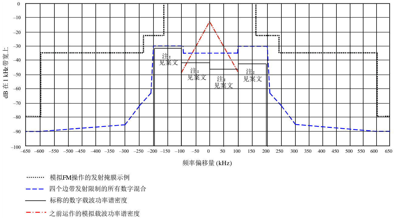
图32 全数字发射限制*
