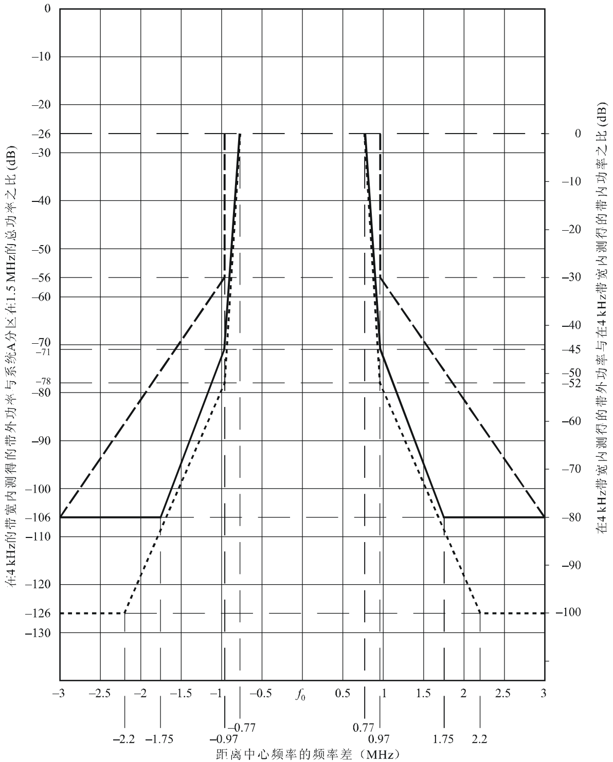
系统A传输信号的带外频谱掩模
