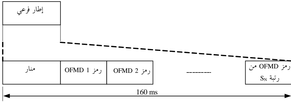
الشكل 46 هيكل إطار فرعي واحد
