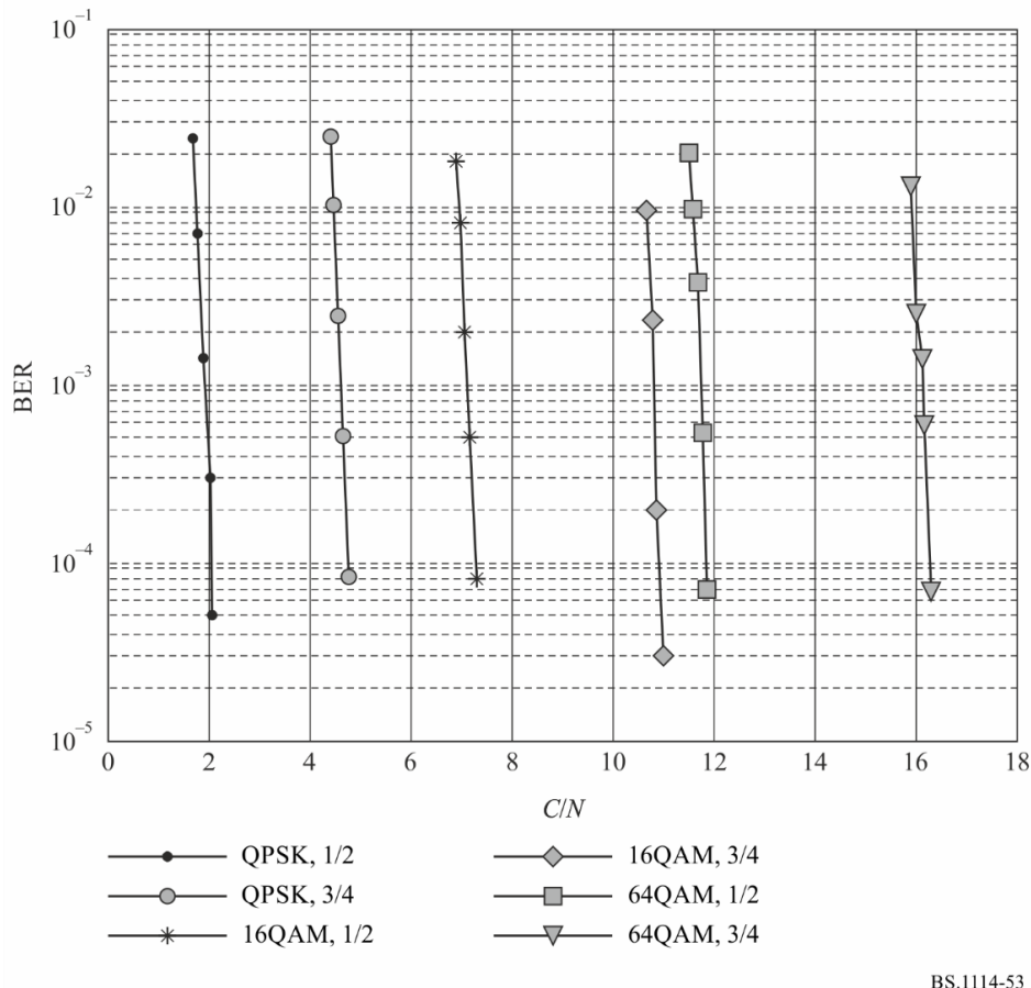
المعدل BER مقابل النسبة (C/N) في قناة غوسية
