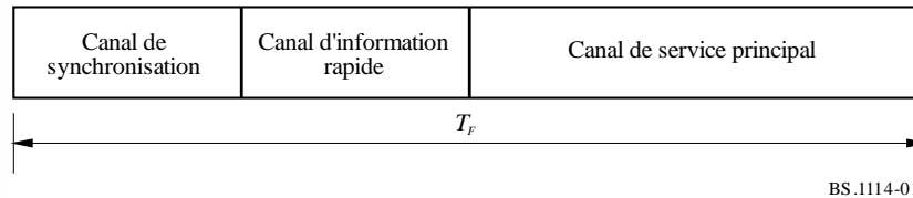
FIGURE 1 Structure de la trame du multiplex
