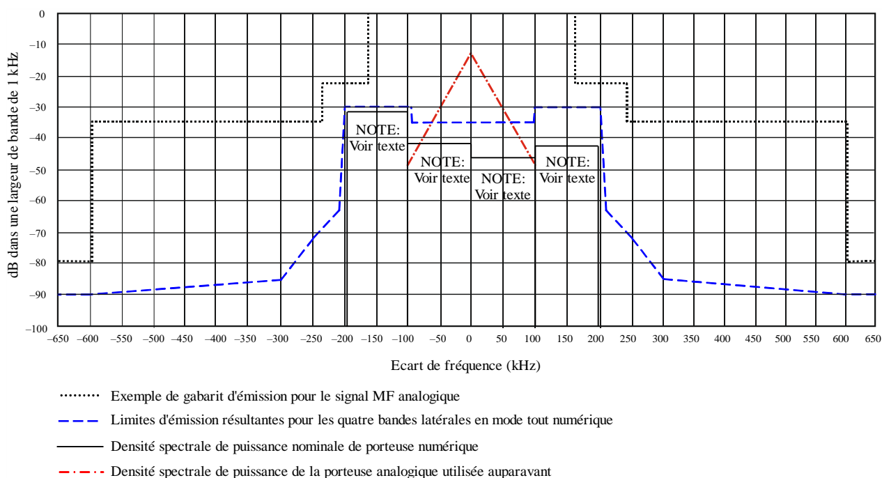
Limites d'émission en mode tout numérique
