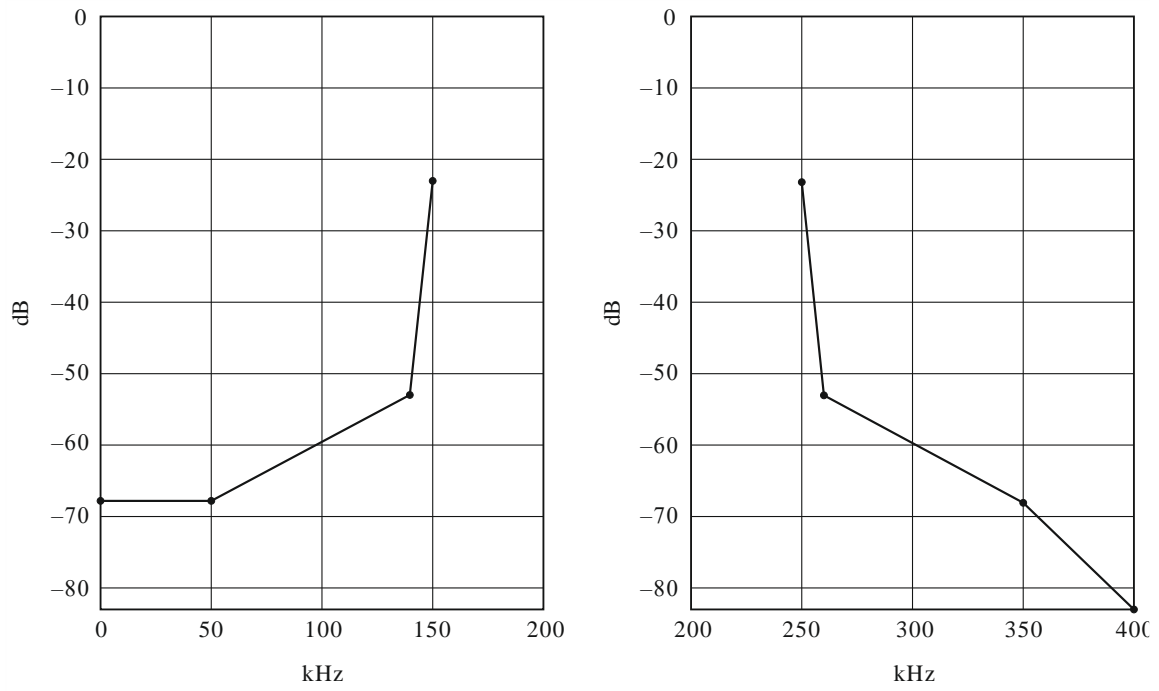
Gabarit spectral du mode d'occupation spectrale D
