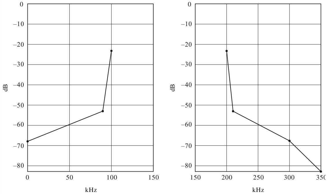
Gabarit spectral du mode d'occupation spectrale F
