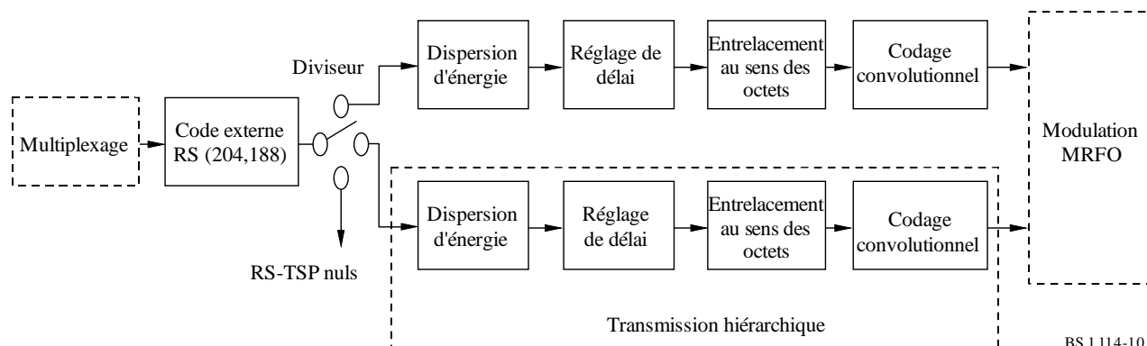
Diagramme de codage de canal
