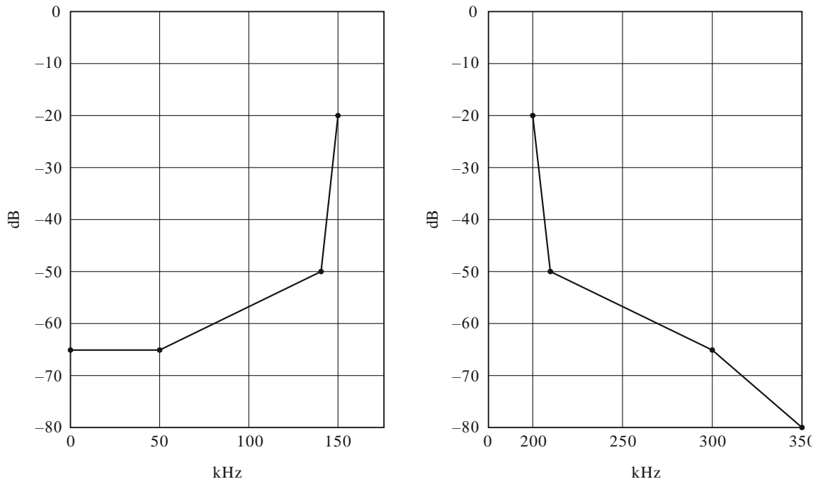
Gabarit spectral du mode d'occupation spectrale C
