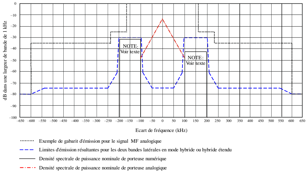
FIGURE 31 Limites d'émission en mode hybride IBOC
