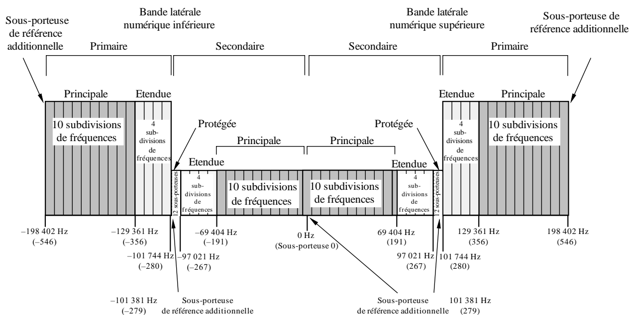
Spectre pour la forme d'onde tout numérique – Modes de service MP5, MP6 et MP12, MS1 à MS4
