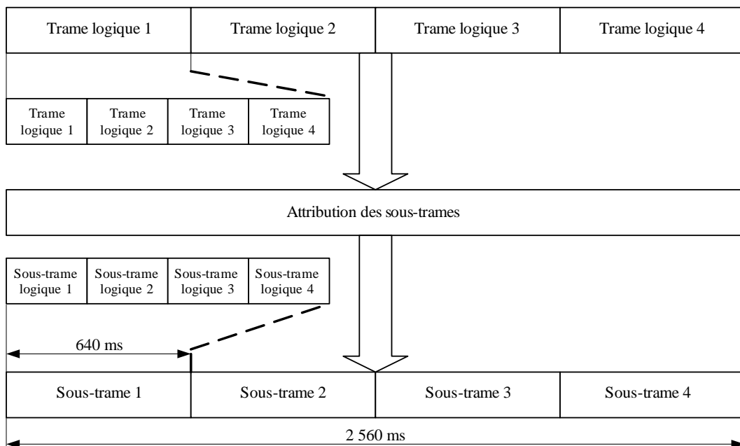
Trame logique et attribution des sous trames
