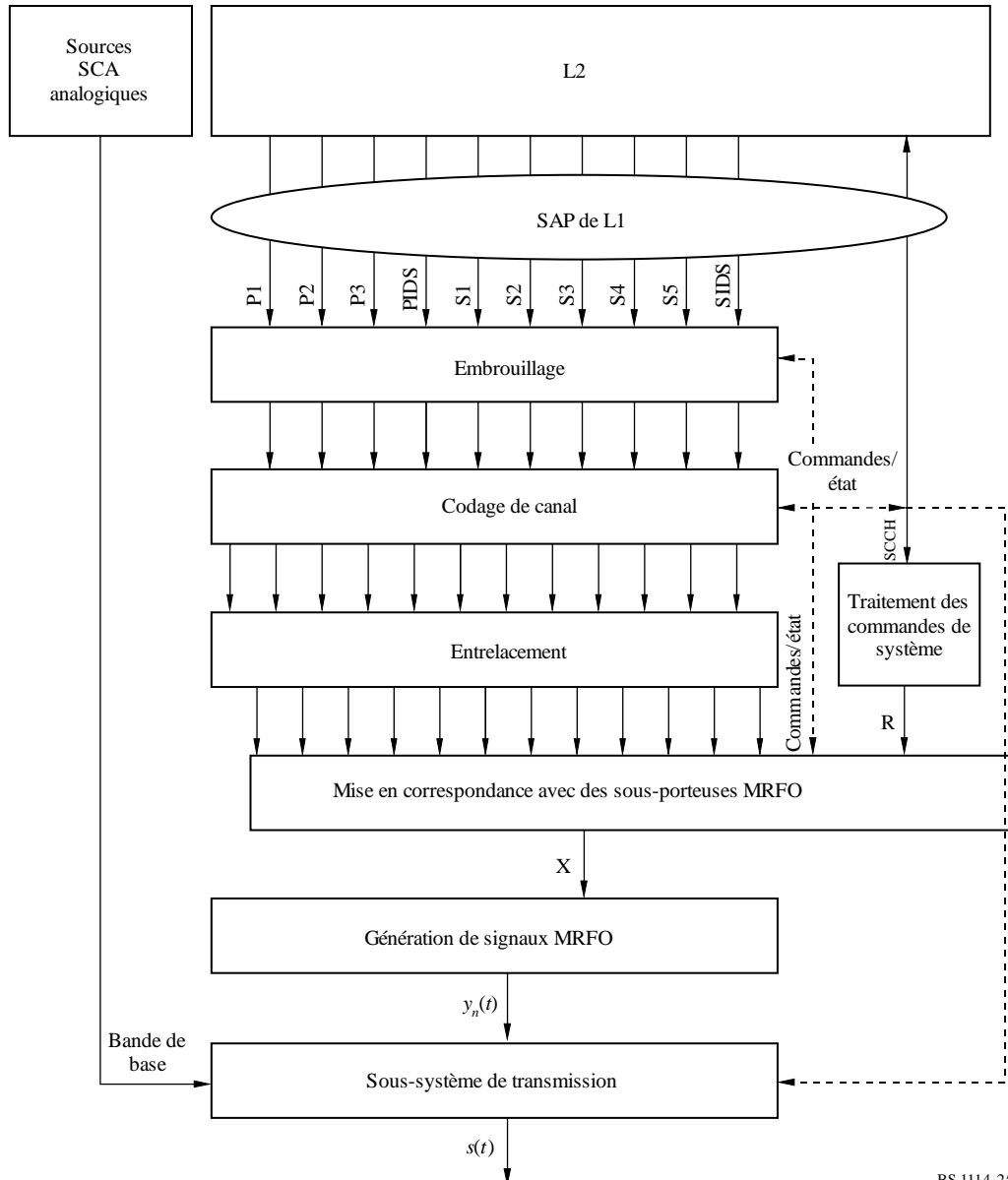
Schéma fonctionnel de L1 à l'interface radioélectrique MF
