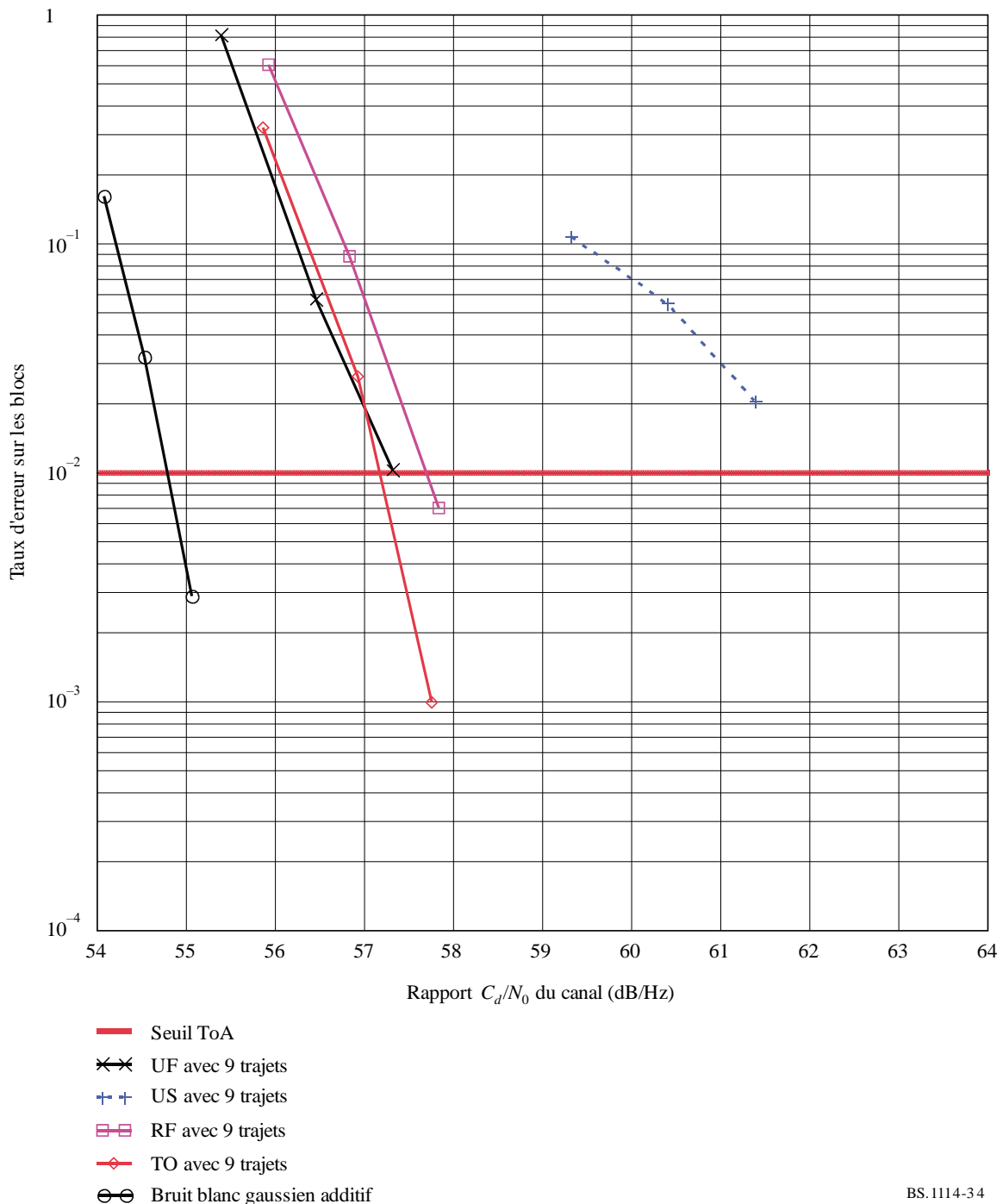
FIGURE 34 Taux d'erreur sur les blocs du système hybride pour différents types d'évanouissement sur 9 trajets et de bruit blanc gaussien additif
