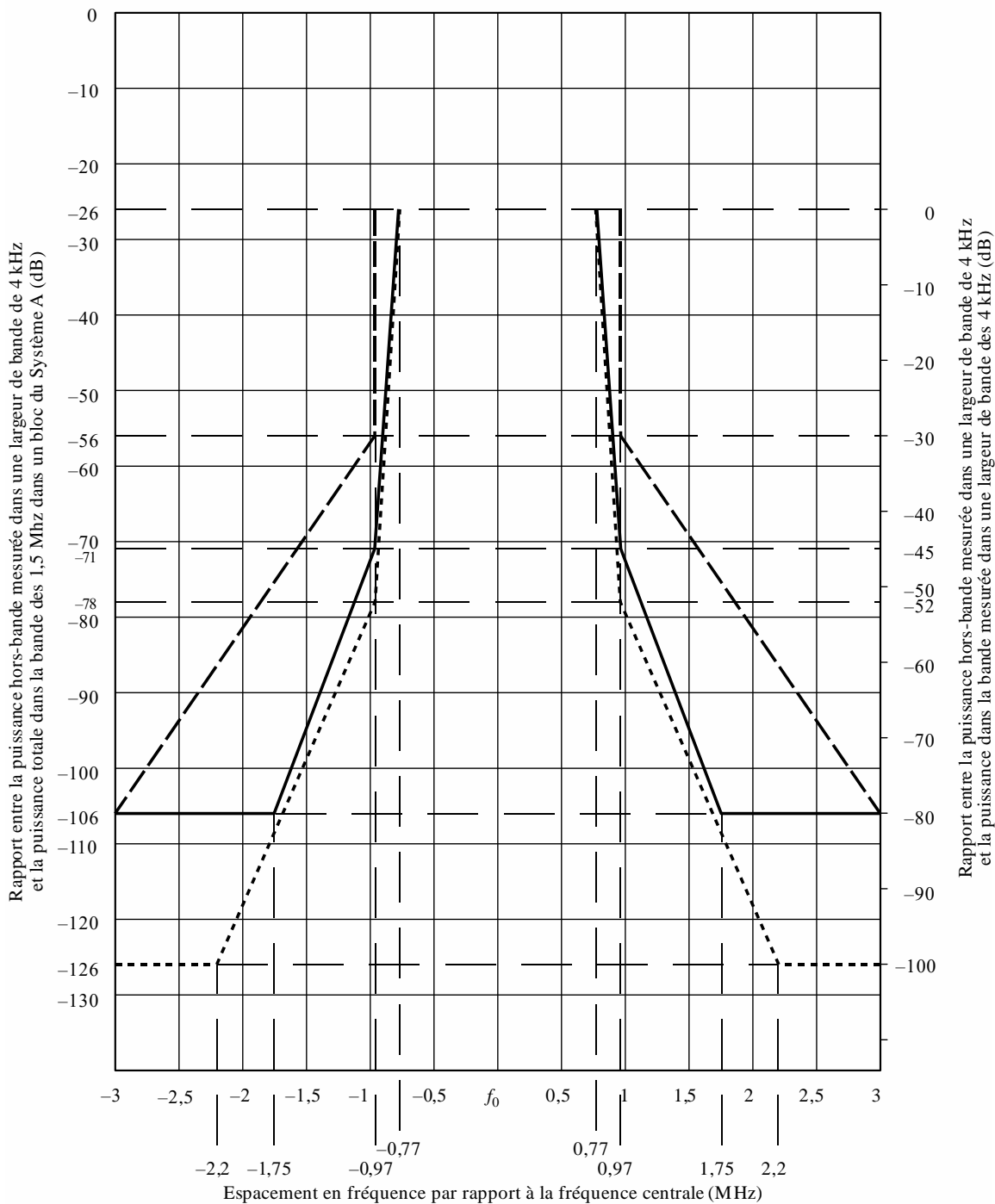
Gabarits du spectre hors bande pour un signal d'émission du Système A
