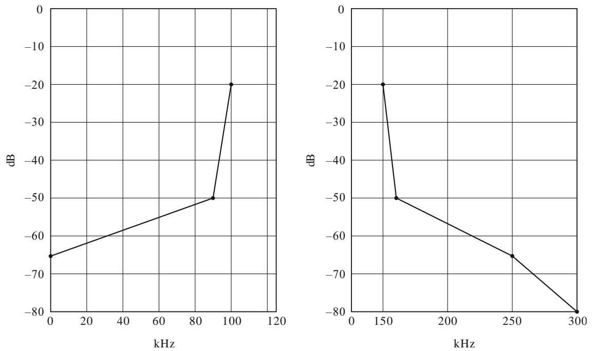
Gabarit spectral du mode d'occupation spectrale E
