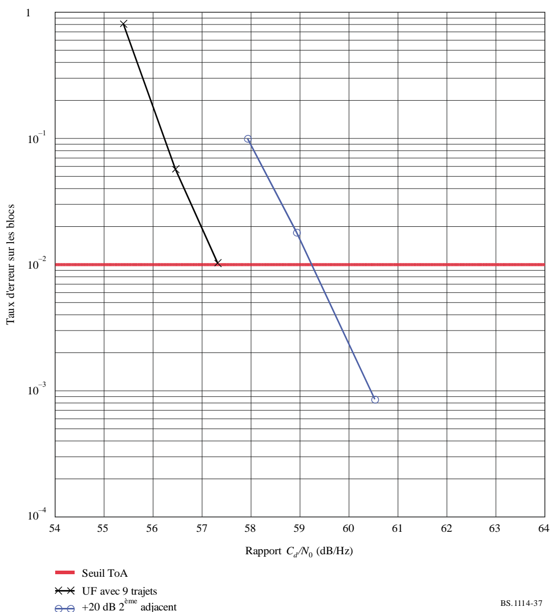
Taux d'erreur sur les blocs du système hybride avec brouilleur du deuxième canal adjacent à évanouissement individuel
