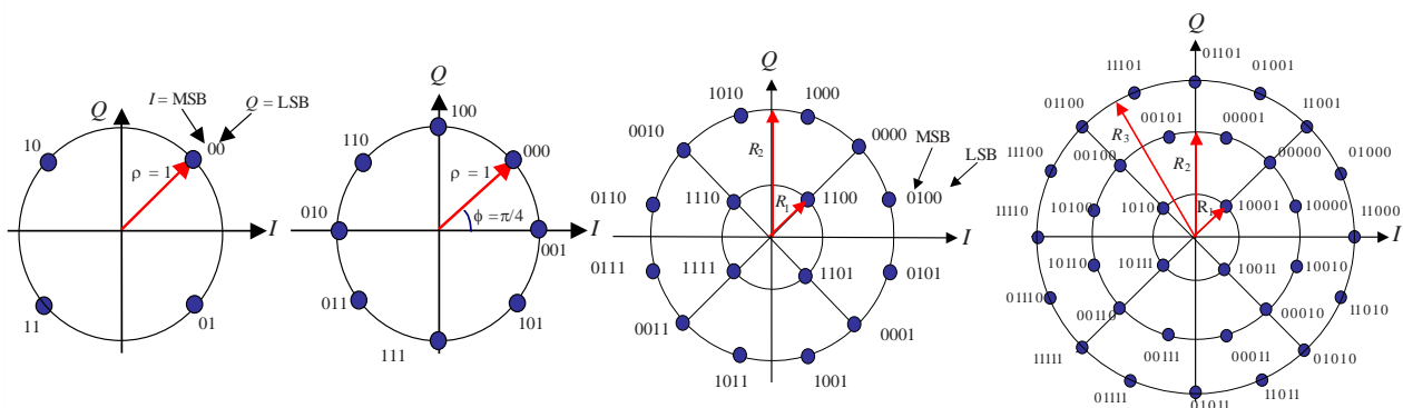
Les quatre constellations possibles pour le système DVB-S2 avant l'embrouillage dans la couche physique
