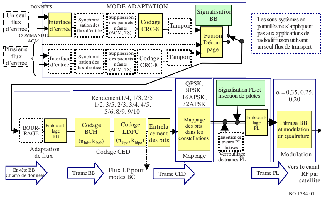
Diagramme des blocs fonctionnels du système DVB-S2
