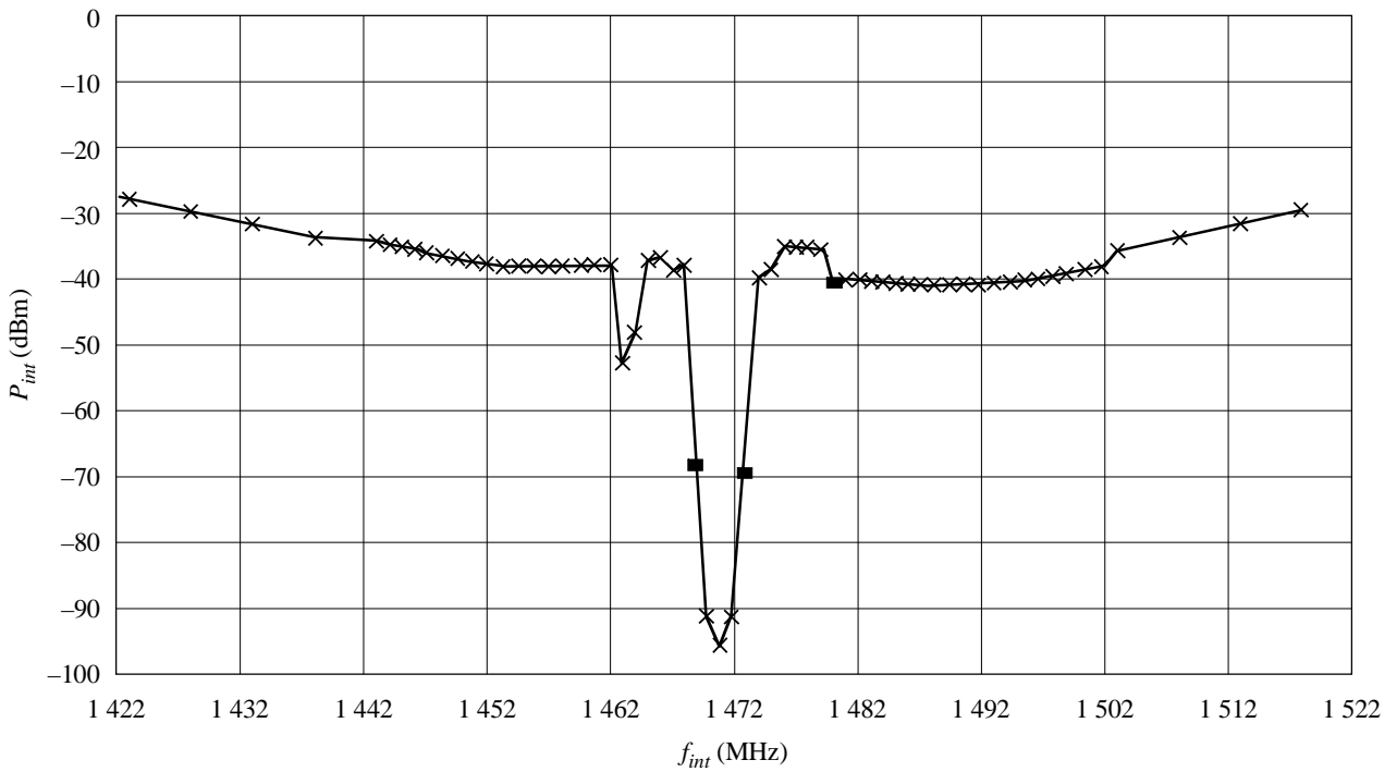
b) Señal interferente: sinusoidal; potencia de la señal: -90 dBm (entrada frontal)
