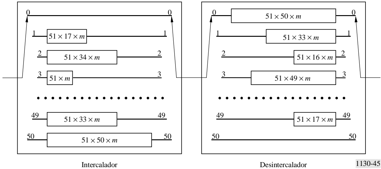
Diagrama conceptual de un intercalador y un desintercalador de bits
