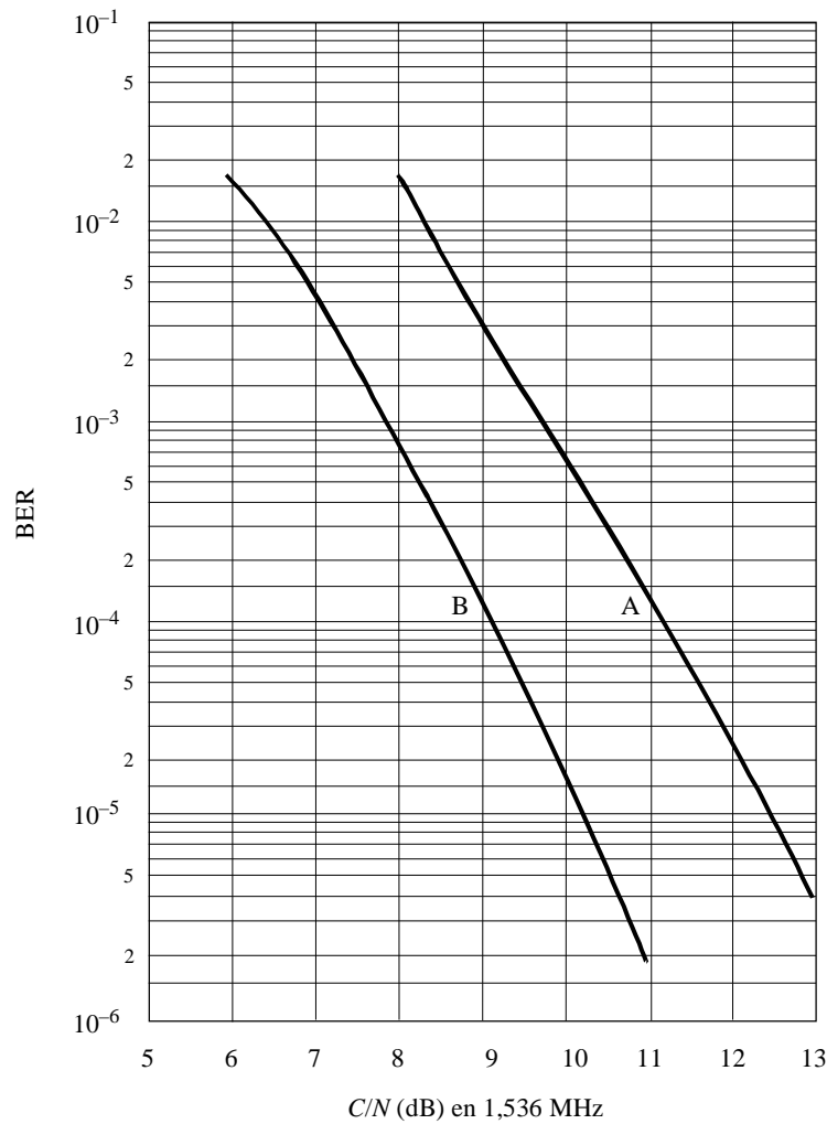
FIGURA 9 BER en función de C/N (en 1,5 MHz) en un canal de Rayleigh, 1 500 MHz, Modo II
