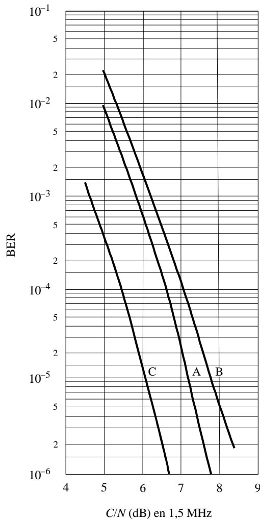
FIGURA 7 BER en función de C/N (en 1,5 MHz) en un canal gaussiano, 226 MHz, Modo I
