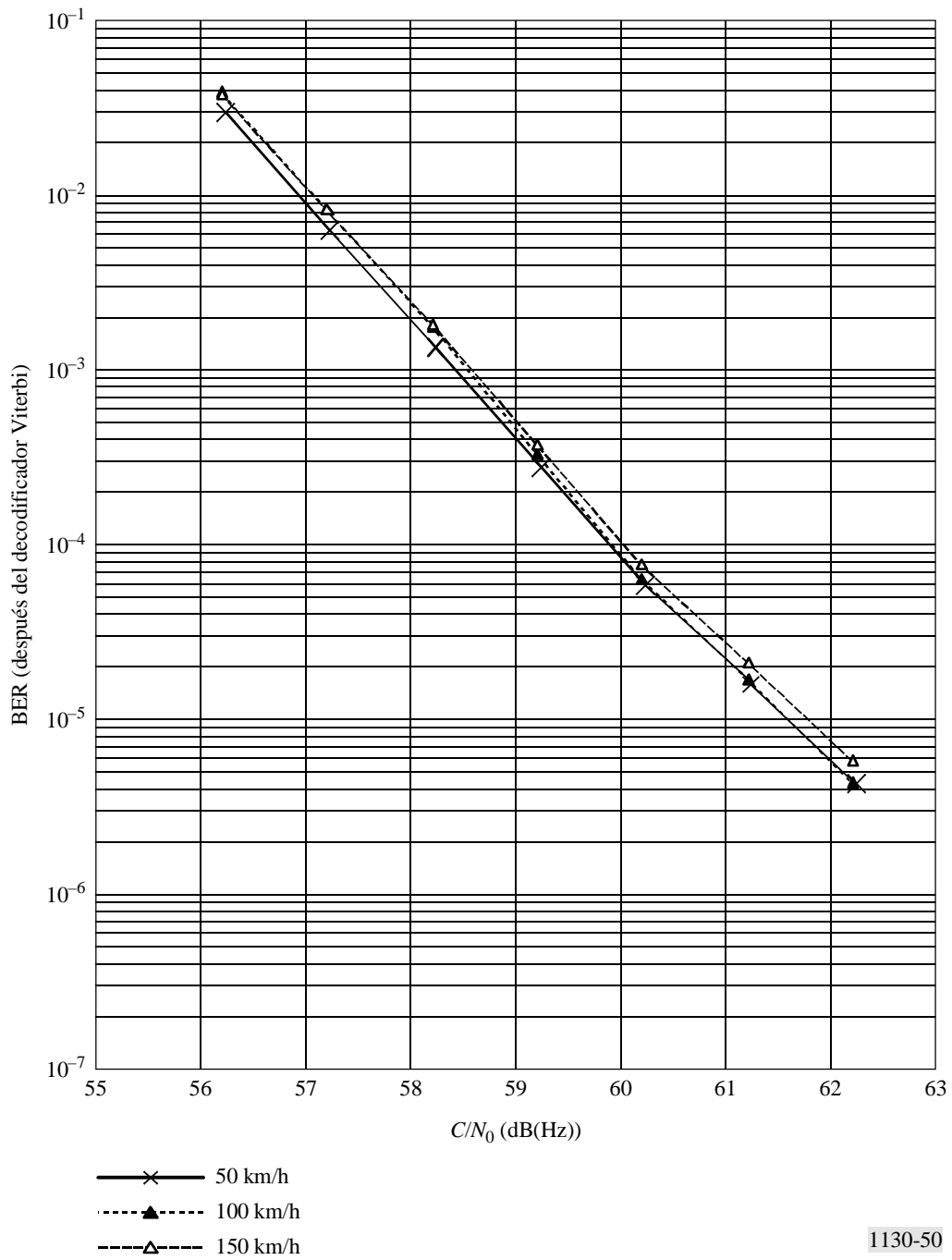
FIGURA 50 BER en función de C/N_0 para recepción de alta velocidad (50 km/h, 100 km/h y 150 km/h)
