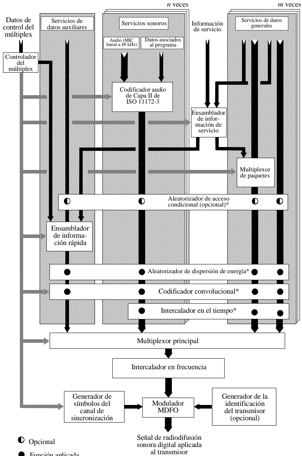
Diagrama conceptual de la parte de transmisión del Sistema
