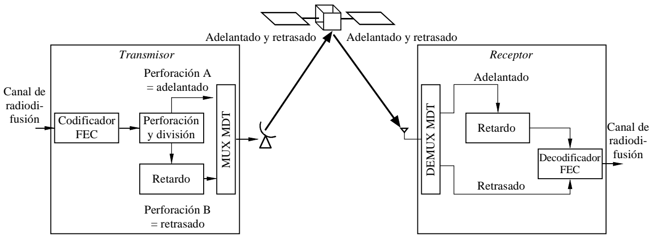
FIGURA 28 Diversidad en el tiempo con un solo satélite
