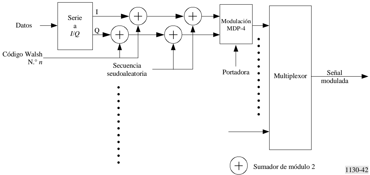
Diagrama de bloque detallado de MDC
