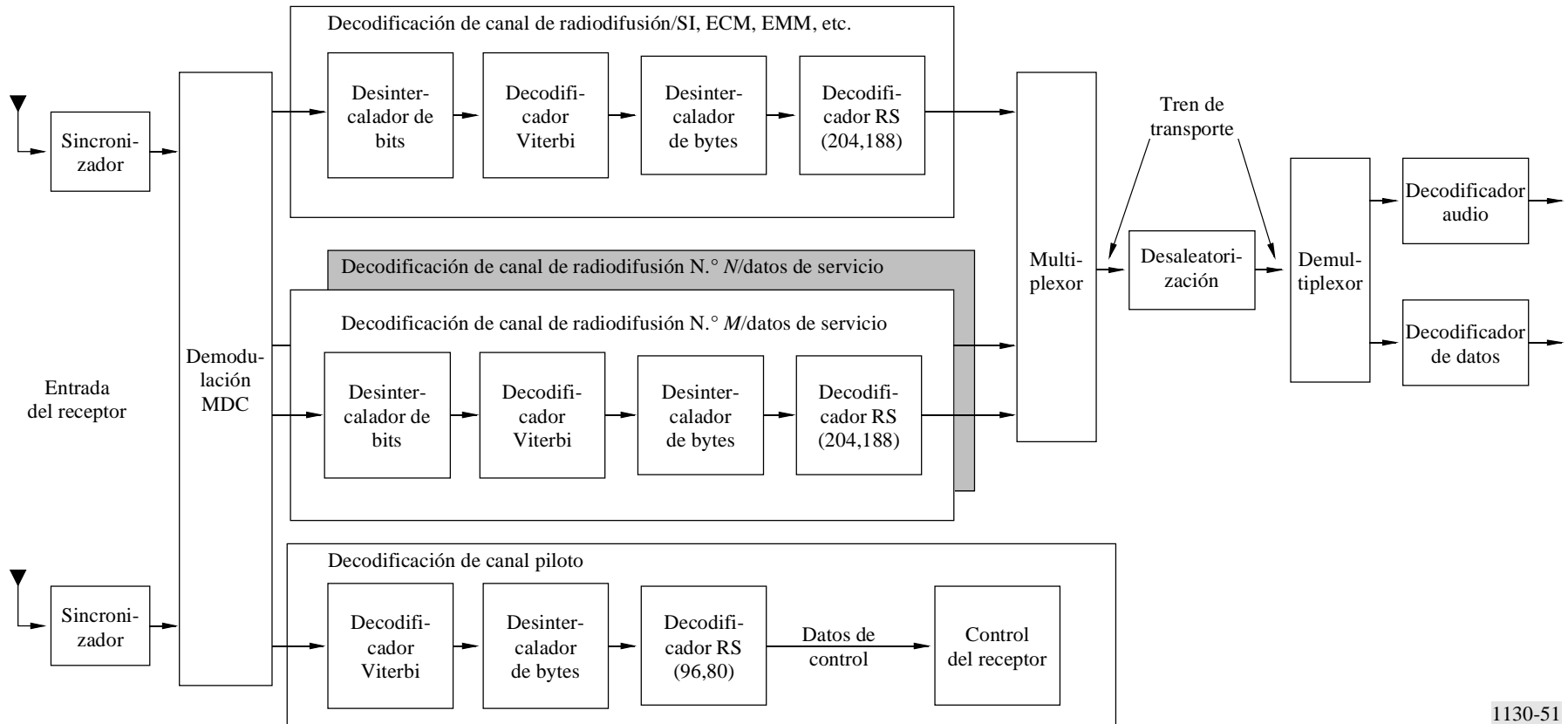
FIGURA 51 Diagrama de bloques de un receptor típico
