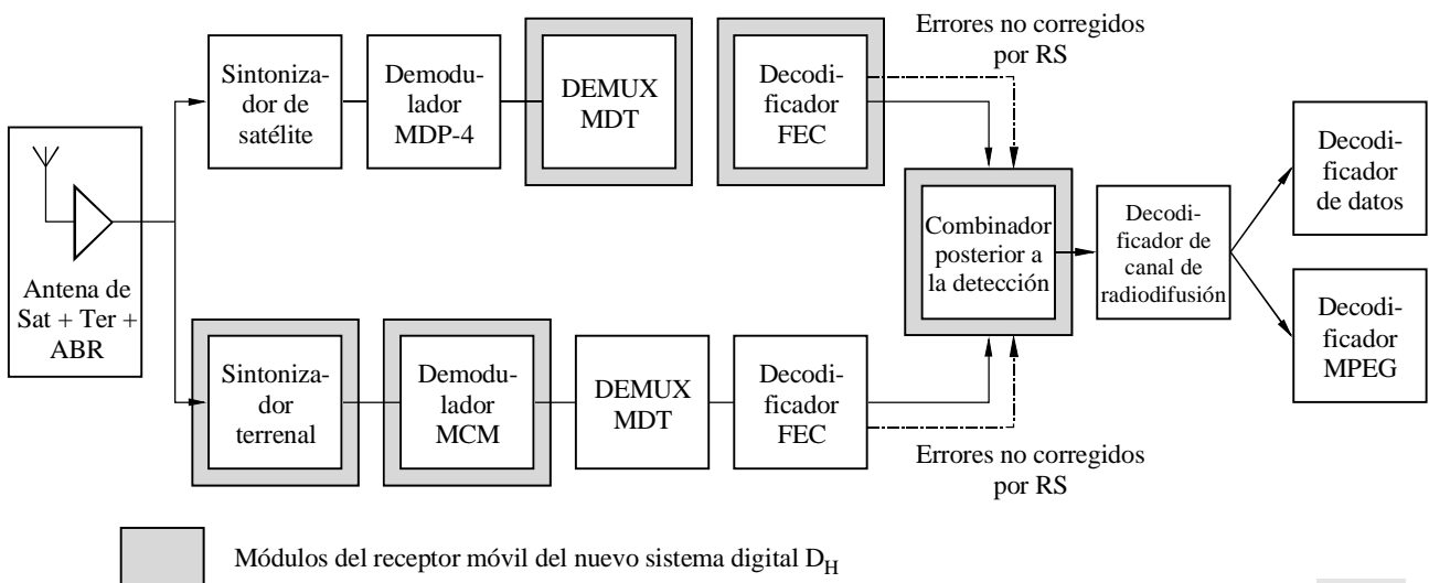
FIGURA 38 Receptor de diversidad en el tiempo solamente
