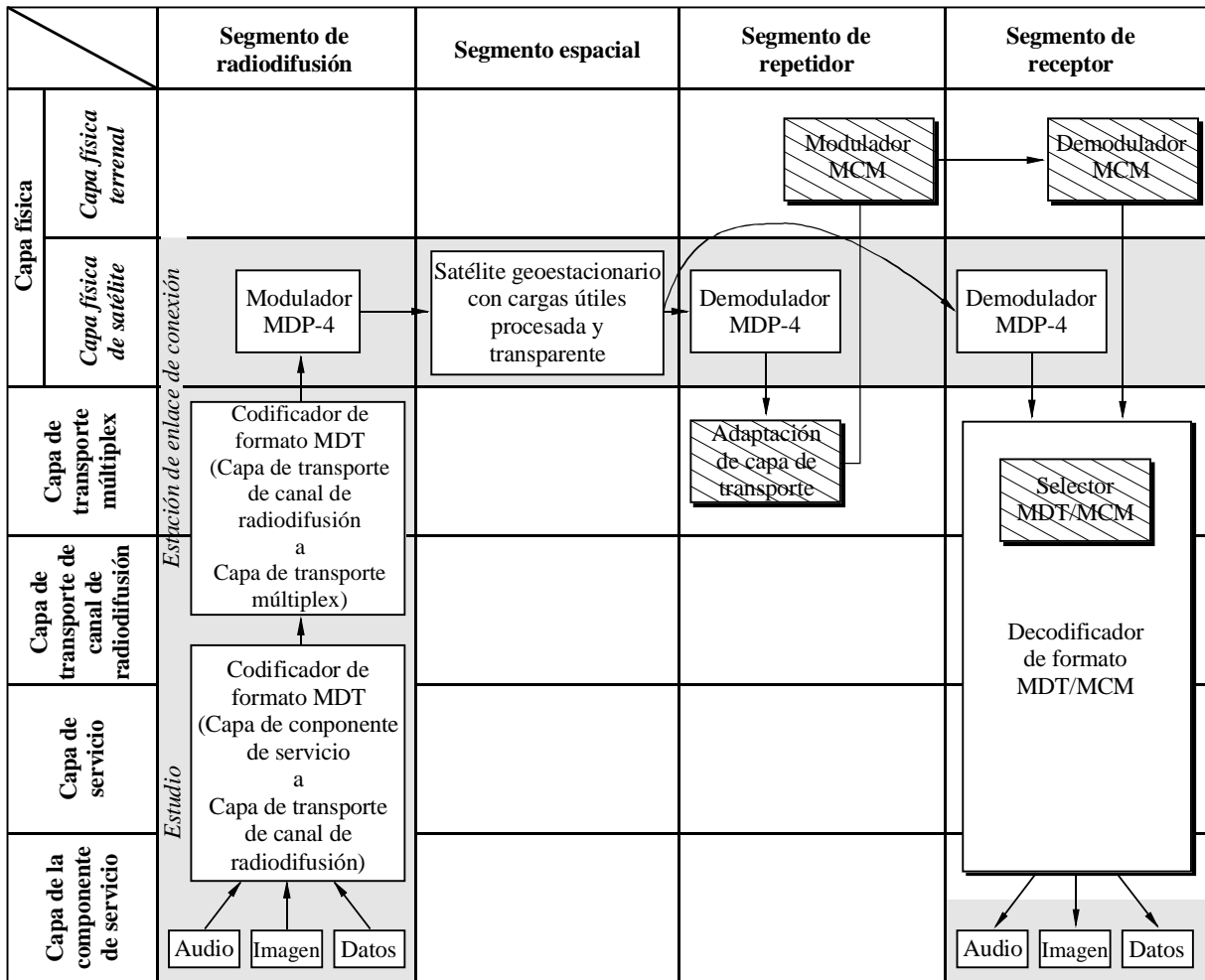
Capas de la señal del Sistema digital D_H de WorldSpace con la ampliación MCM
