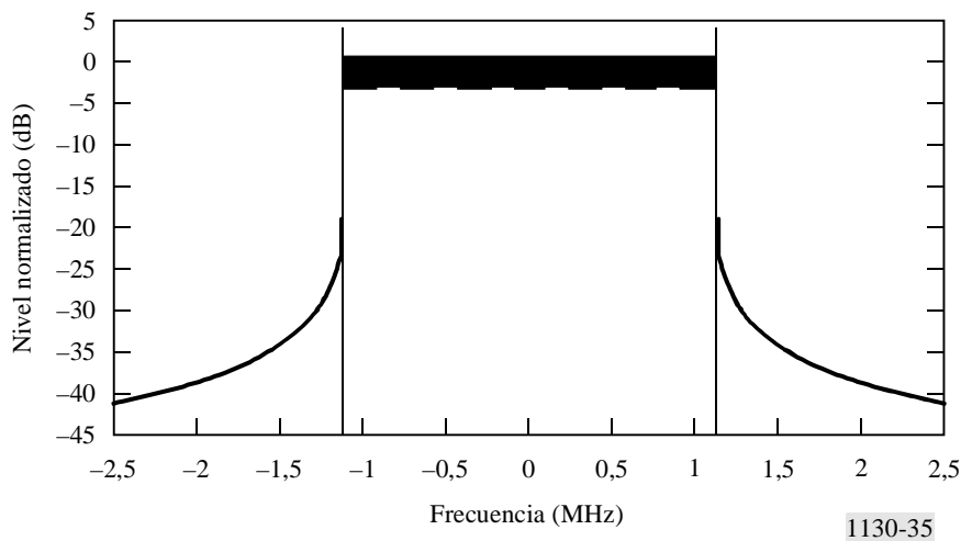
FIGURA 35 Espectro teórico de MCM
