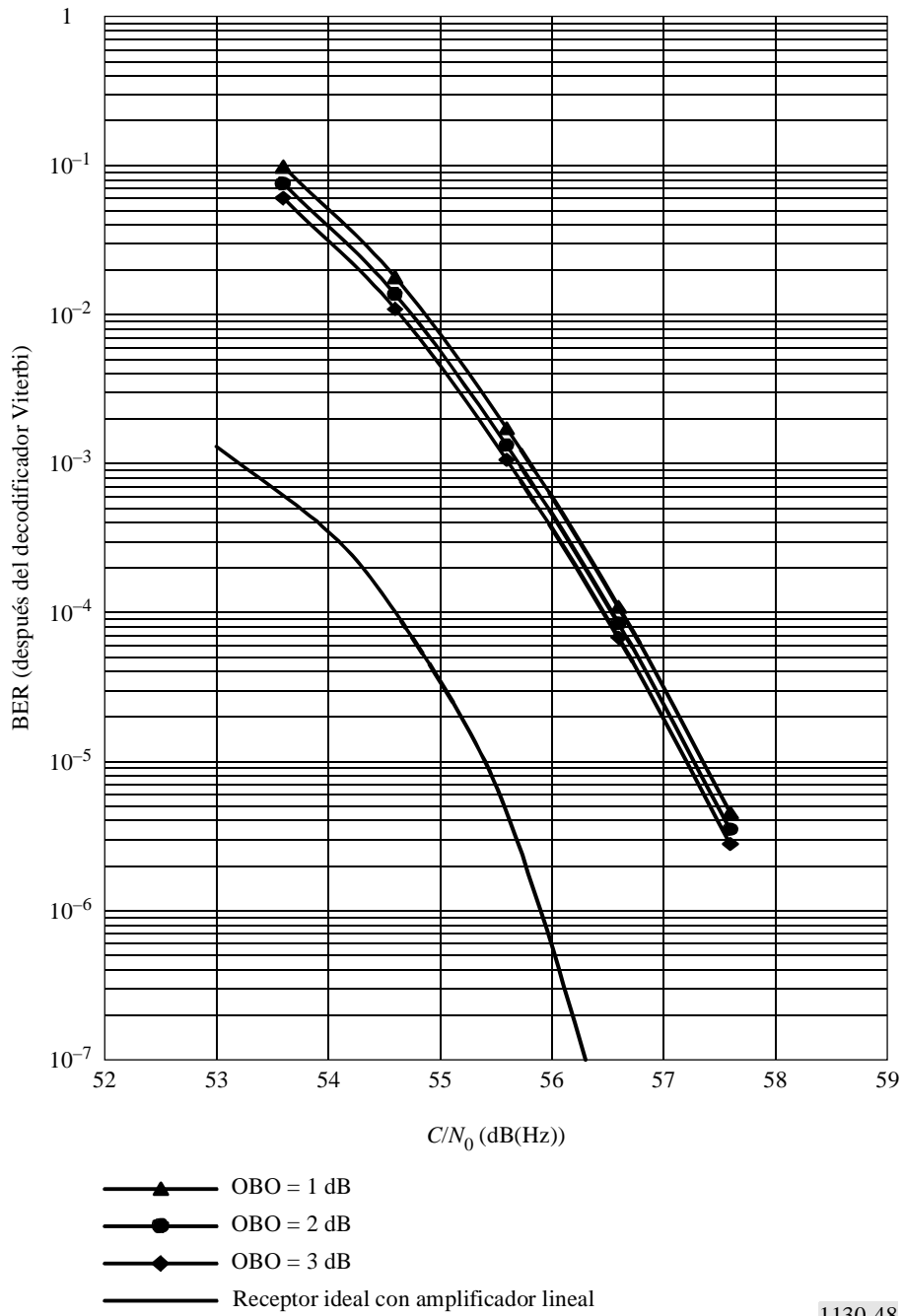
FIGURA 48 BER en función de C/N_0 en un entorno AWGN para diferentes niveles de OBO del transpondedor
