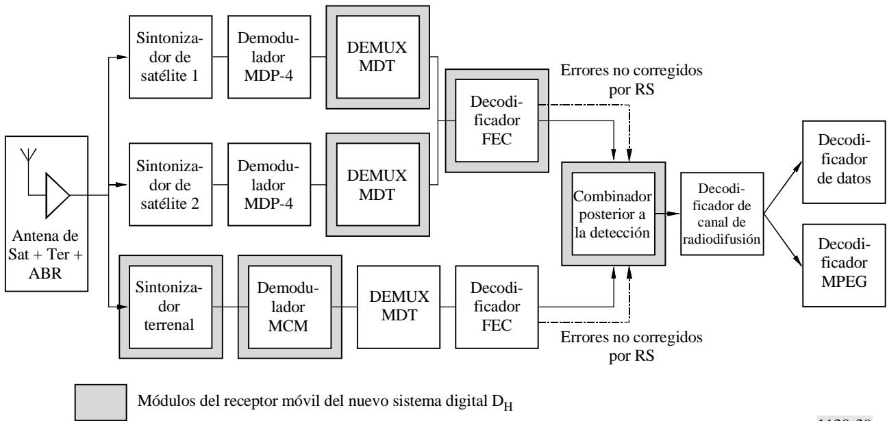
Receptor de diversidad en el tiempo y espacial
