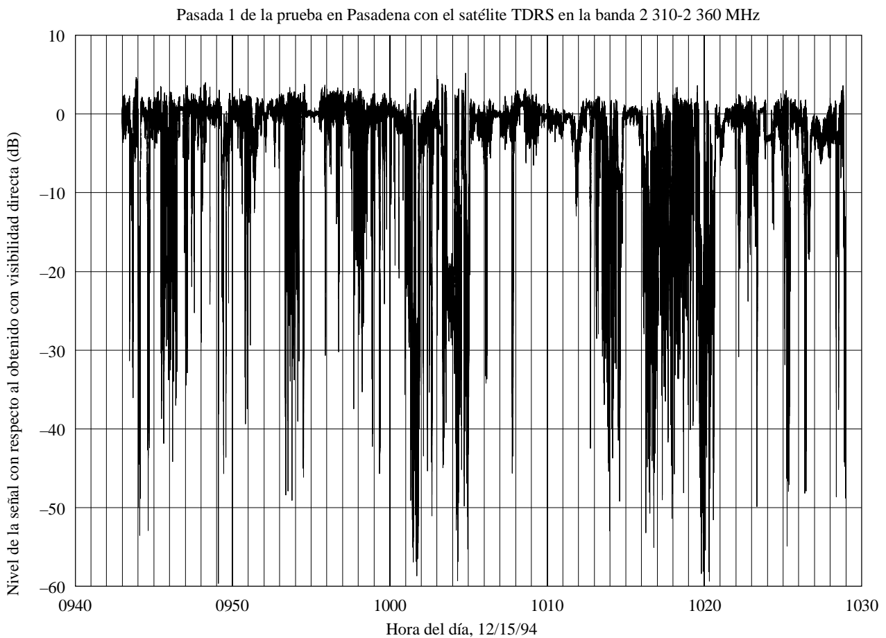
FIGURA 14 Modelo de canal de satélite
