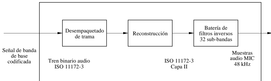
Diagrama de bloques del decodificador audio básico del Sistema
