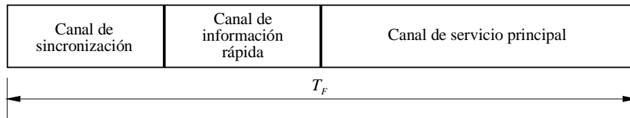
Estructura de la trama múltiplex
