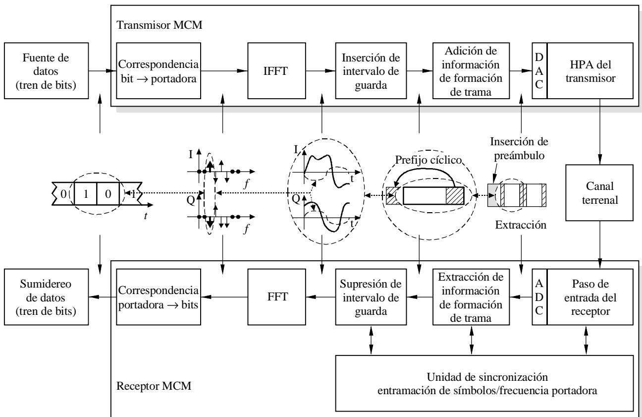
FIGURA 32 Conversión de MDT a MCM
