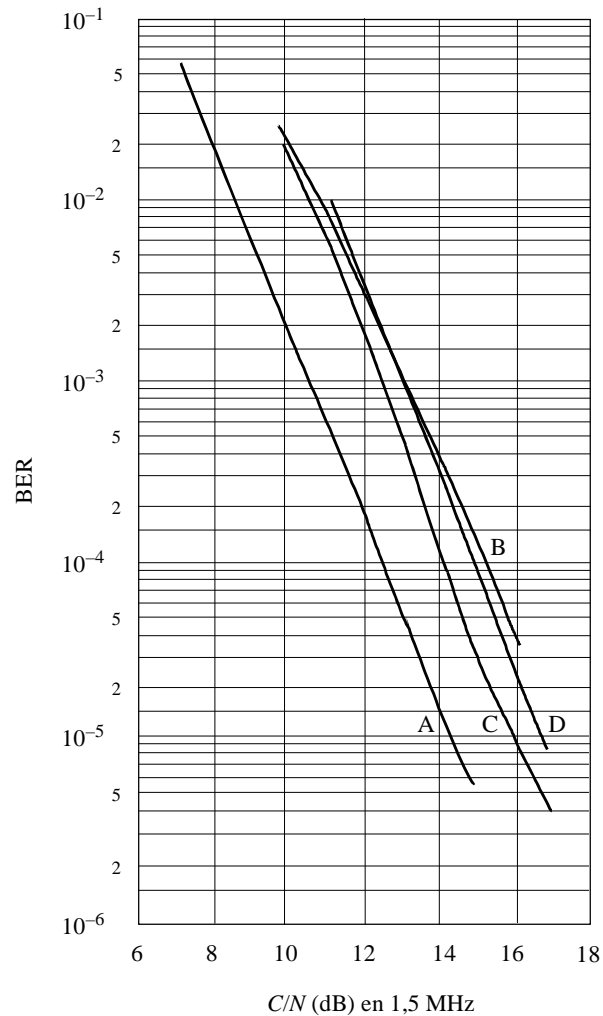
FIGURA 8 BER en función de C/N (en 1,5 MHz) en un canal de Rayleigh 226 MHz, Modo I
