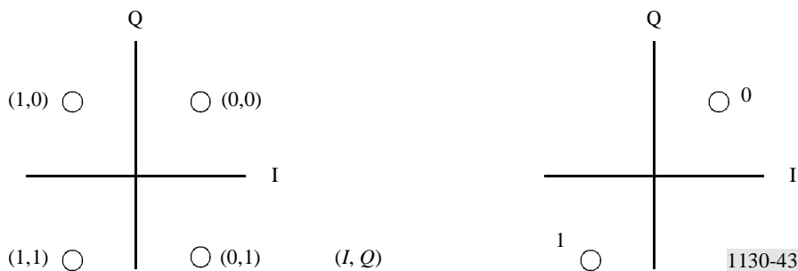
Correspondencias de símbolos de modulación MDP-4 y MDP-2
