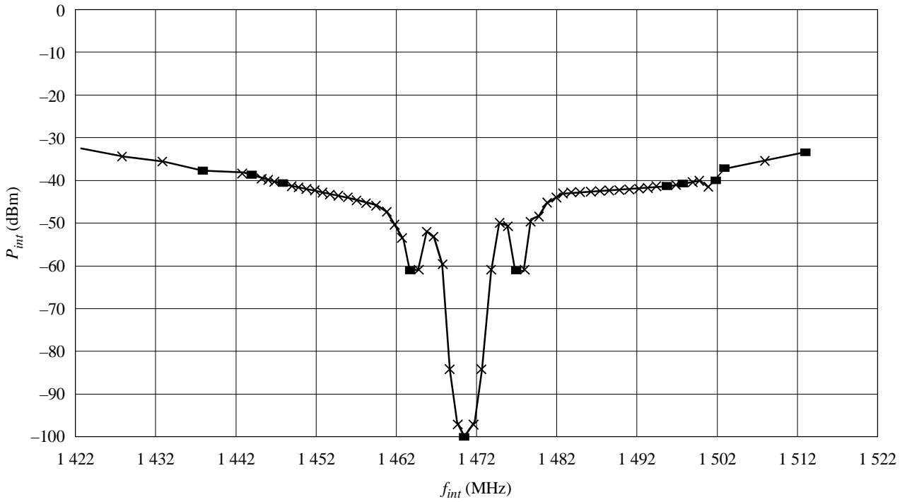
a) Señal interferente: MDP-4; potencia de la señal: -90 dBm (entrada frontal)
