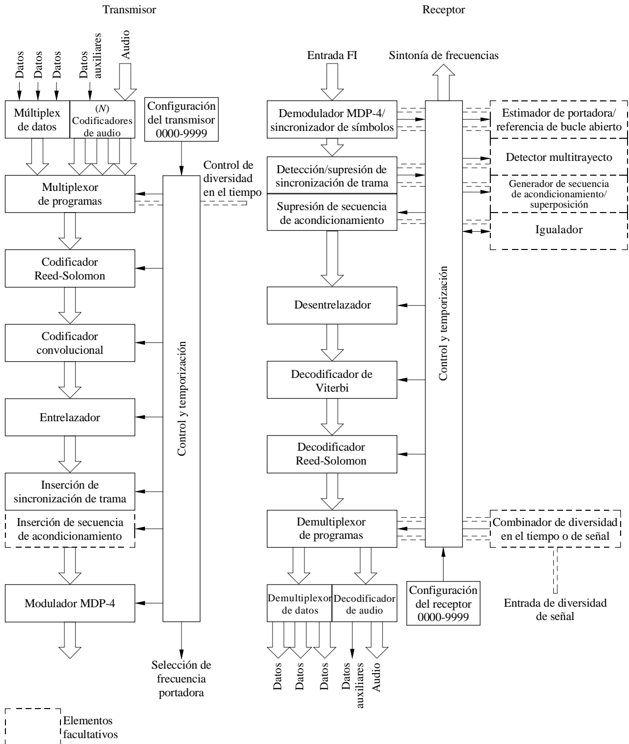
FIGURA 11 Diagrama de bloques del Sistema B
