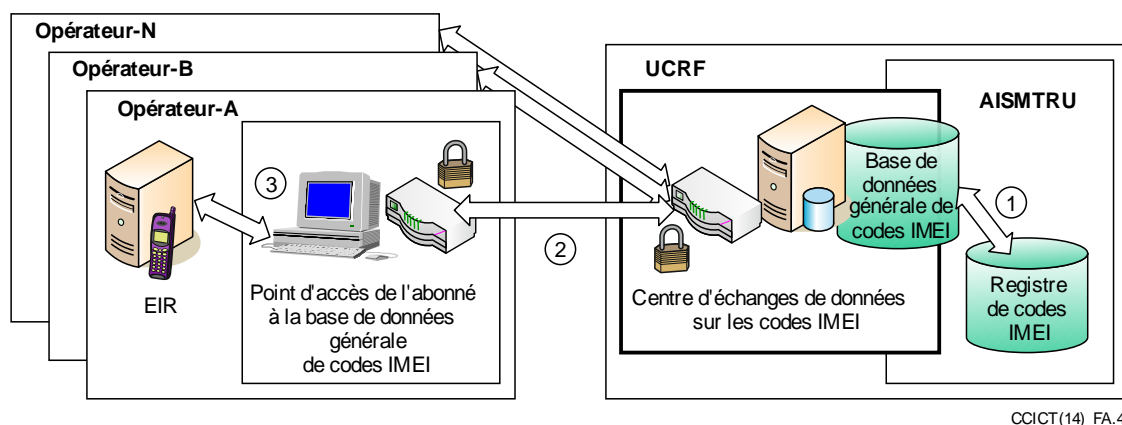
Figure A.4 – Registre EIR et base de données générale de codes IMEI
