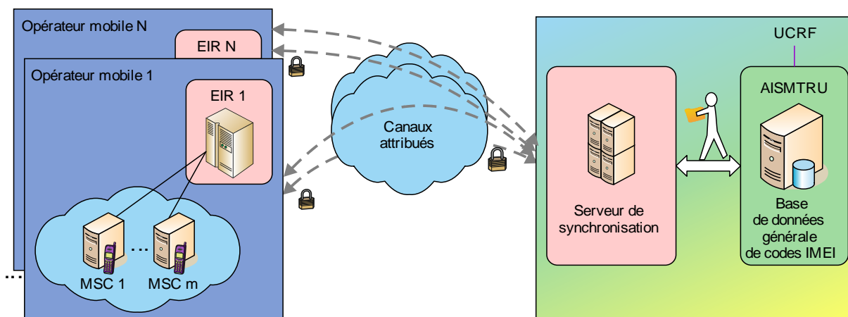
Figure A.5 – Serveur de synchronisation
