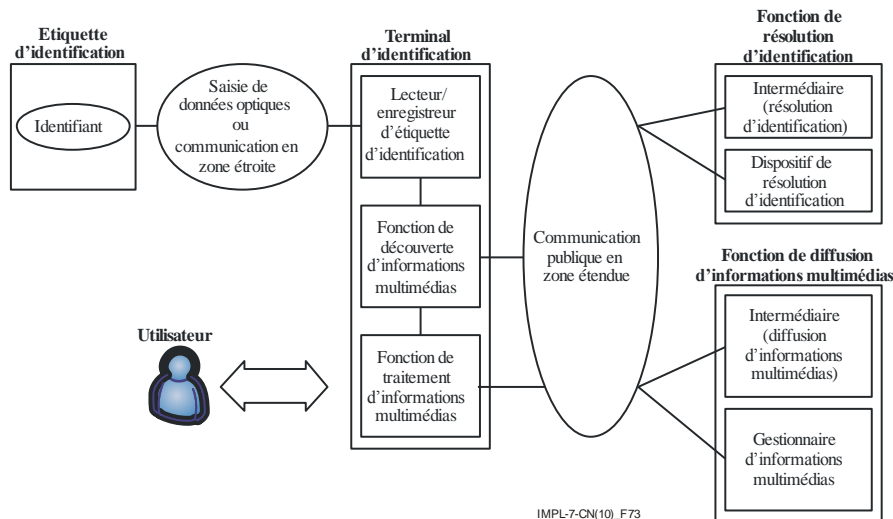
Figure 6 – Architecture fonctionnelle pour l'accès à des informations multimédias déclenché par une identification basée sur une étiquette (Recommandation UIT-T H.621)
