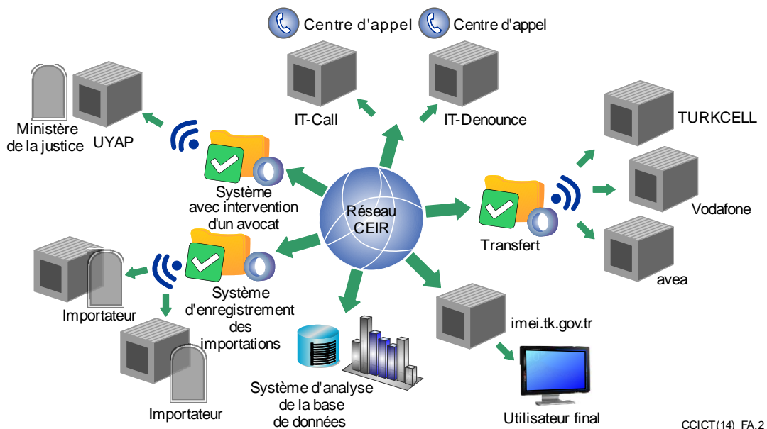
Figure A.2 – Structure du Registre central d'identités d'équipements
