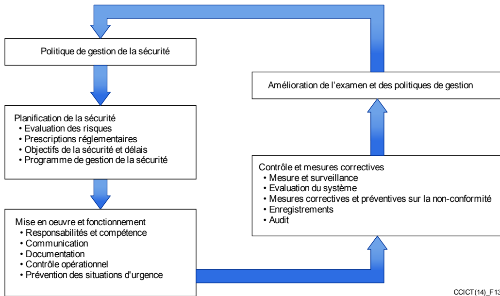
Figure 13 – Eléments du système de gestion de la sécurité ISO 28000
