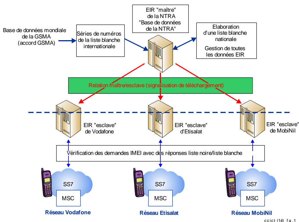
Figure A.1 – Solution de base de données centrale EIR IMEI en Egypte
