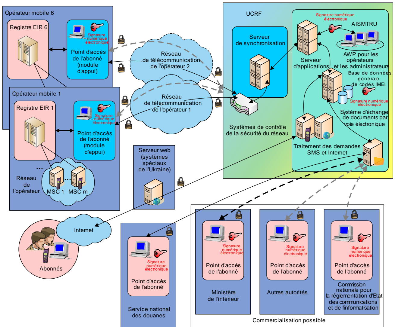
Figure A.6 – Système global de protection des informations (CIPS) de l'AIMS TRU
