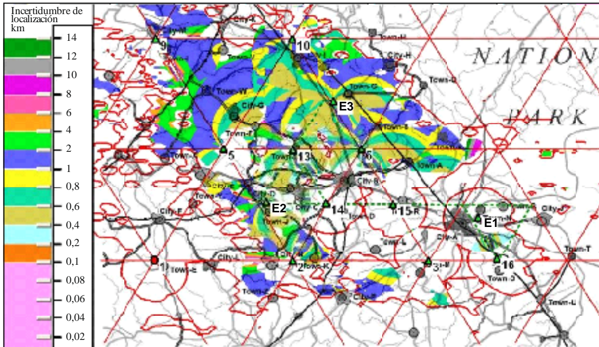
FIGURA 13 Plantilla de cobertura de localización de la SMN más densa para transmisores de prueba de categoría I
