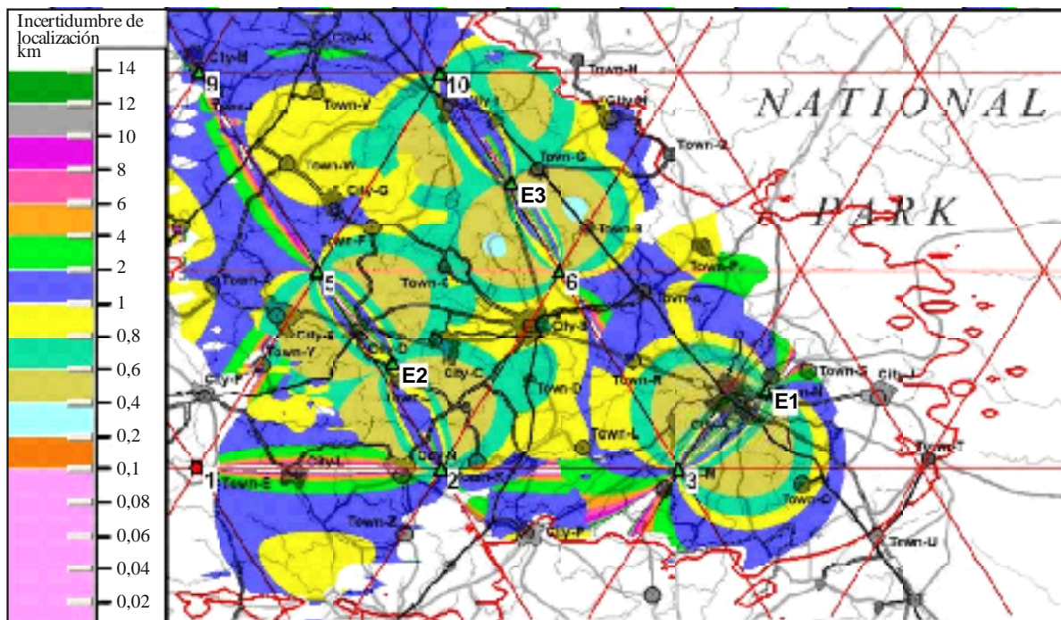
FIGURA 8 Plantilla de cobertura de localización de la red primaria (sin las estaciones 4, 7 y 11) para transmisores de prueba de categoría II
