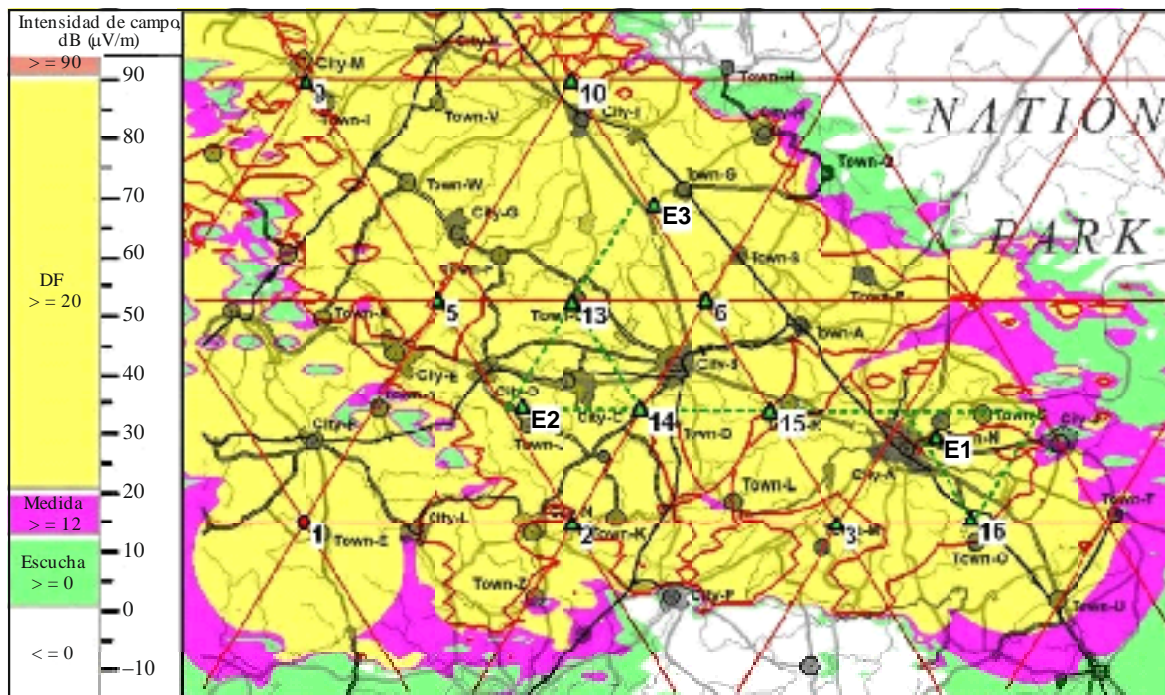
FIGURA 14 Cobertura de comprobación técnica de la SMN más densa para transmisores de 10 W con altura de antena de 5 m
