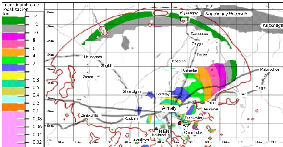
FIGURA A2-3 Cobertura de radiogoniometría y localización con un emplazamiento inadecuado de la estación BUT
