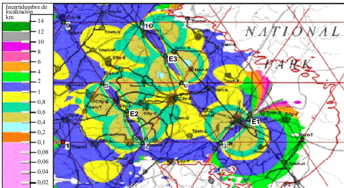
FIGURA 9 Plantilla de cobertura de localización de la red primaria (sin las estaciones 4, 7 y 11) para transmisores de prueba de categoría III
