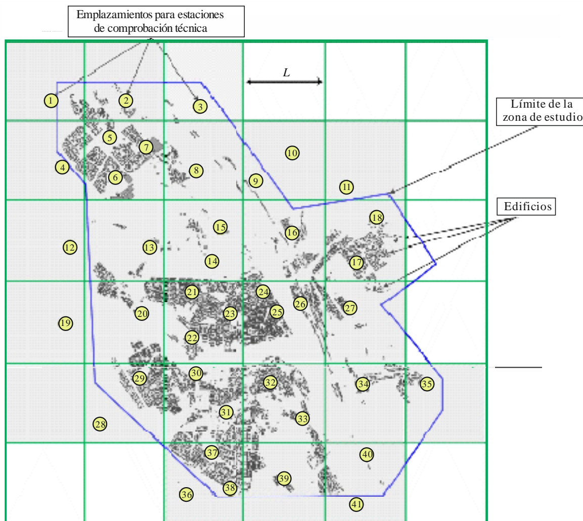
FIGURA 18 Selección de posibles emplazamientos para las estaciones de comprobación técnica
