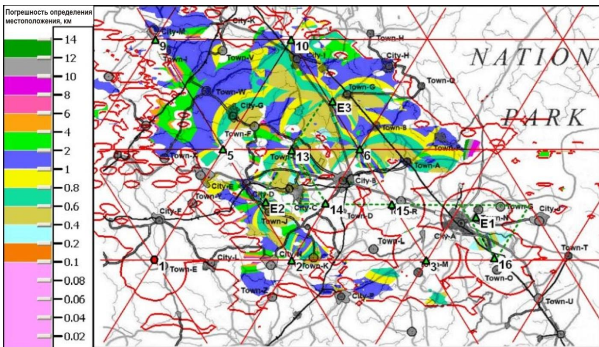
Шаблон охвата функцией определения местоположения в более плотной сети SMN при использовании испытательных передатчиков категории I
