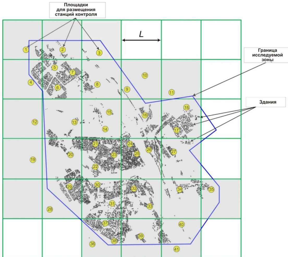
Выбор возможных площадок для размещения станций радиоконтроля
