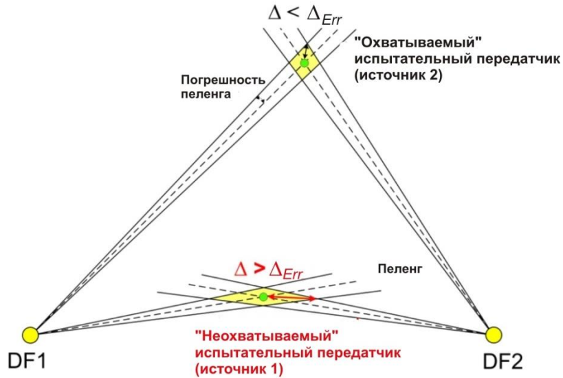
Пример определения зоны охвата двумя станциями АОА
