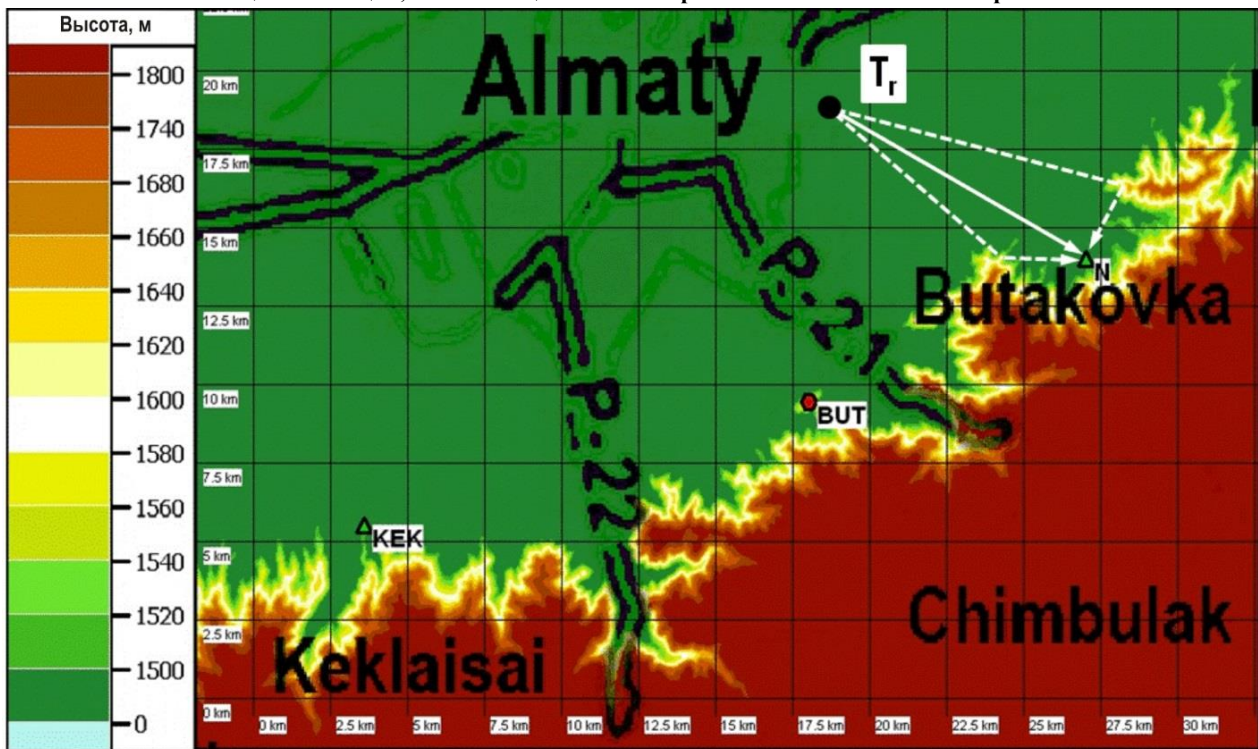
РИСУНОК А2-4 Размещение станций, позволяющее снизить вероятность возникновения отражений
