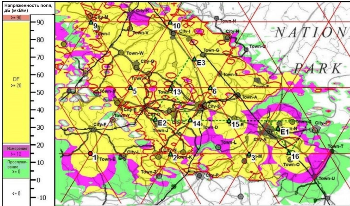
Охват услугами контроля в более плотной сети SMN при использовании испытательных передатчиков категории I
