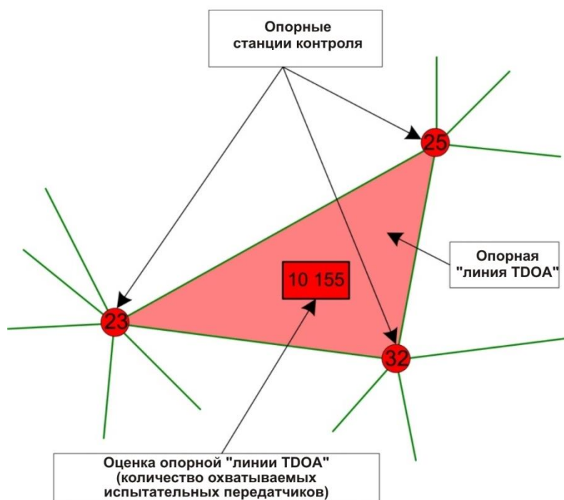
РИСУНОК 24 Часть схемы "линий TDOA"
