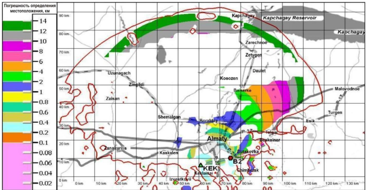
РИСУНОК А2-3 Зоны охвата функциями радиопеленгации и определения местоположения при неправильном размещении станции BUT
