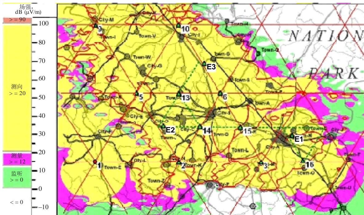
有关10 W测试发射机（天线高度5 m）的密集SMN的监测覆盖范围
