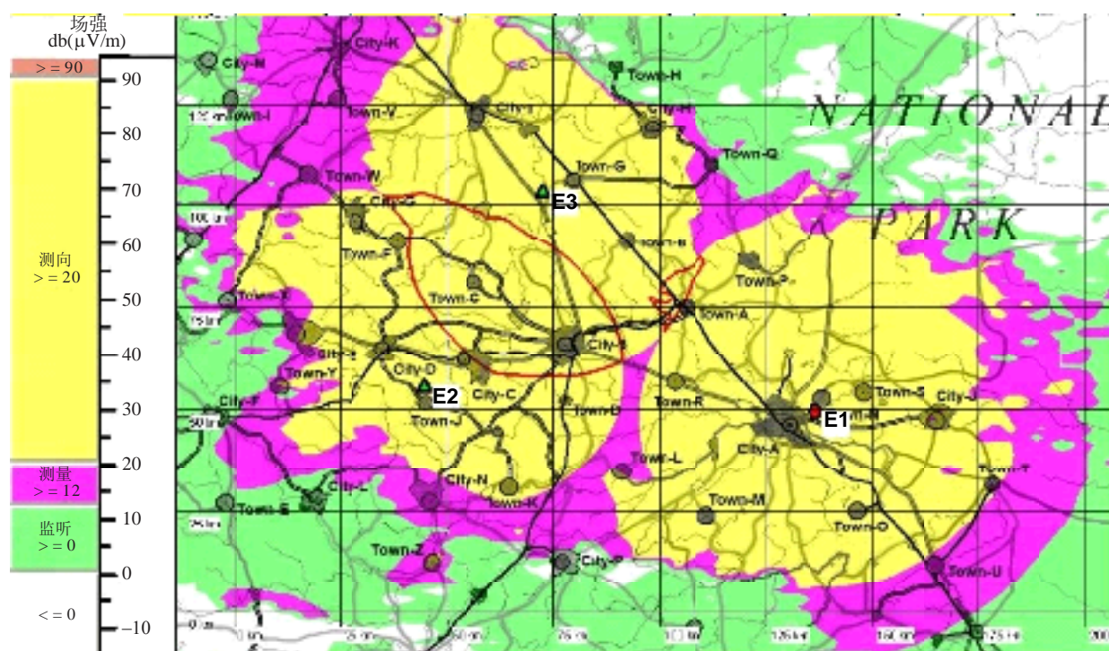
现有三个站总的监测覆盖区域
