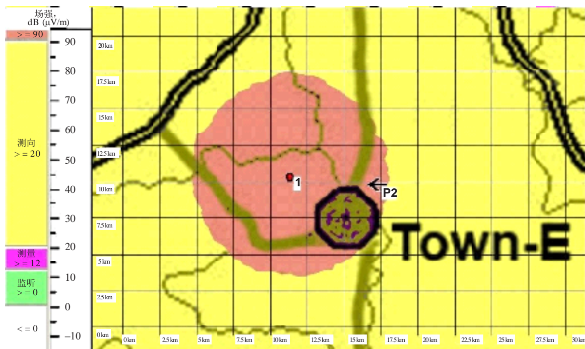
图17 站1的干扰保护区域
