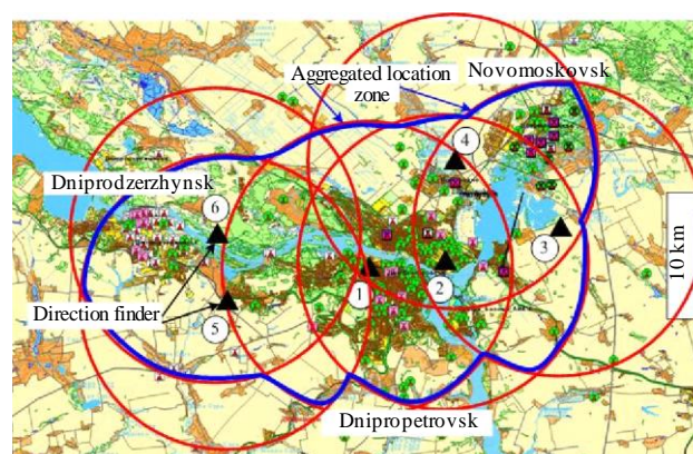
频谱监测网络的聚合定位面积
