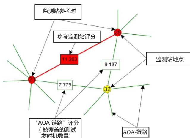
图23 “AOA-链路”部分示意图
