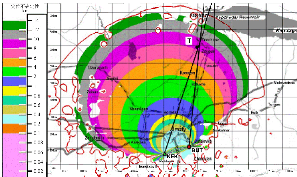
KEK站和BUT站适当选址的测向和定位覆盖范围
