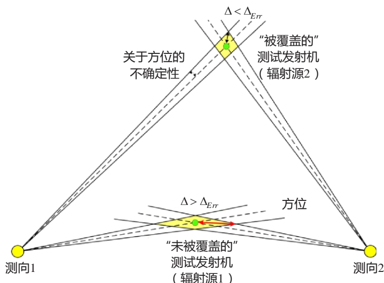
图22 通过两个AOA站确定覆盖区域示例
