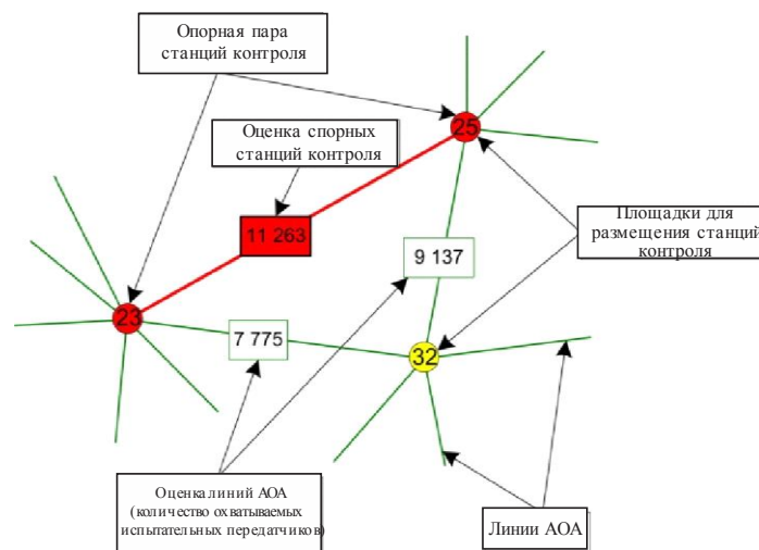
РИСУНОК 30 Часть схемы линий АОА
