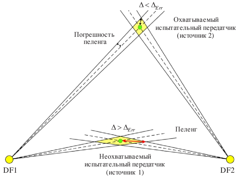
РИСУНОК 29 Пример определения зоны охвата двумя станциями АОА
