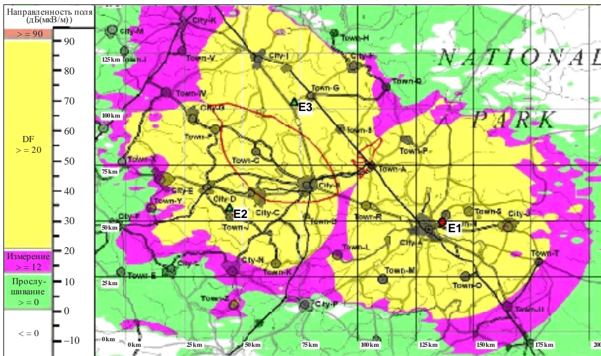
Общие зоны охвата трех действующих станций функциями контроля
