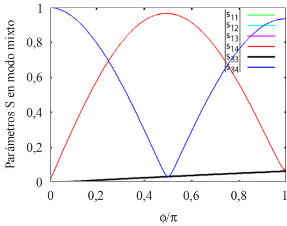
Modo par con pérdidas \phi_e = \phi_o = \phi , \alpha_e/\beta_e = 0,05
