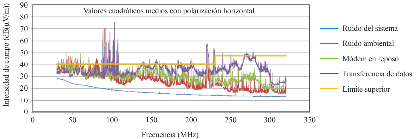
Valores cuadráticos medios (r.m.s.) de la intensidad de campo con polarización horizontal (dB(μV/m))
