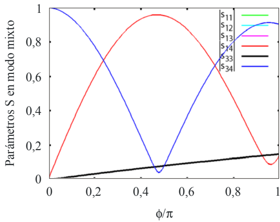
Modo dispersivo, modo par con pérdidas \phi_e = 1,1\phi_o = 1,1\phi , \alpha_e/\beta_e = 0,05
