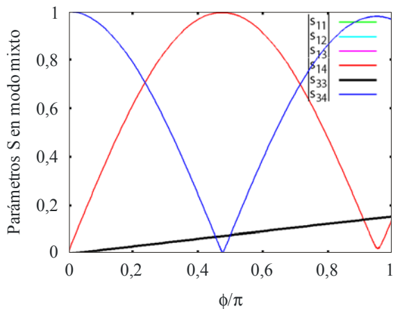
Modo dispersivo \phi_e = 1,1\phi_o = 1,1\phi
