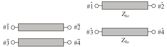
(a) Líneas acopladas (b) Modos par-impar
