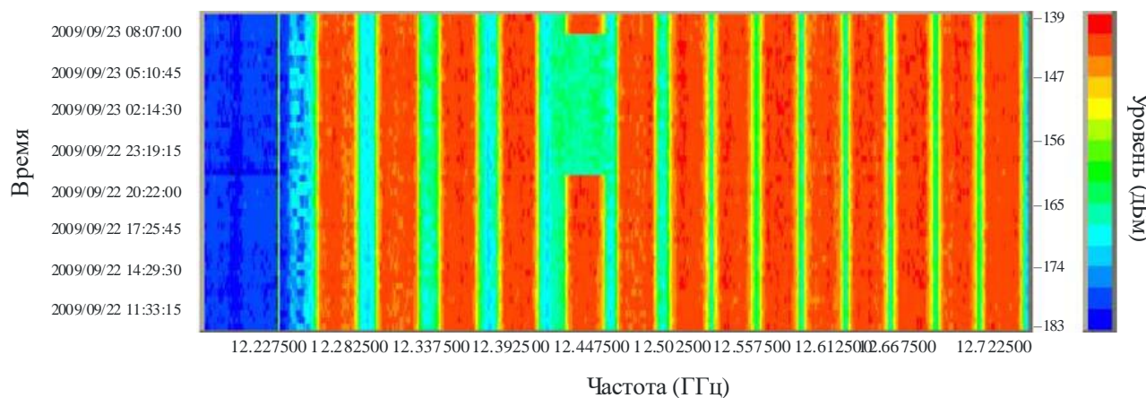
Пример выведенных на экран результатов анализа использования частот
