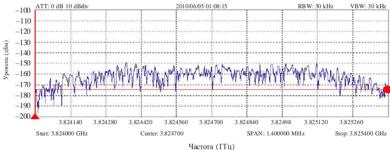
Пример выведенных на экран результатов анализа радиопараметров
