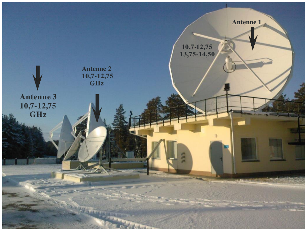
FIGURE 21 Vue d'ensemble des systèmes N° 1, 2 et 3
