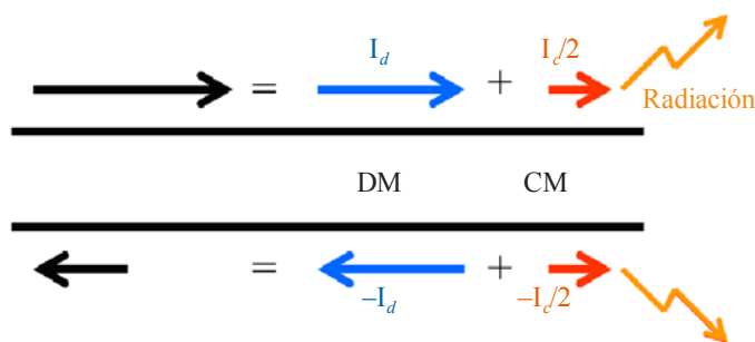
FIGURA 2-1 Corriente en modo diferencial y en modo común por una línea de transmisión de dos conductores
