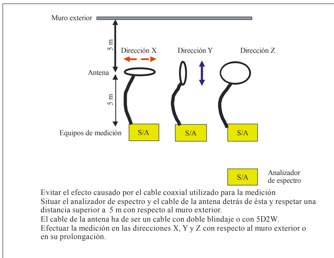
FIGURA A3-20 Posicionamiento del equipo de medición
