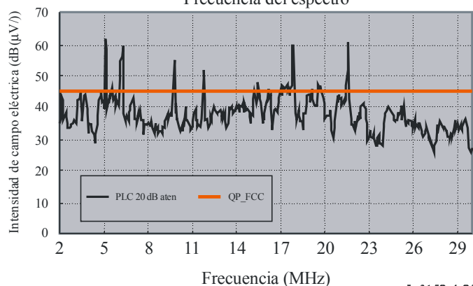
FIGURA 4-5 Medición a 10 m Frecuencia del espectro
