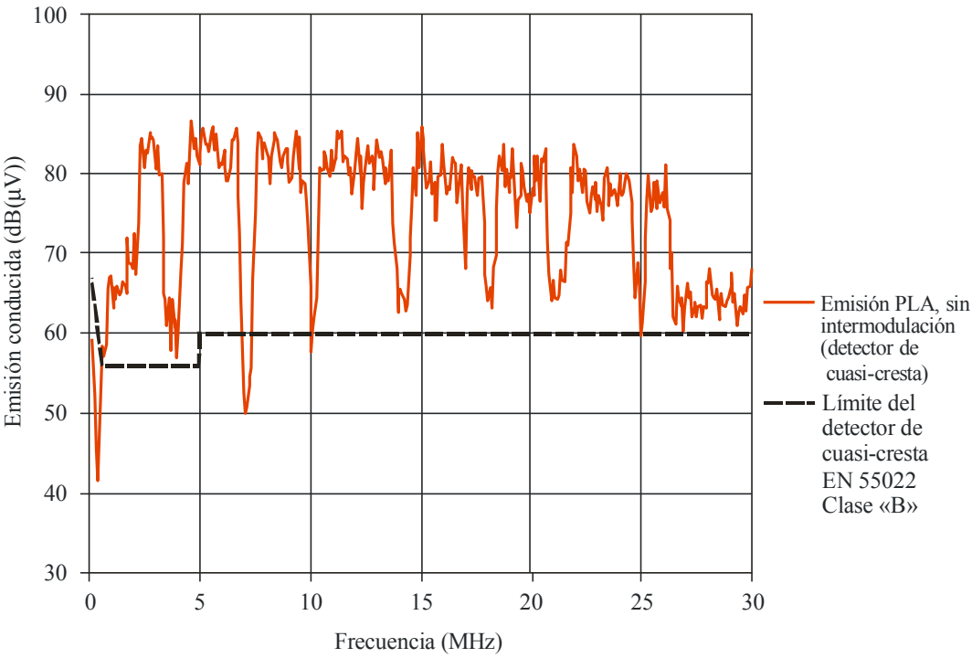
FIGURA 4-8 Efectos de la intermodulación en las ranuras
