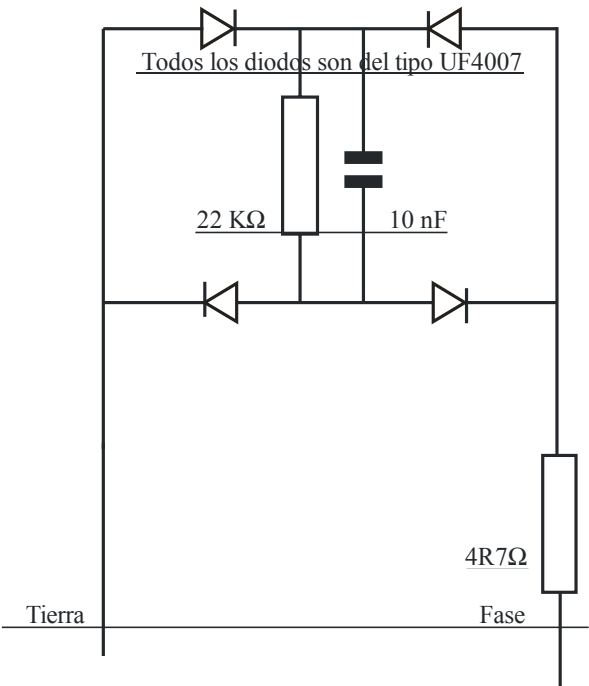
FIGURA 4-7 Pequeña fuente de alimentación simulada
