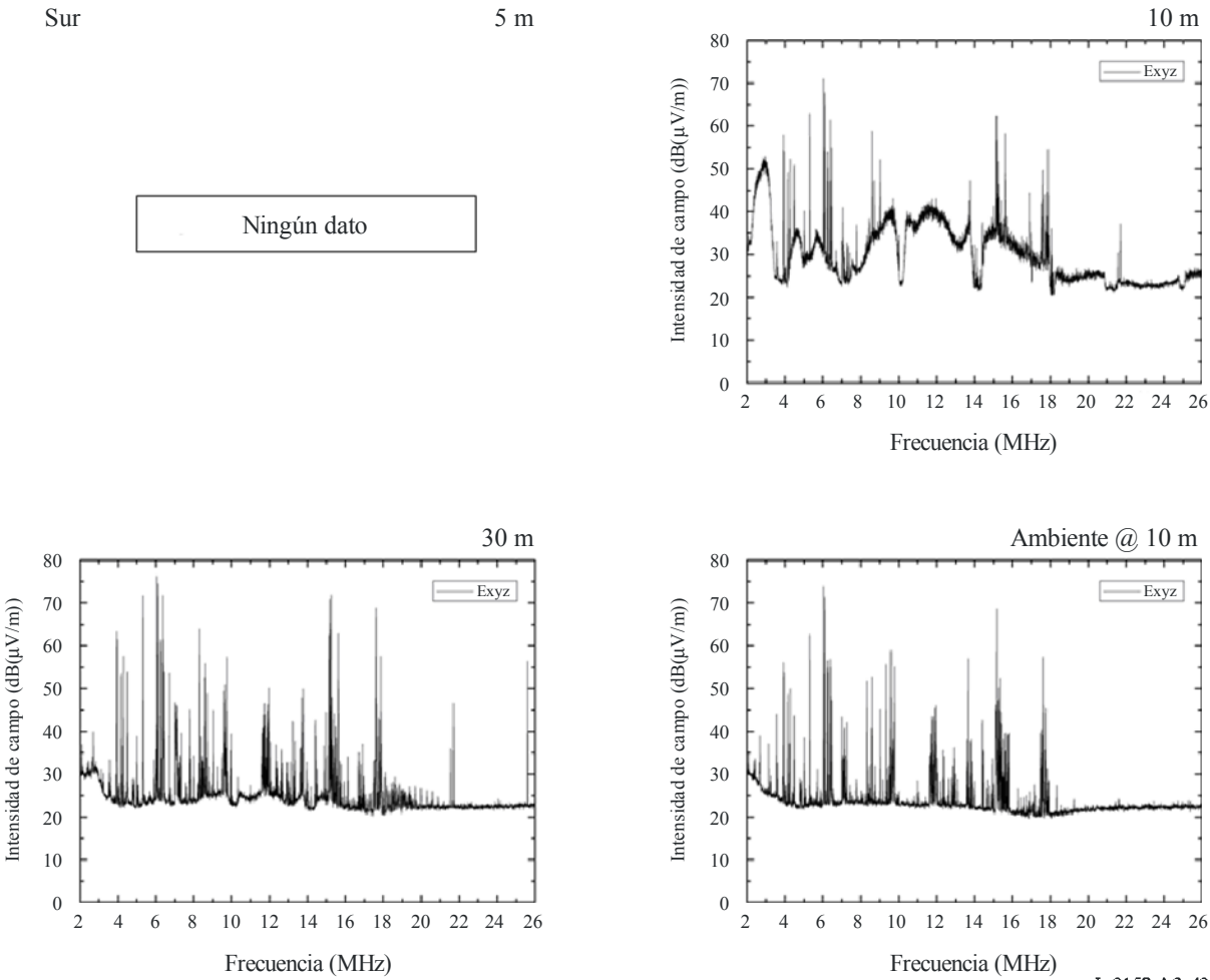
FIGURA A3-42 Intensidad de campo de fuga eléctrica (dB(μV/m)) del módem UPA hacia el Sur
