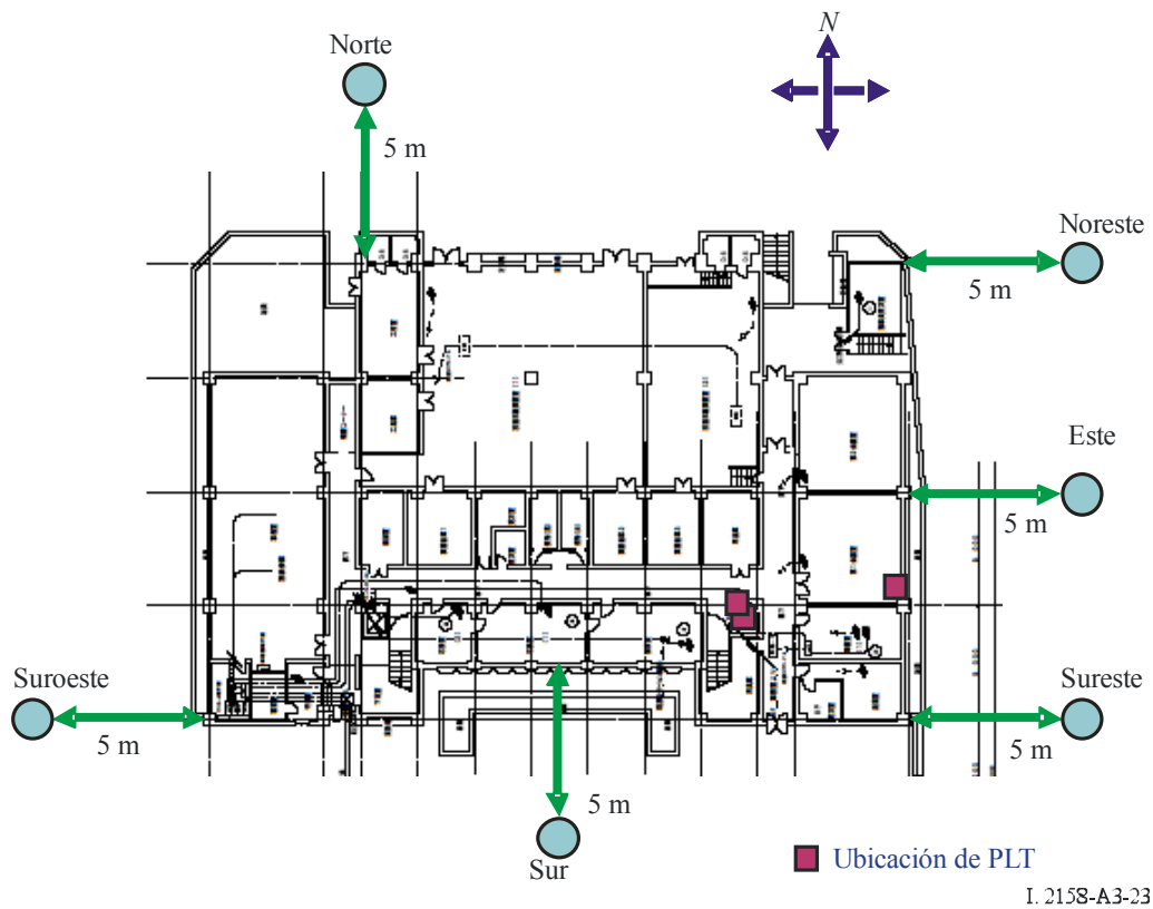
FIGURA A3-23 Condiciones de la medición (2)
