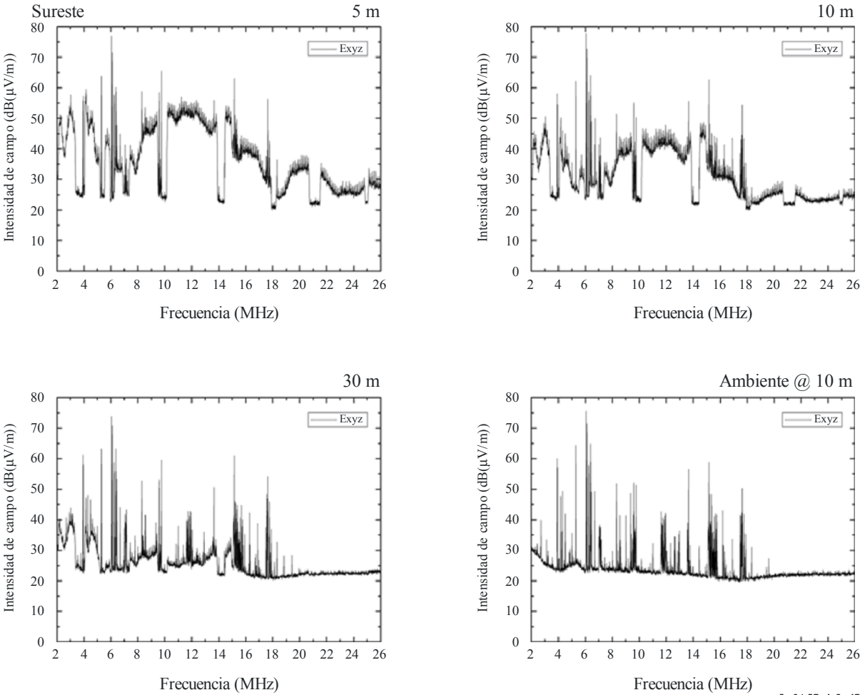
FIGURA A3-40 Intensidad de campo de fuga eléctrica (dB(μV/m)) del módem HDPLC hacia el Sureste
