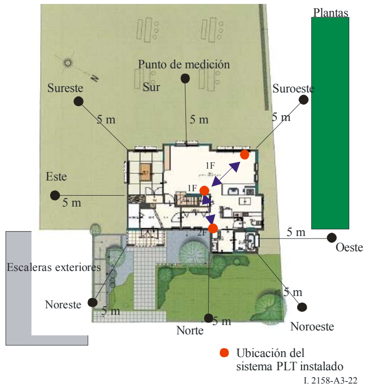
FIGURA A3-22 Condiciones de la medición (1)
