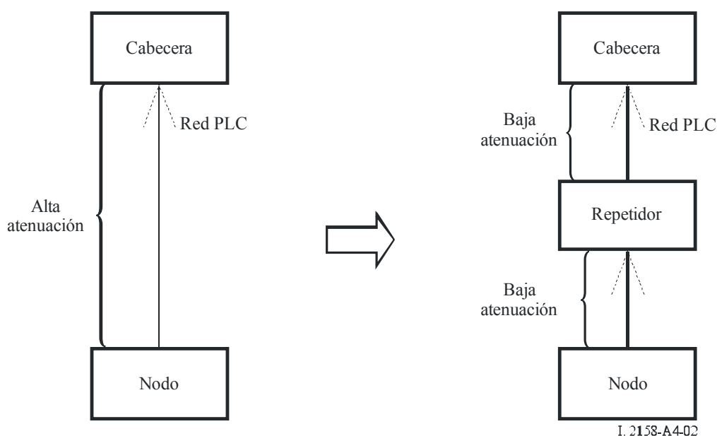
FIGURA A4-2 Utilización típica de un repetidor
