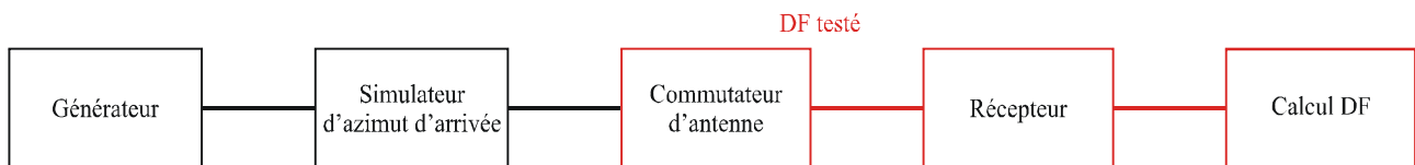
FIGURE 15 Dispositif de mesure de la précision DF pour une station de radiogoniométrie sur une plate-forme
