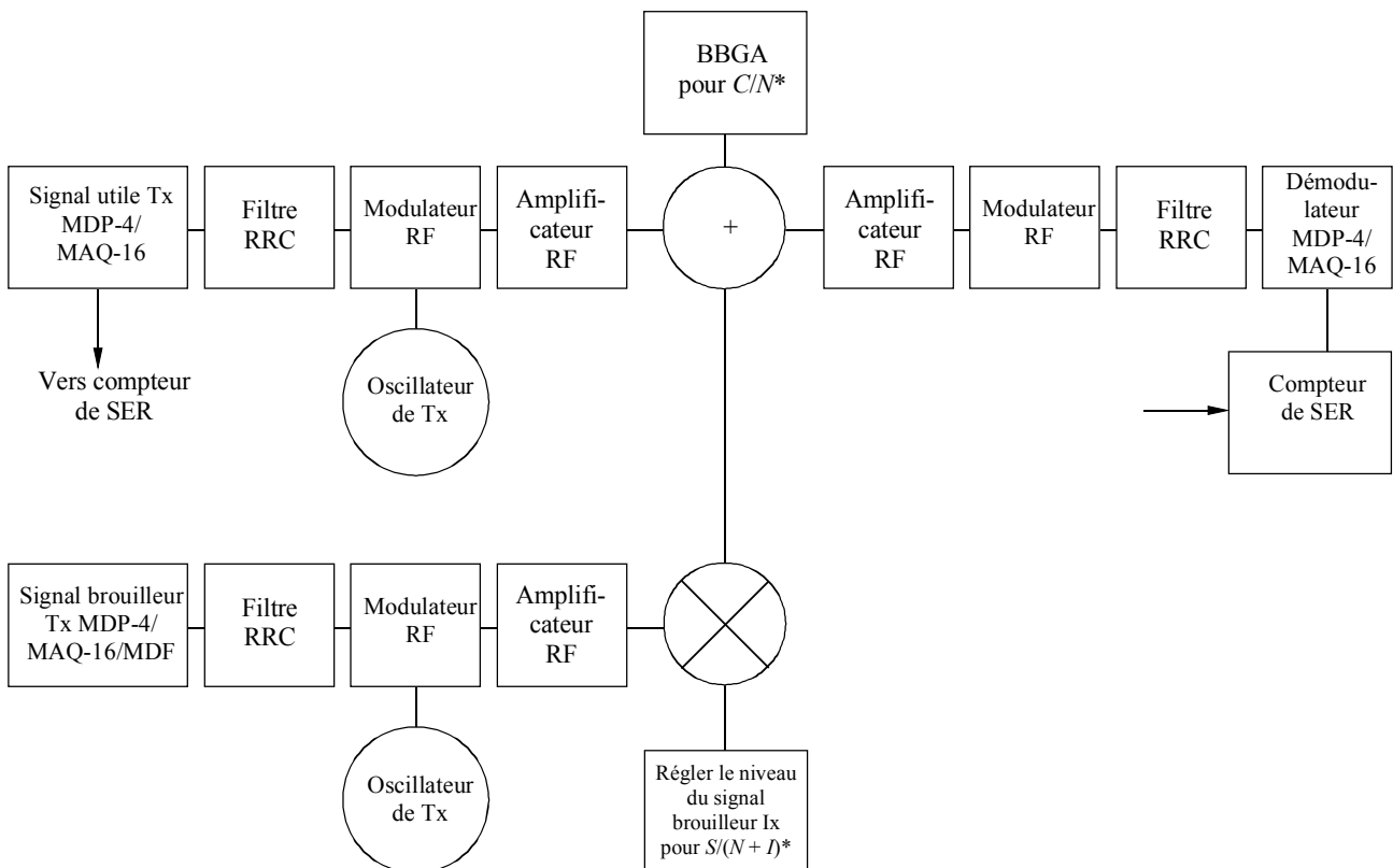
FIGURE 1 Configuration de simulation générique pour liaison fixe utile à modulation MDP-4 et MAQ-16 en présence de bruit et de brouillage
