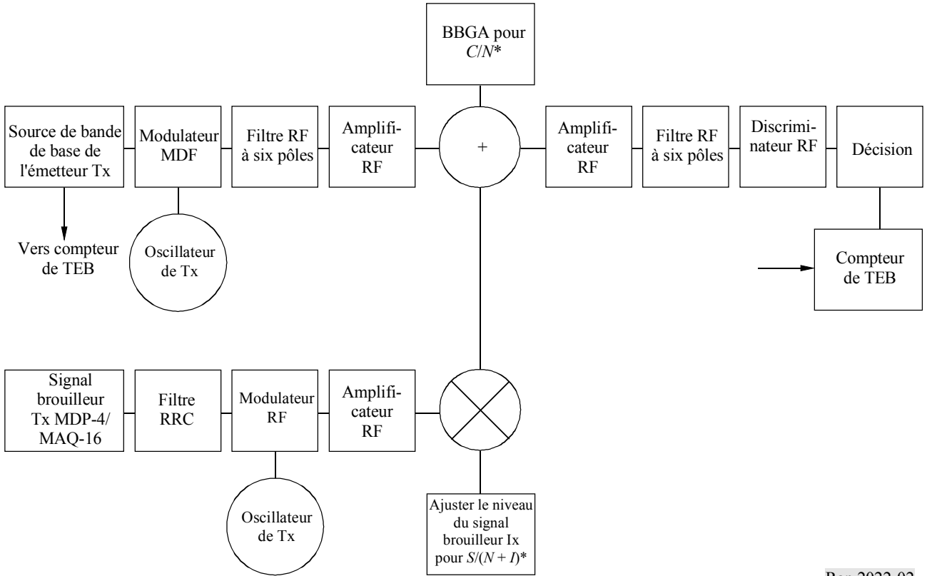
FIGURE 2 Configuration de simulation simplifiée pour liaison fixe utile à modulation MDF en présence de bruit et de brouillage
