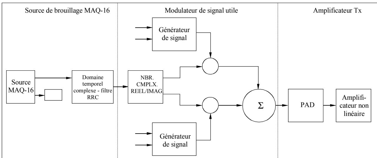
FIGURE 5 Emetteur MAQ-16
