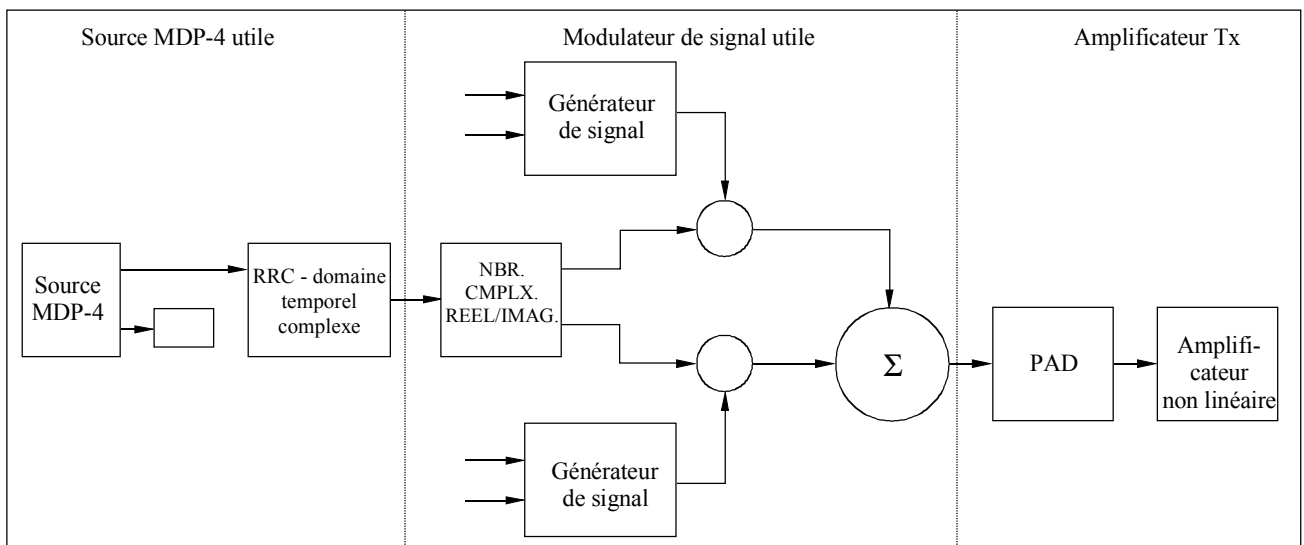
FIGURE 3 Emetteur MDP-4
