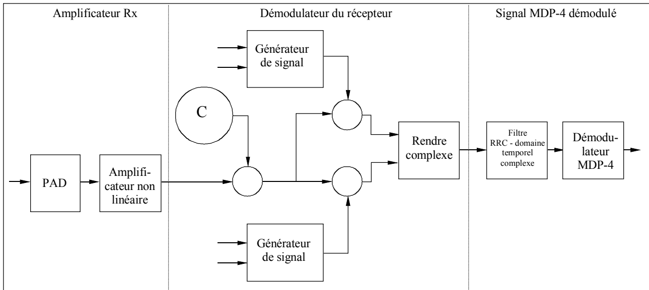
FIGURE 4 Récepteur MDP-4
