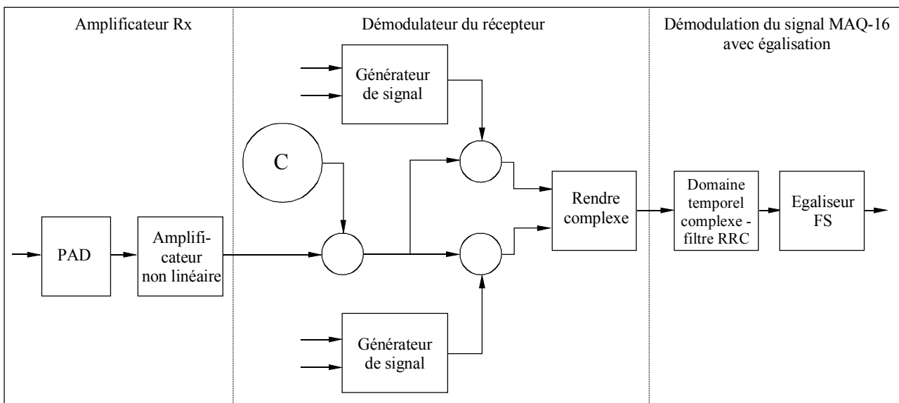
FIGURE 6 Récepteur MAQ-16
