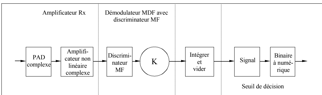
FIGURE 8 Récepteur MDF
