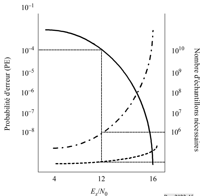
Comparaison du nombre d'échantillons entre la méthode Monte Carlo et la méthode IIS
