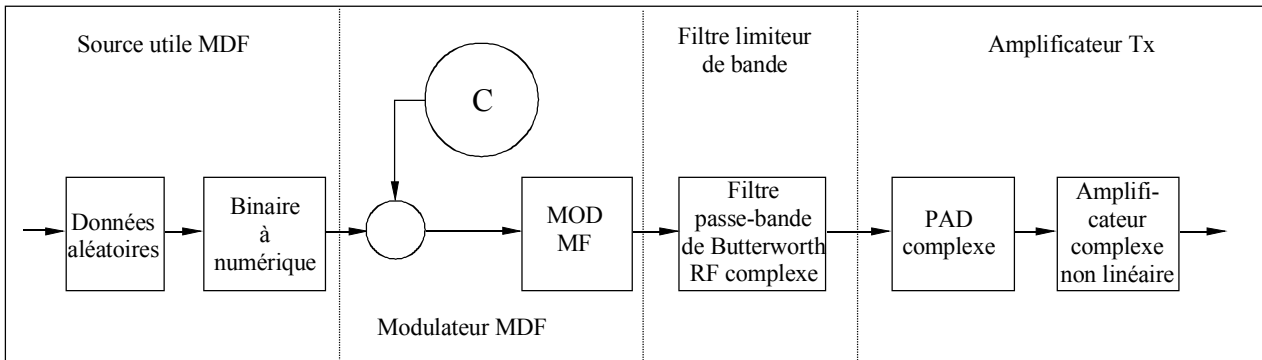
FIGURE 7 Emetteur MDF
